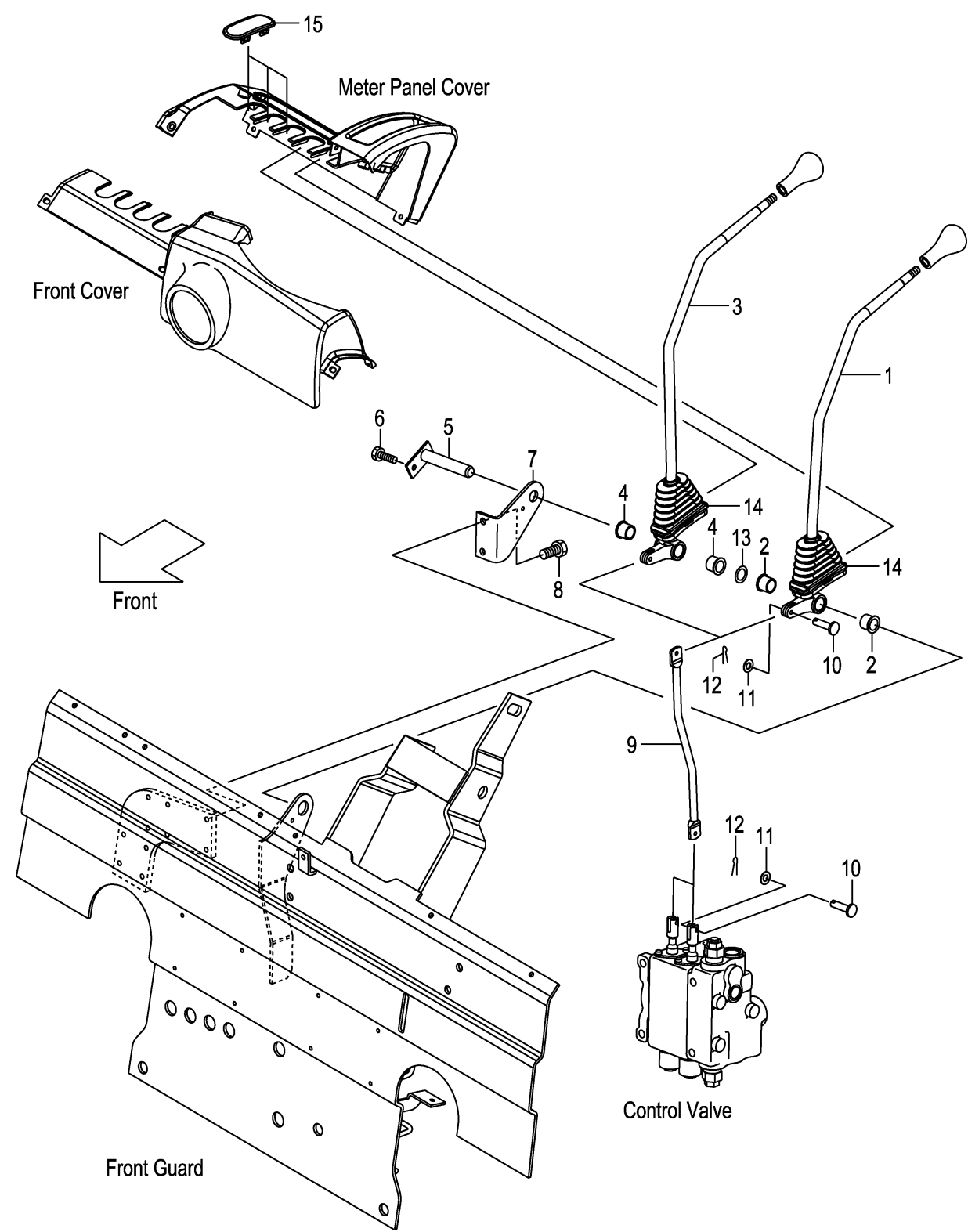
FIG.137 VALVE CONTROL [2SV] (F7Z373A0) バルブコントロール
