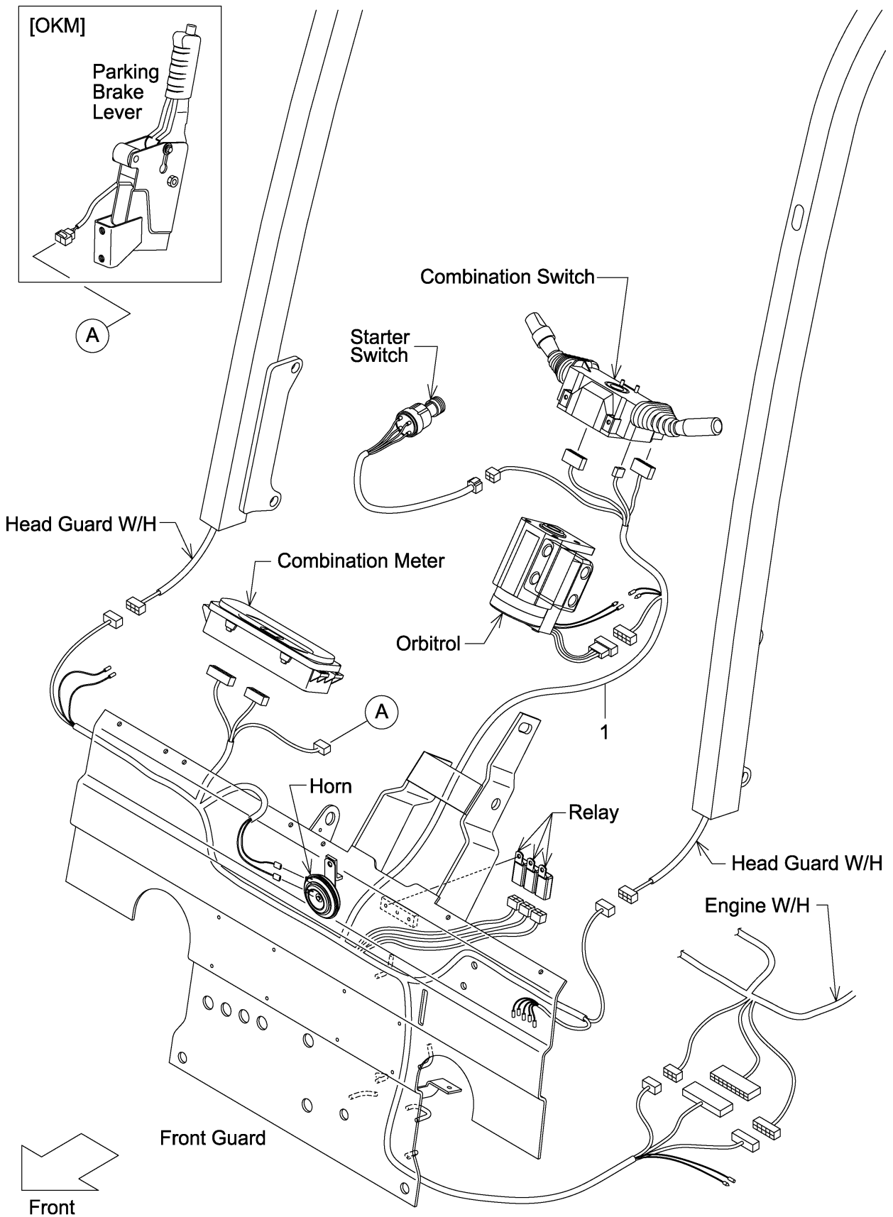
FIG.16 FRONT GUARD WIRE HARNESS (TOR-CON) (F7Z32430) フロントガードワイヤハーネス
