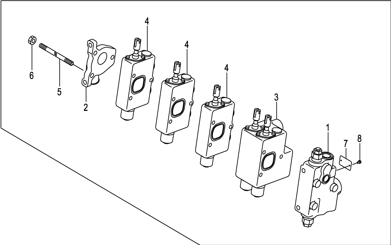
FIG.135 CONTROL VALVE [5SV] (F7Z37340) コントロールバルブ
