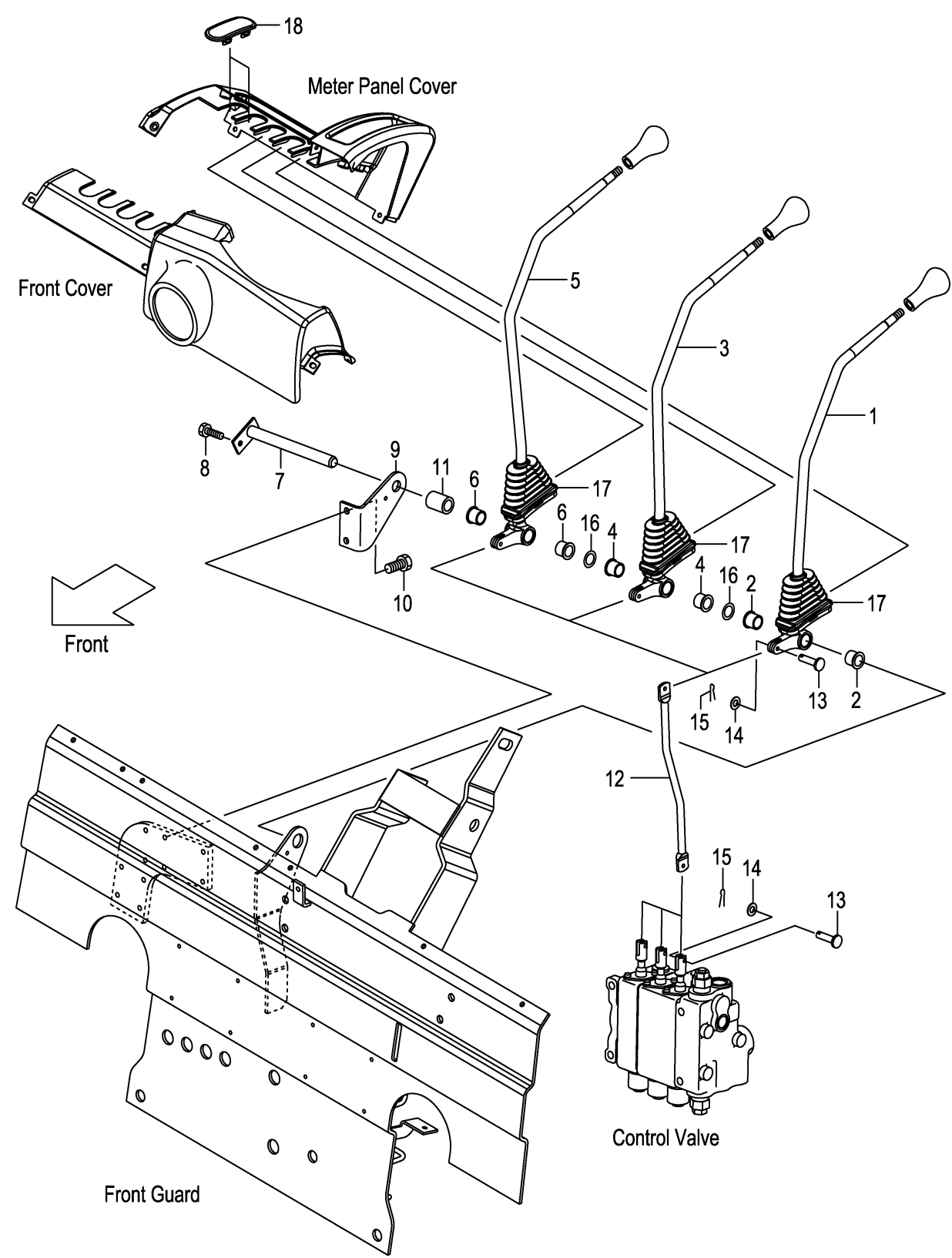
FIG.138 VALVE CONTROL [3SV] (F7Z373B0) バルブコントロール
