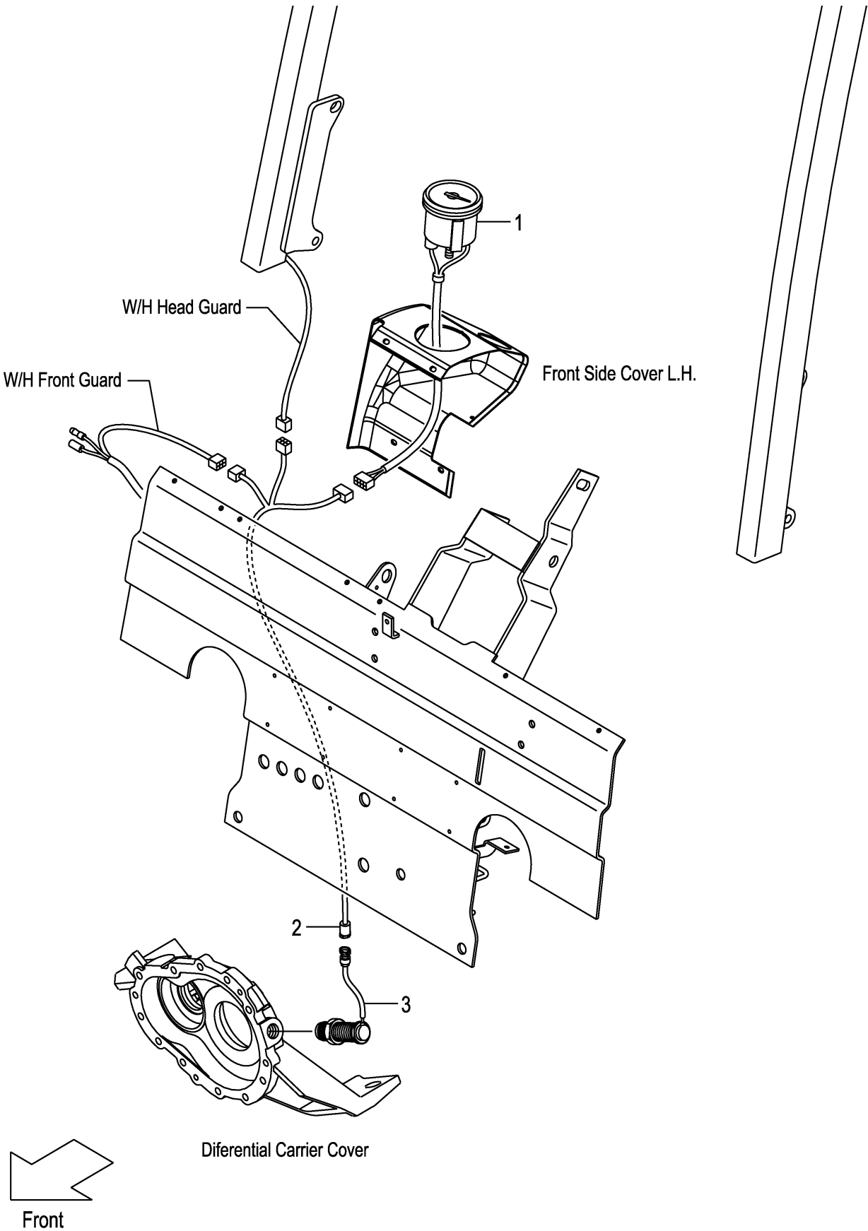
FIG.43 SPEED METER [SM] (F7Z326B0) スピードメータ
