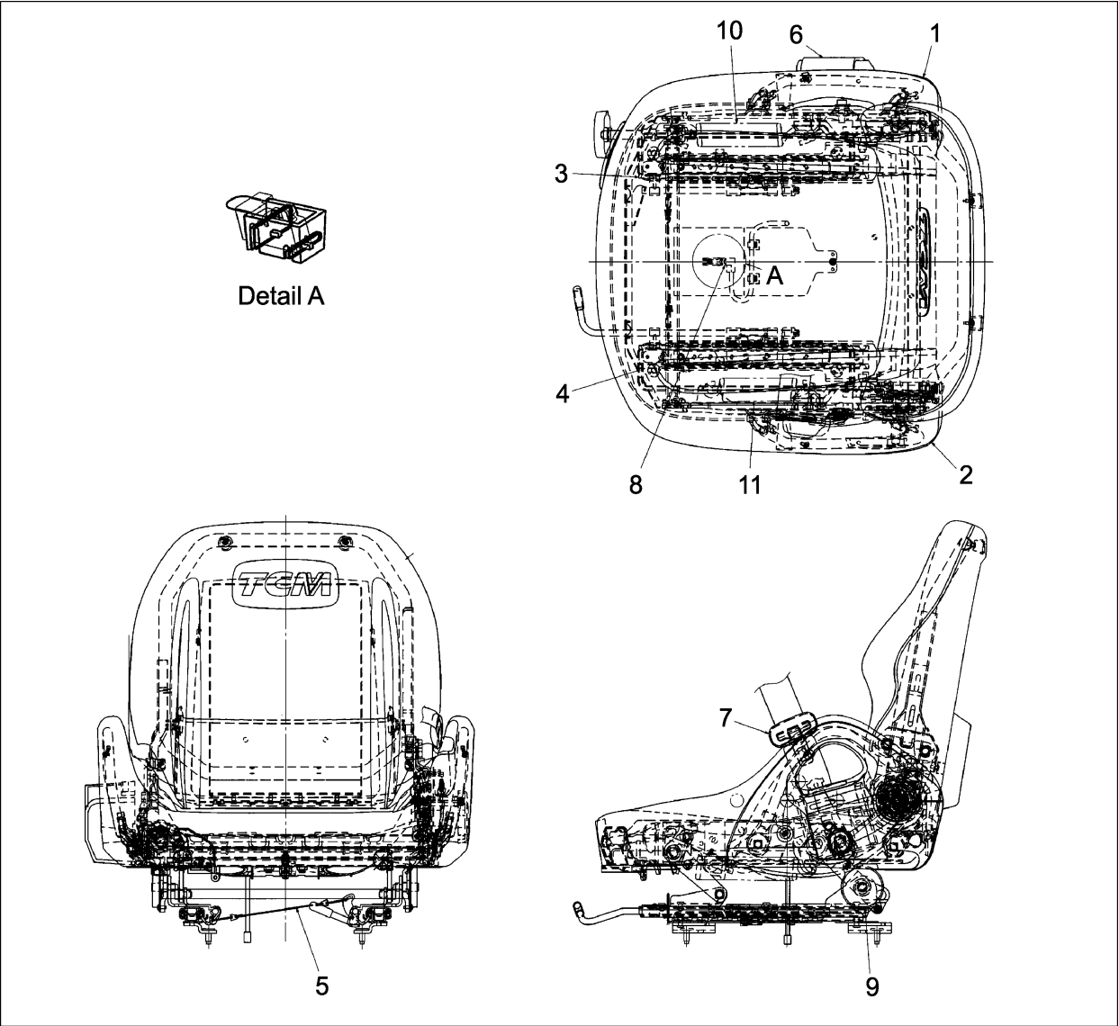
FIG.129 SEAT (F7Z36810) シート
