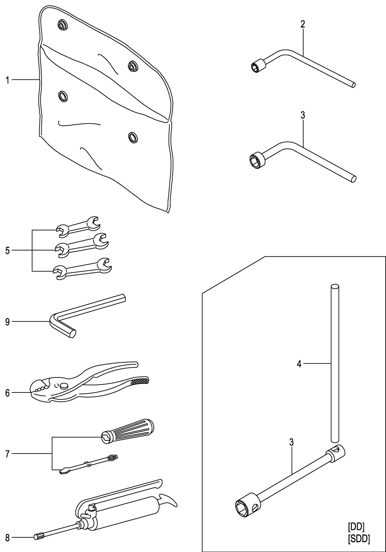
FIG.152 SERVICE TOOL (F7Z39210) サービスツール
