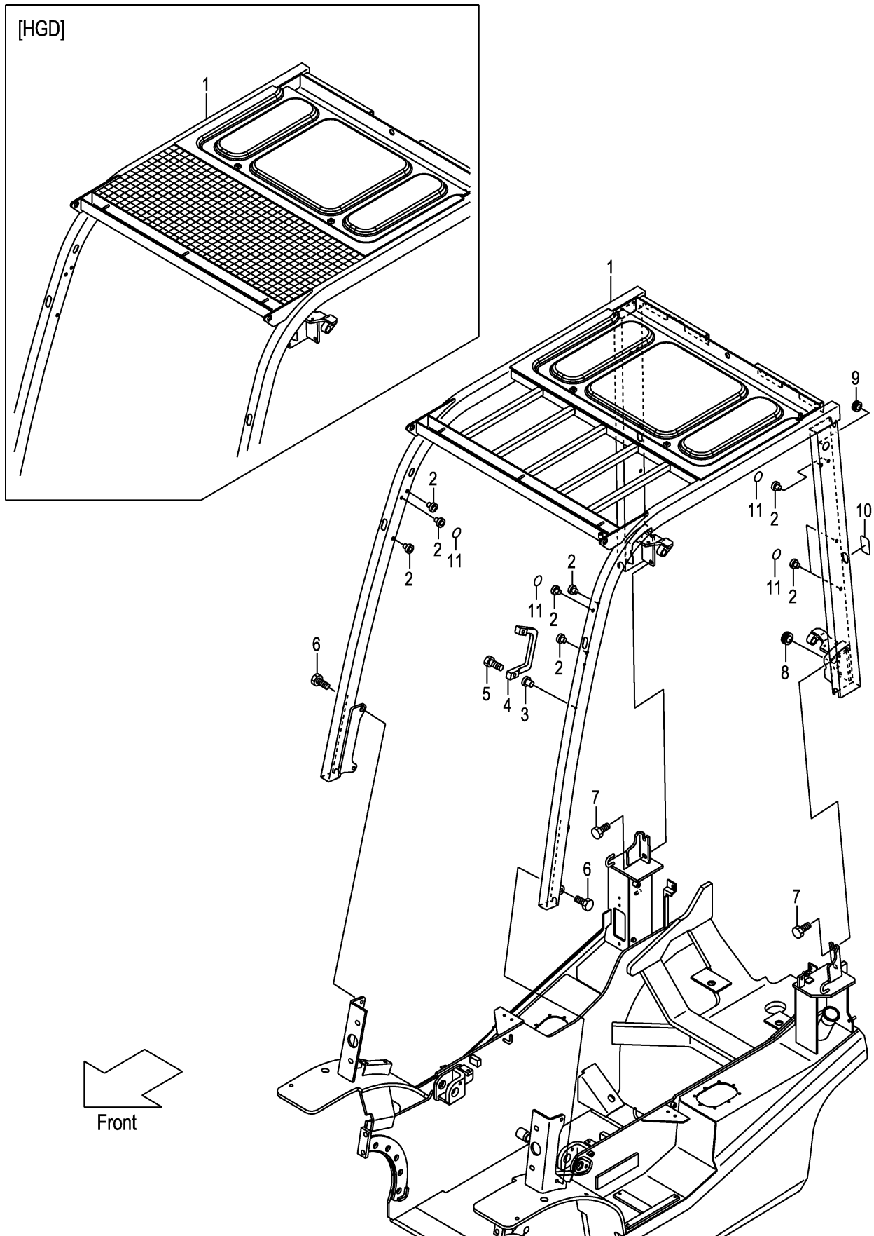
FIG.94 OVERHEAD GUARD (F7Z35110) オーバヘッドガード
