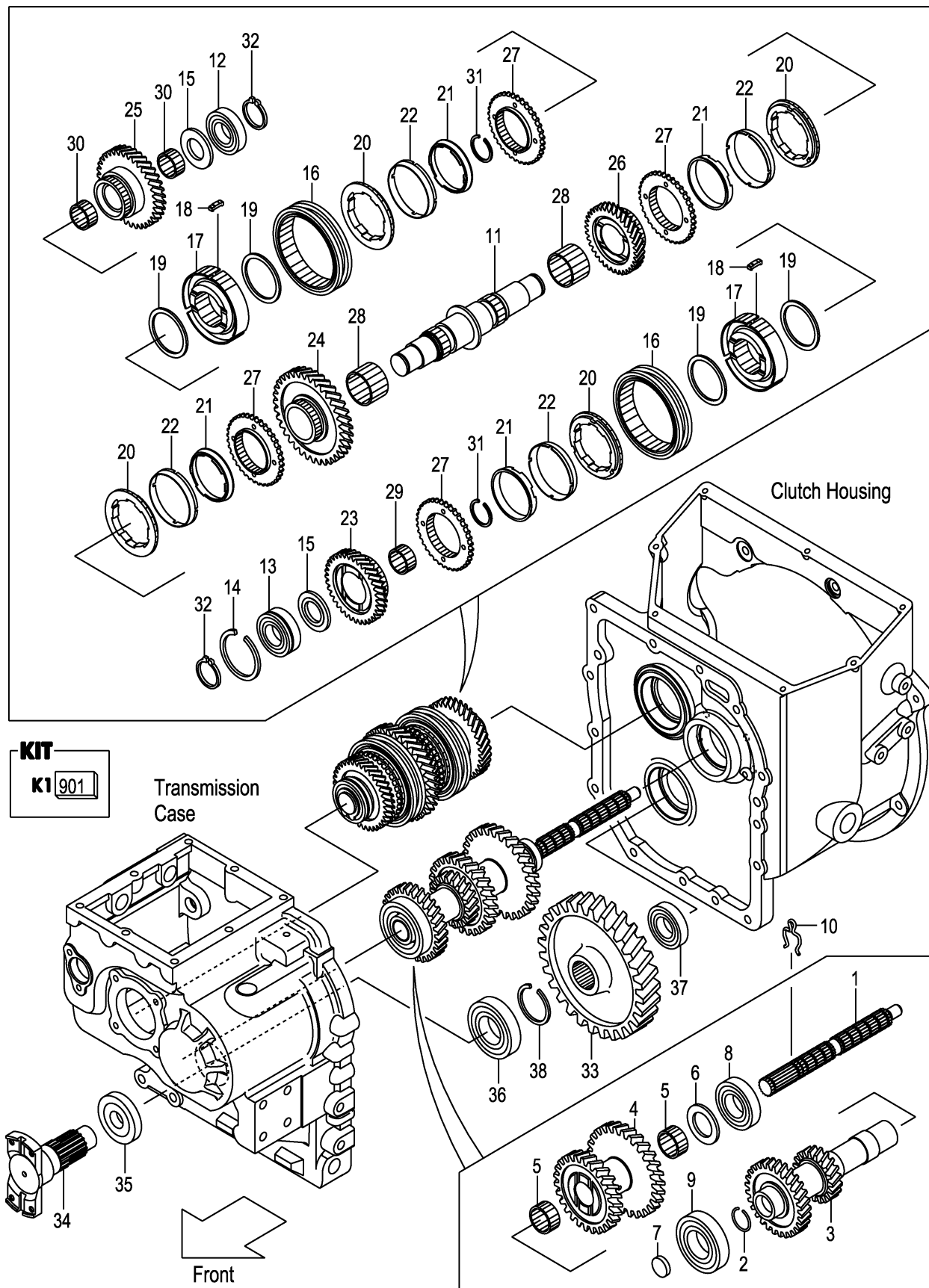
FIG.58 MISSION GEAR (CLUTCH) (F7Z32570) ミッションギヤー
