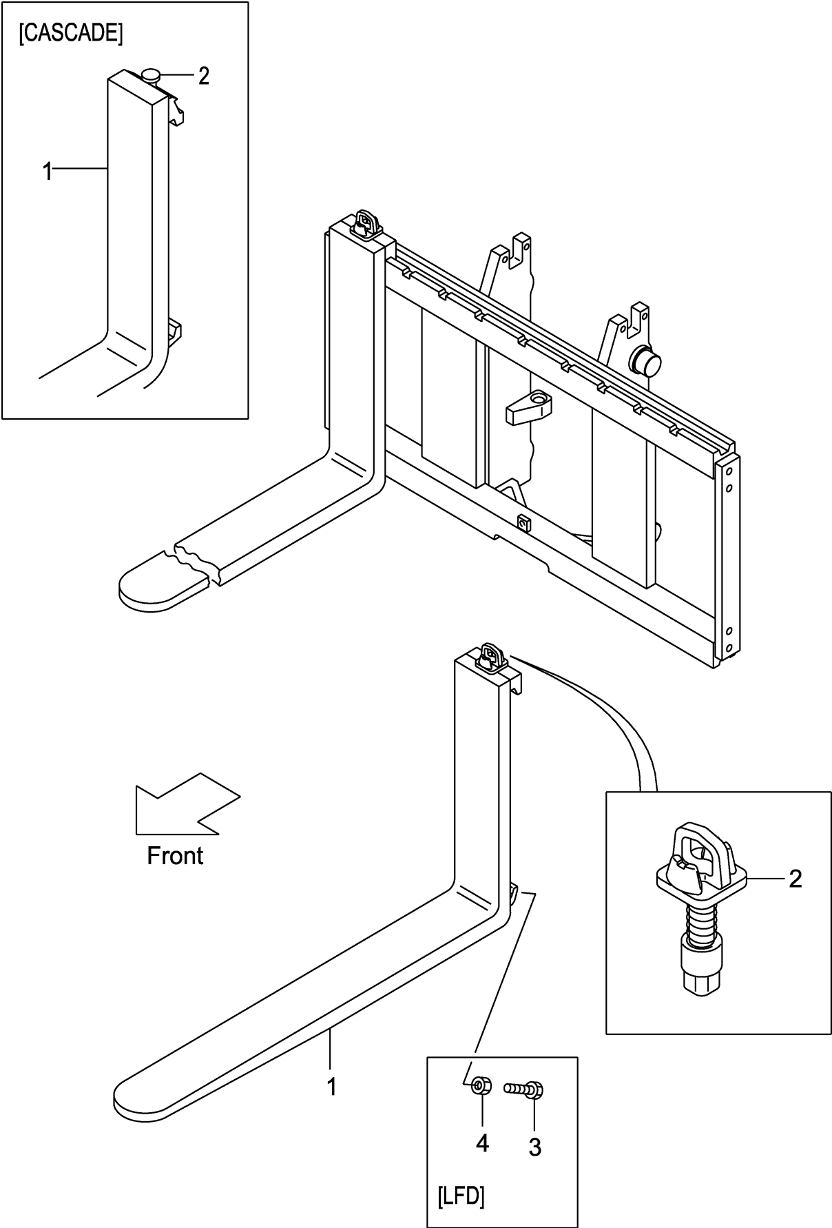
FIG.175 FORK [VFHM2N8] (M7028190) フォーク
