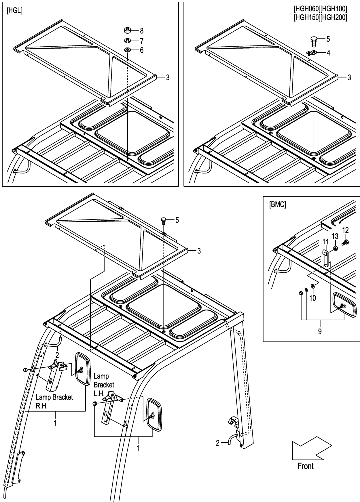
FIG.99 HEAD GUARD PARTS (F7Z351A0) ヘッドガードパーツ
