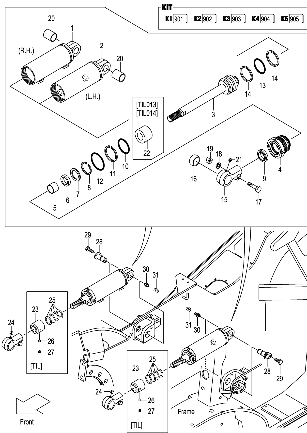
FIG.147 TILT CYLINDER (F7Z38510) ティルトシリンダ
