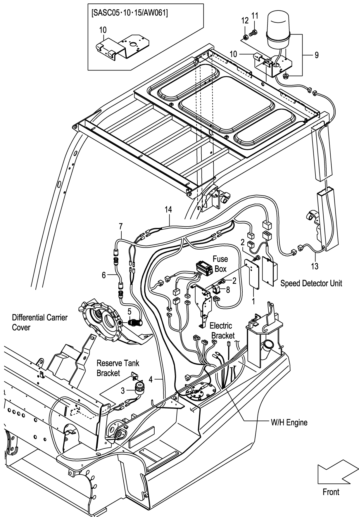
FIG.49 SPEED ALARM SYSTEM [SASC] (F7Z326H0) スピード・アラームシステム
