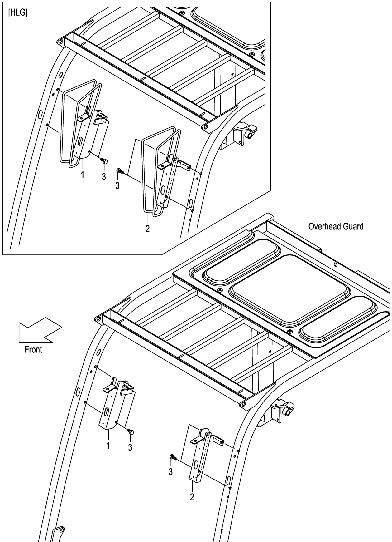
FIG.95 FRONT LAMP BRACKET (F7Z35120) フロントランプブラケット
