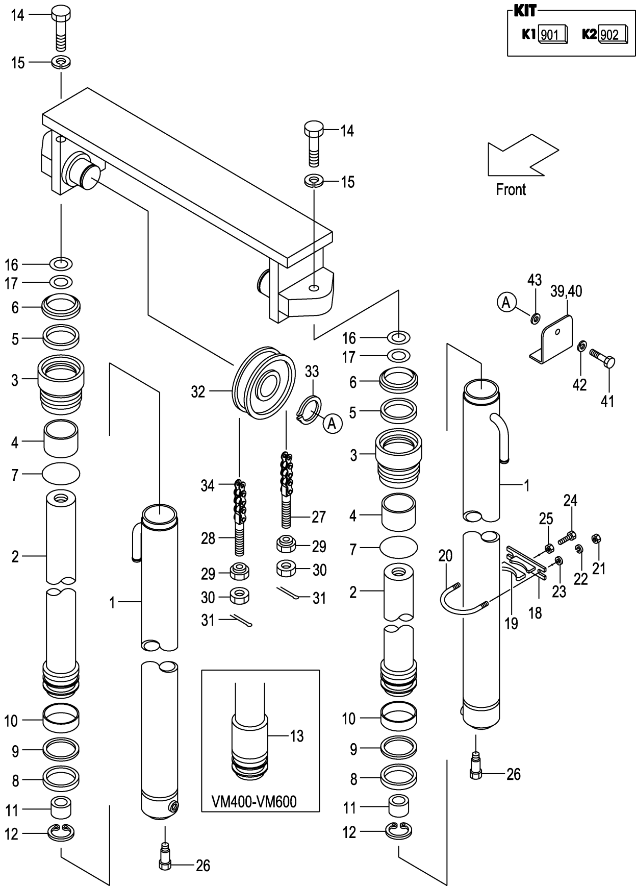
FIG.157 LIFT CYLINDER [VM2N9] (M7028430) リフトシリンダ
