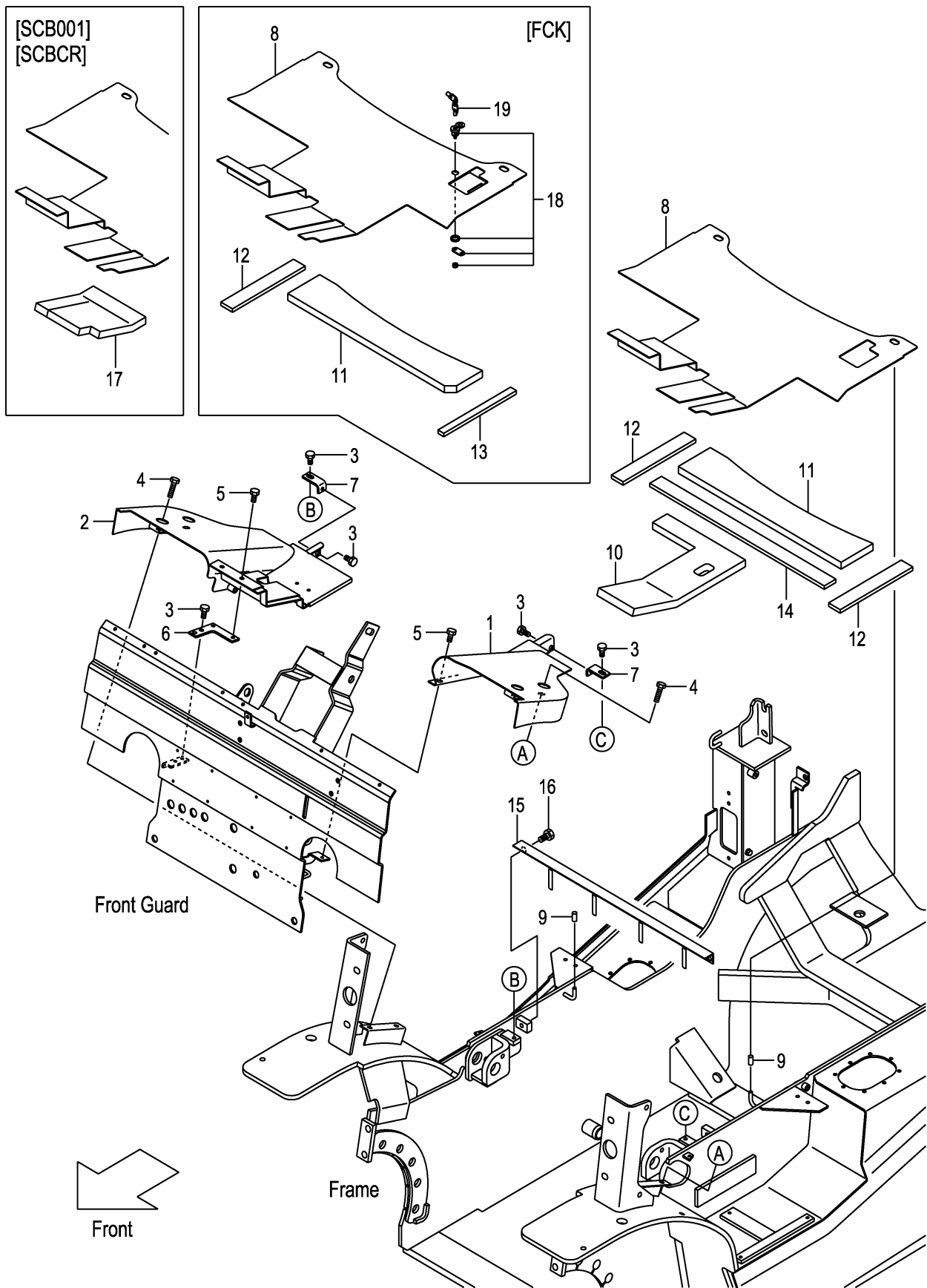
FIG.122 FLOOR BOARD (F7Z36450) フロアボード
