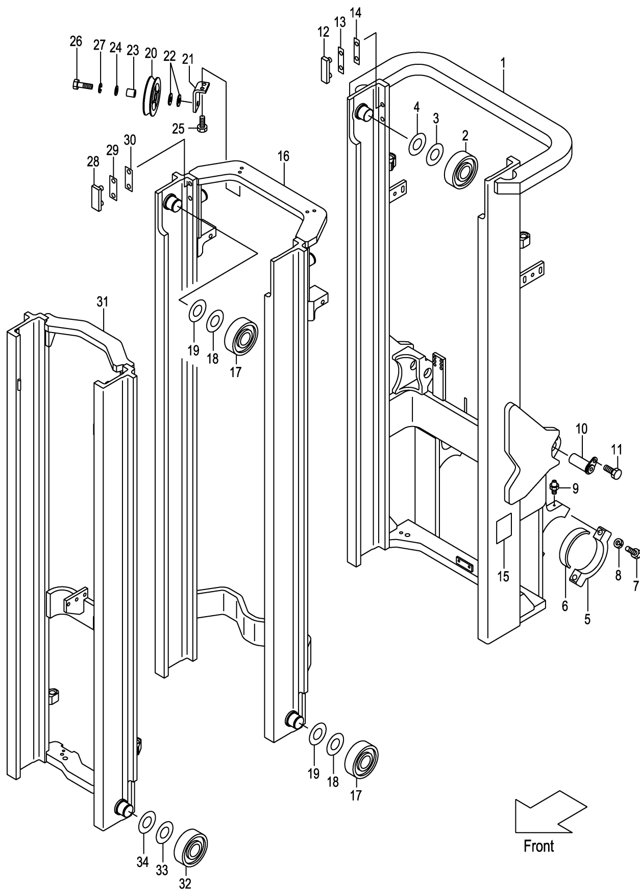
FIG.178 MAST [VFHM2N8] (M7020760) マスト
