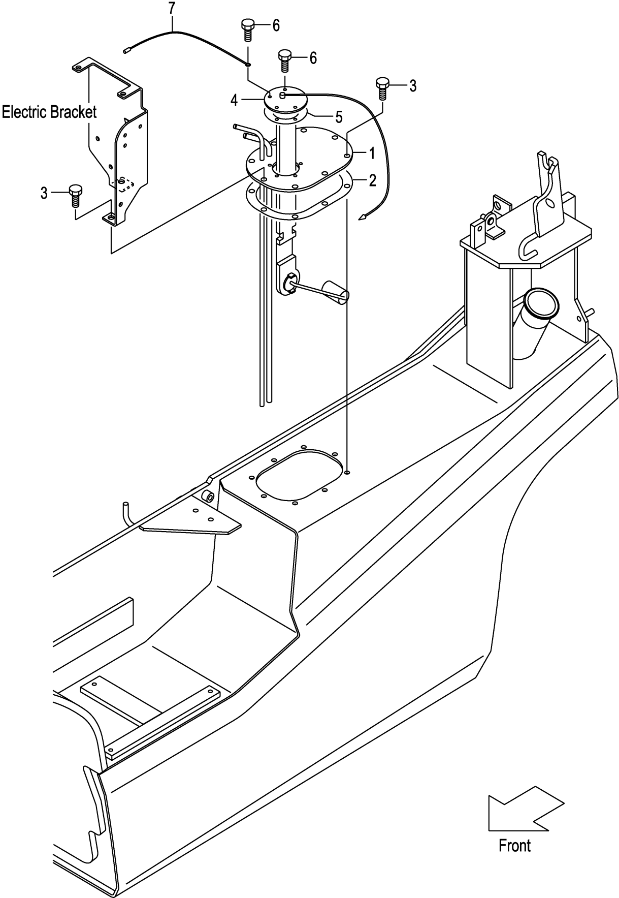
FIG.115 FUEL TANK (F7Z36150) フューエルタンク
