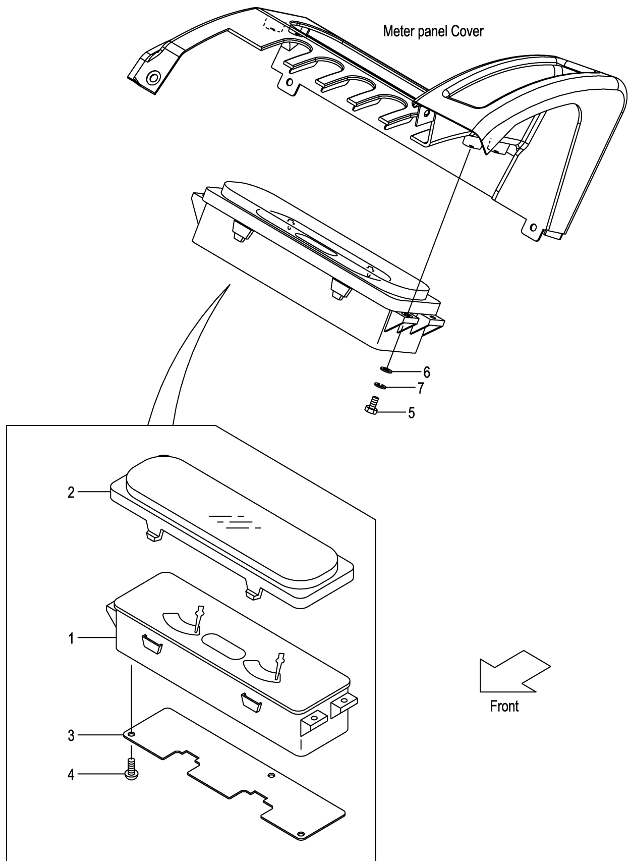
FIG.14 COMBINATION METER (F7Z32410) コンビネーションメータ
