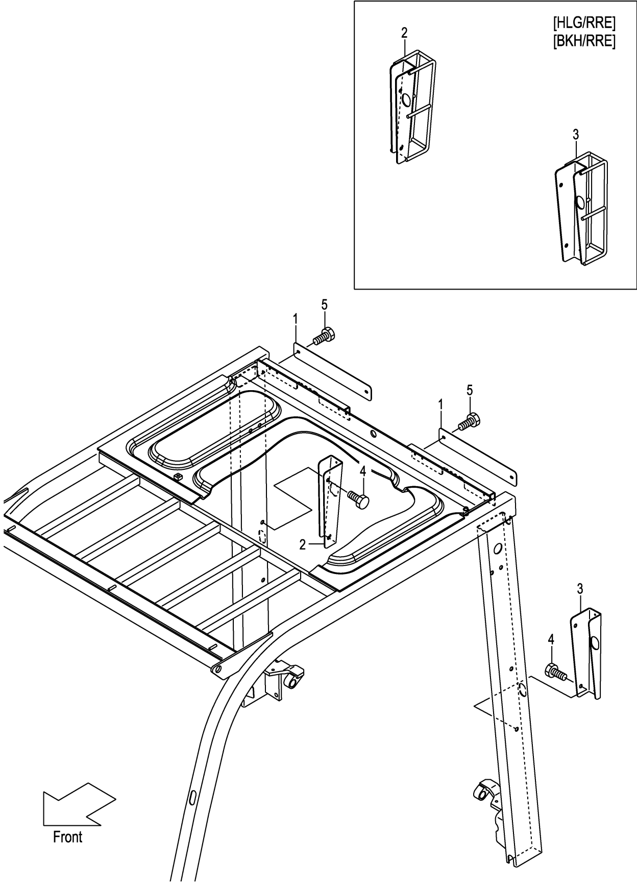
FIG.98 REAR LAMP COVER [RRE] (F7Z35150) リヤーランプカバー
