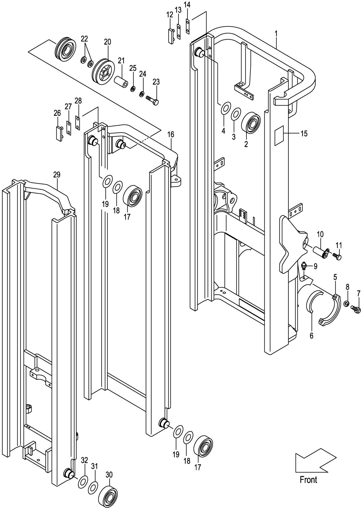
FIG.170 MAST [VFHM2N9] (M7020740) マスト
