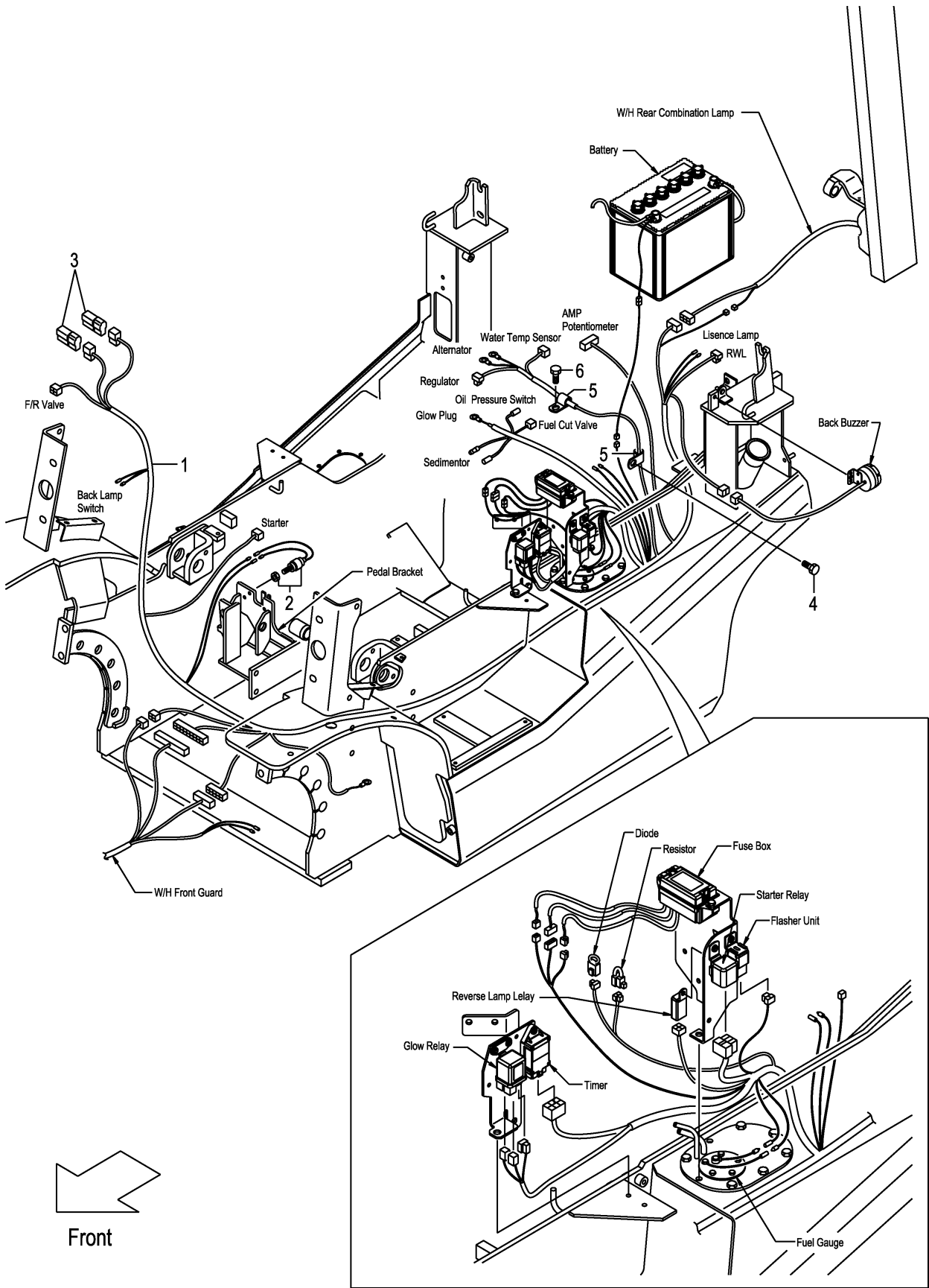
FIG.22 ENGINE WIRE HARNESS (TOR-CON) (F7Z324D0) エンジンワイヤハーネス
