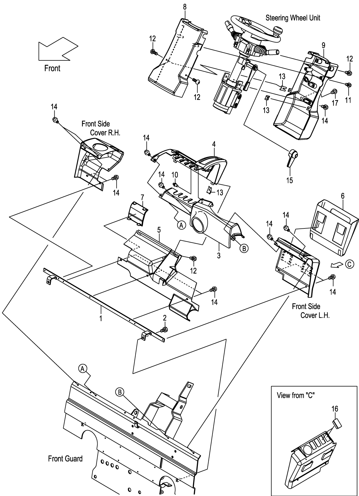
FIG.125 FRONT COVER (TOR-CON) (F7Z36480) フロントカバー
