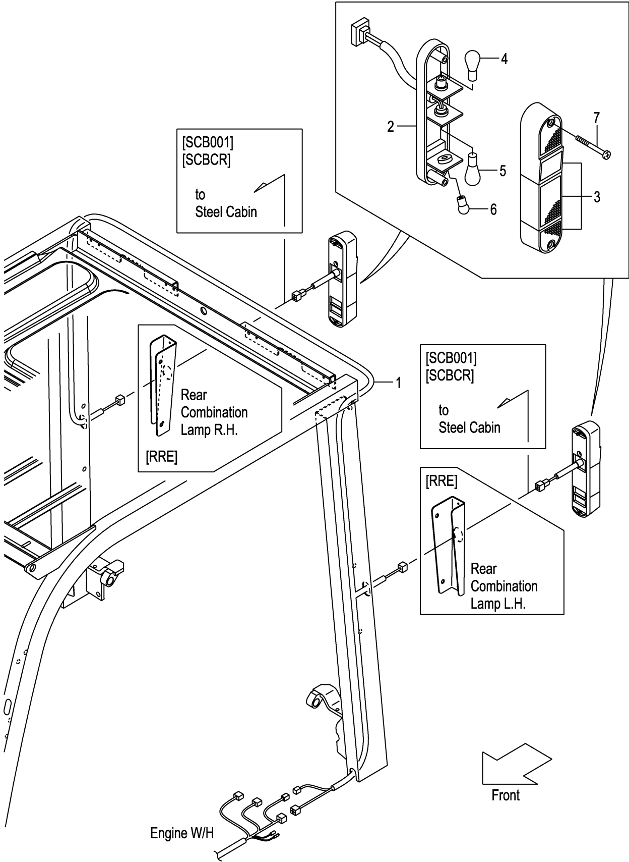
FIG.26 REAR COMBINATION LAMP [RRE][SCB001][SCBCR] (F7Z324J0) リヤコンビネーションランプ
