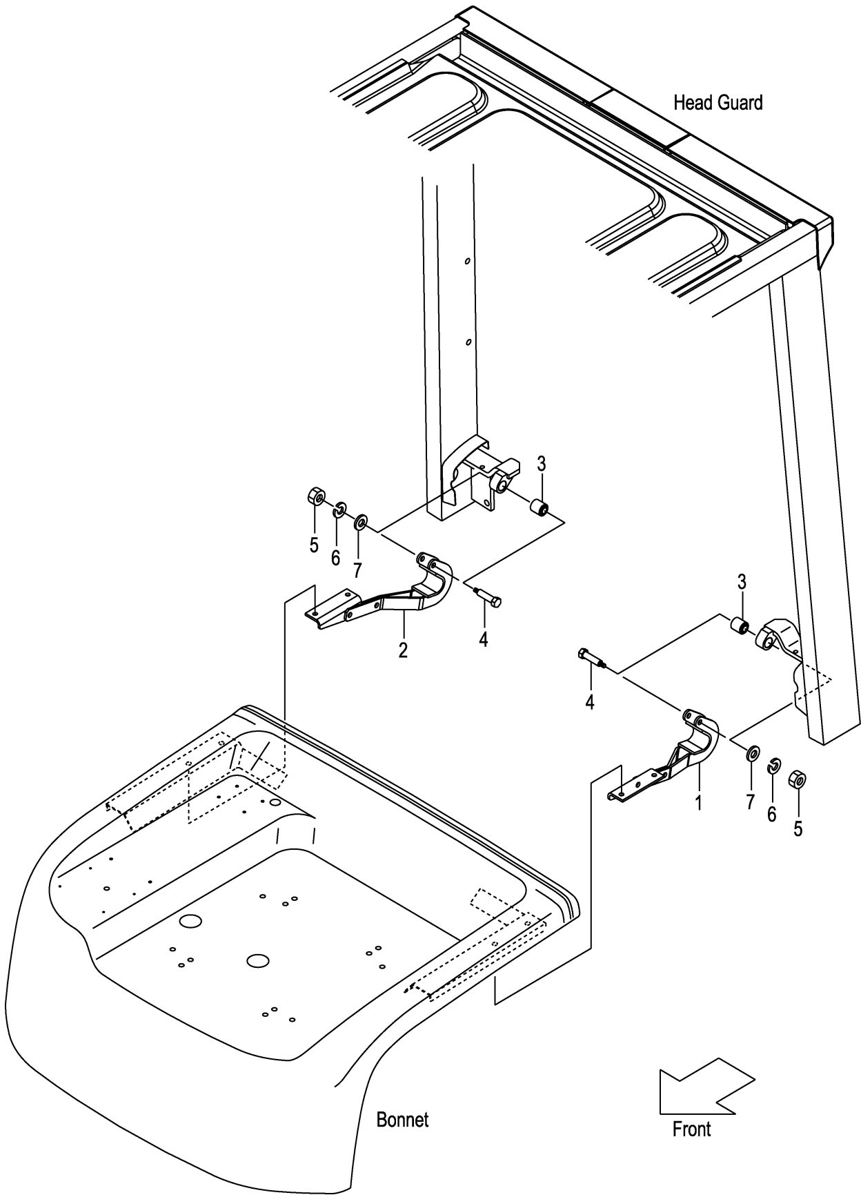
FIG.121 BONNET HINGE (F7Z36440) ホンネットヒンジ
