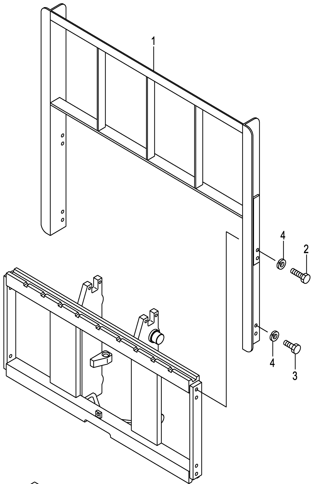
FIG.177 BACKREST [VFHM2N8] (M70282A0) バックレスト
