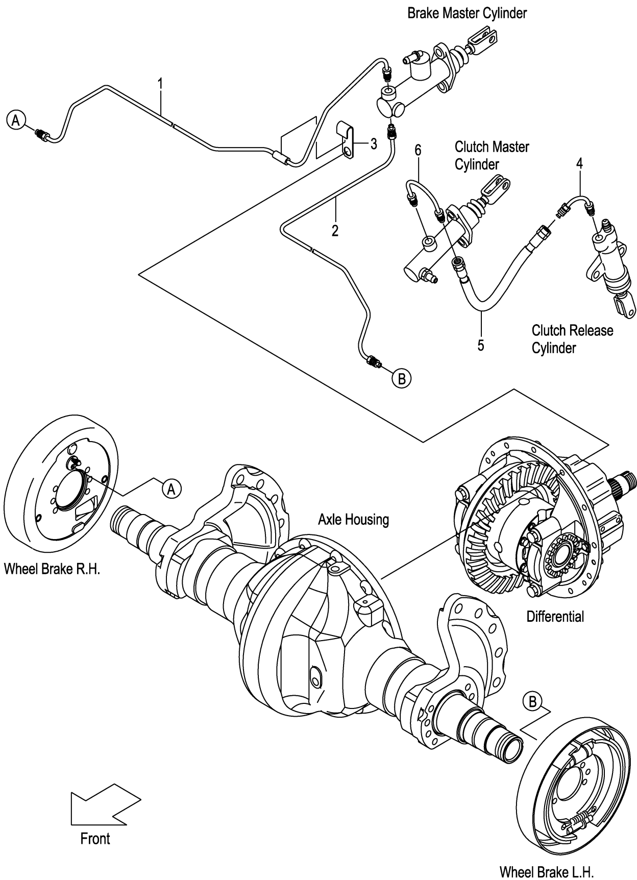
FIG.105 BRAKE PIPE (CLUTCH) (F7Z35490) ブレーキパイプ
