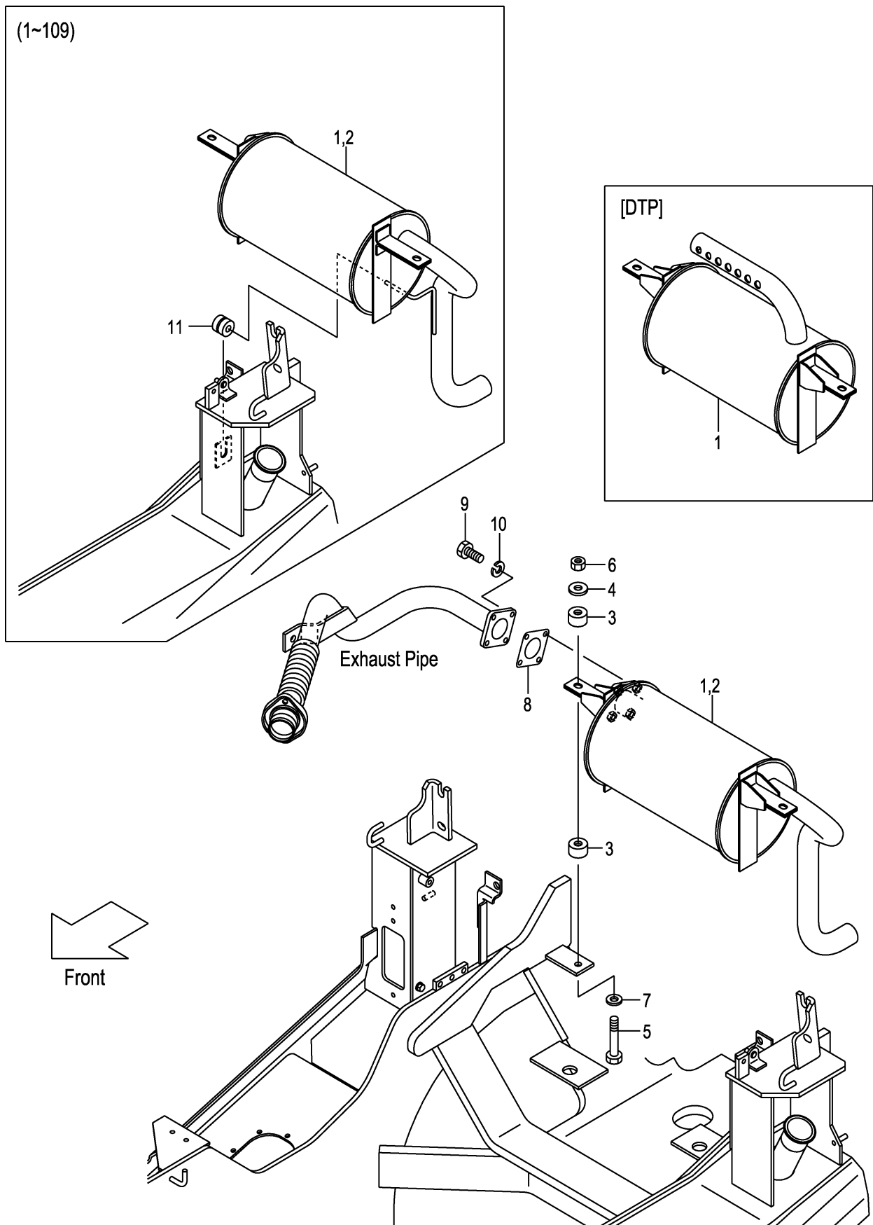
FIG.11 EXHAUST SYSTEM (F7Z32310) エキゾーストシステム
