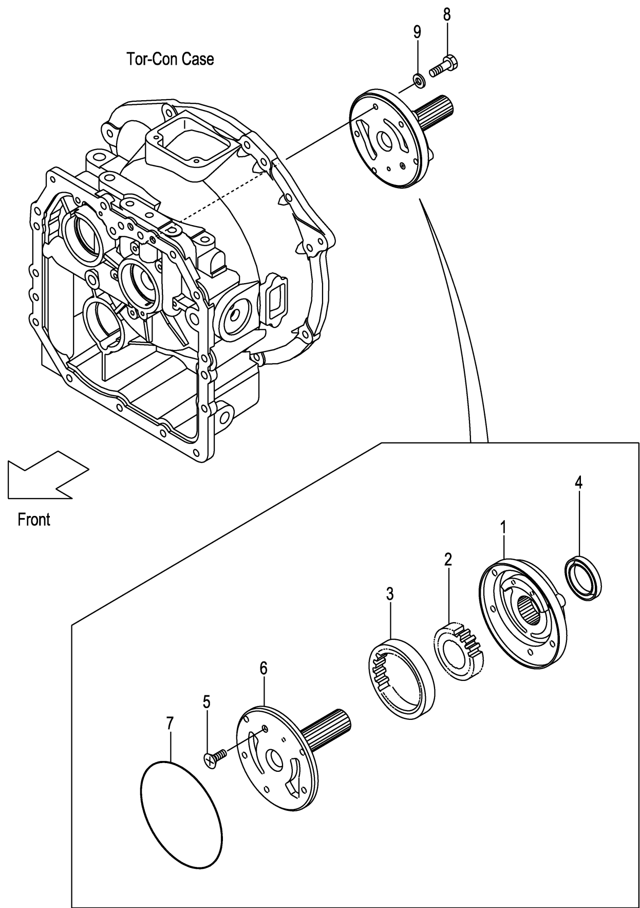
FIG.60 CHARGING PUMP (TOR-CON) (F7Z32590) チャージングポンプ°
