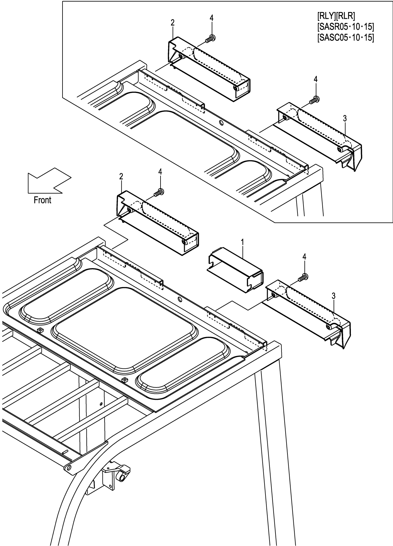
FIG.97 REAR LAMP COVER (F7Z35140) リヤーランプカバー
