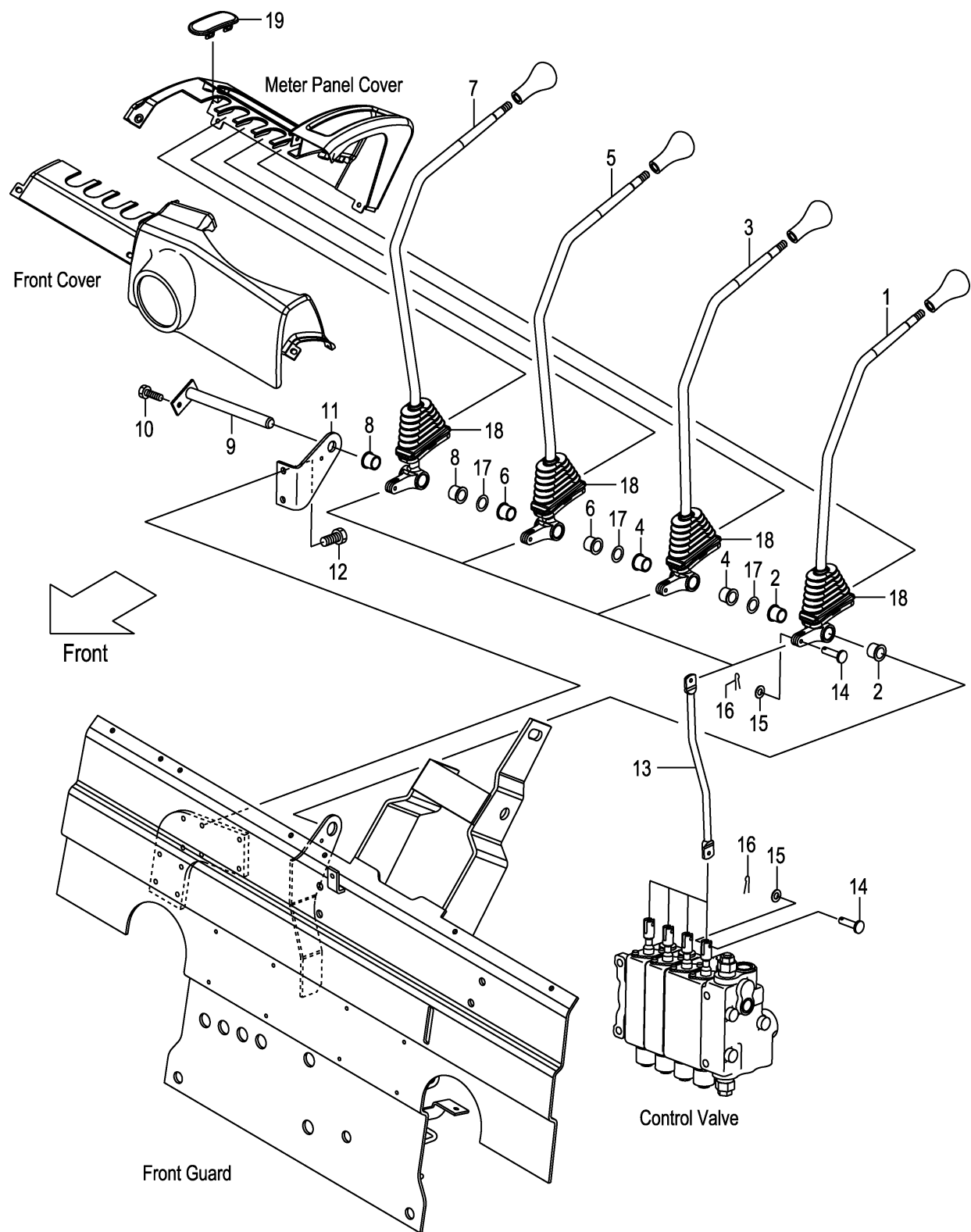
FIG.139 VALVE CONTROL [4SV] (F7Z373C0) バルブコントロール
