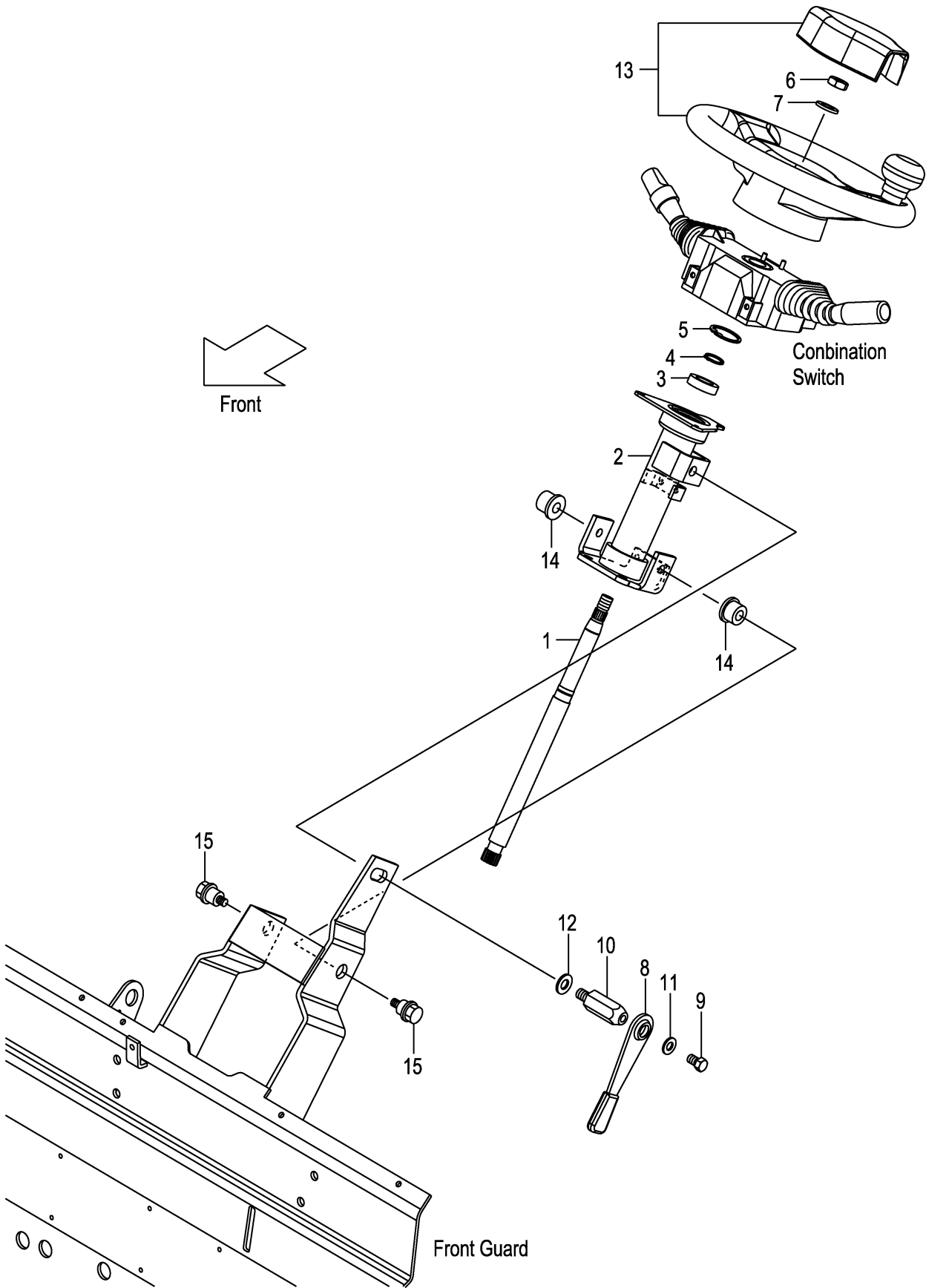
FIG.71 STEERING WHEEL UNIT (F7Z34110) ステアリングホイールユニット
