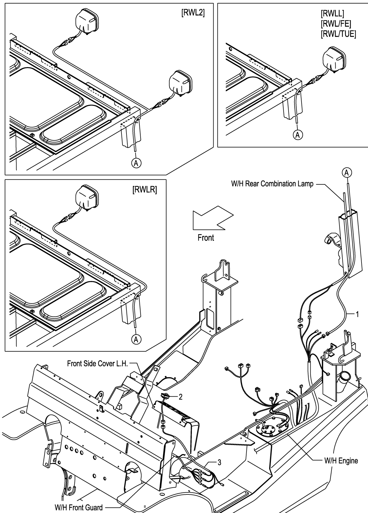
FIG.34 REAR WORKING LIGHT WIRE HARNESS [RWL] (F7Z324T0) リヤーワーキングライトワイヤハーネス
