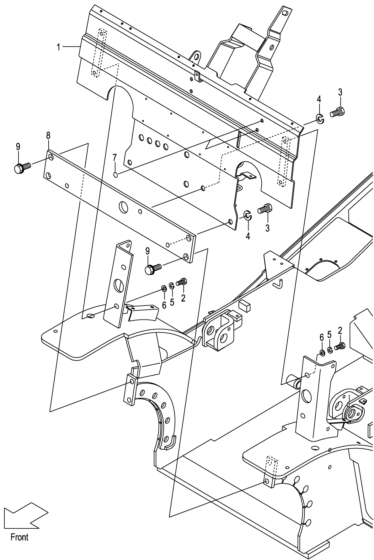
FIG.118 FRONT GUARD (F7Z36410) フロントガード
