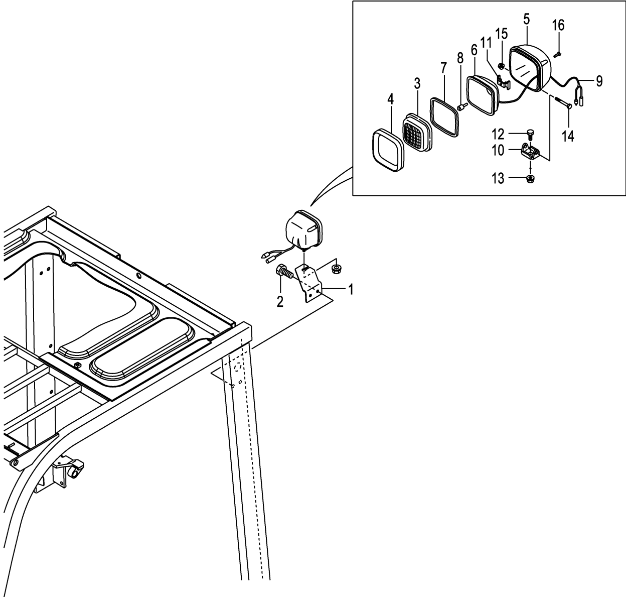
FIG.31 REAR WORKING LIGHT [RWLL] (F7Z324Q0) リヤワーキングライト
