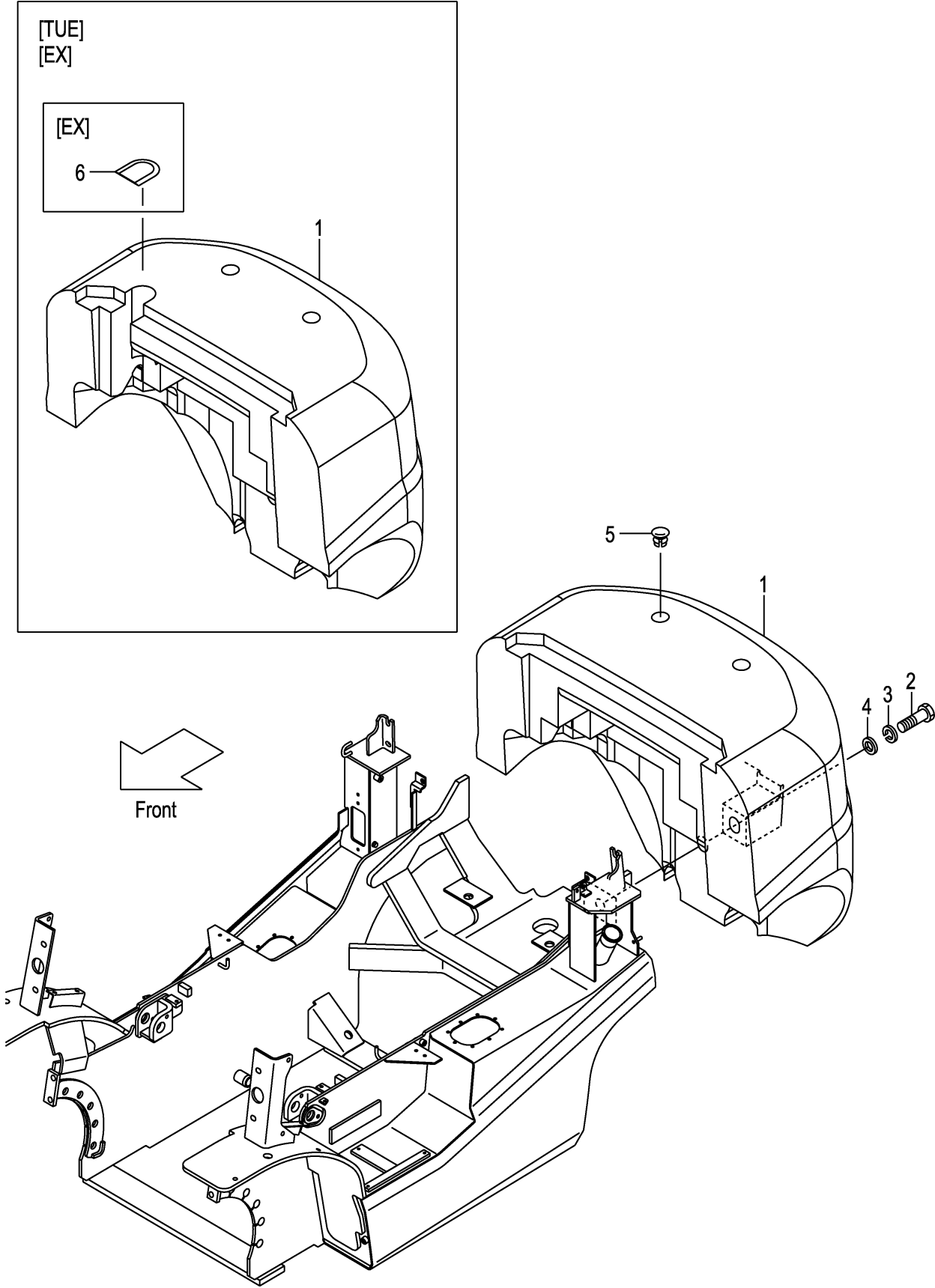
FIG.116 BALANCE WEIGHT (F7Z36310) バランスウエイト
