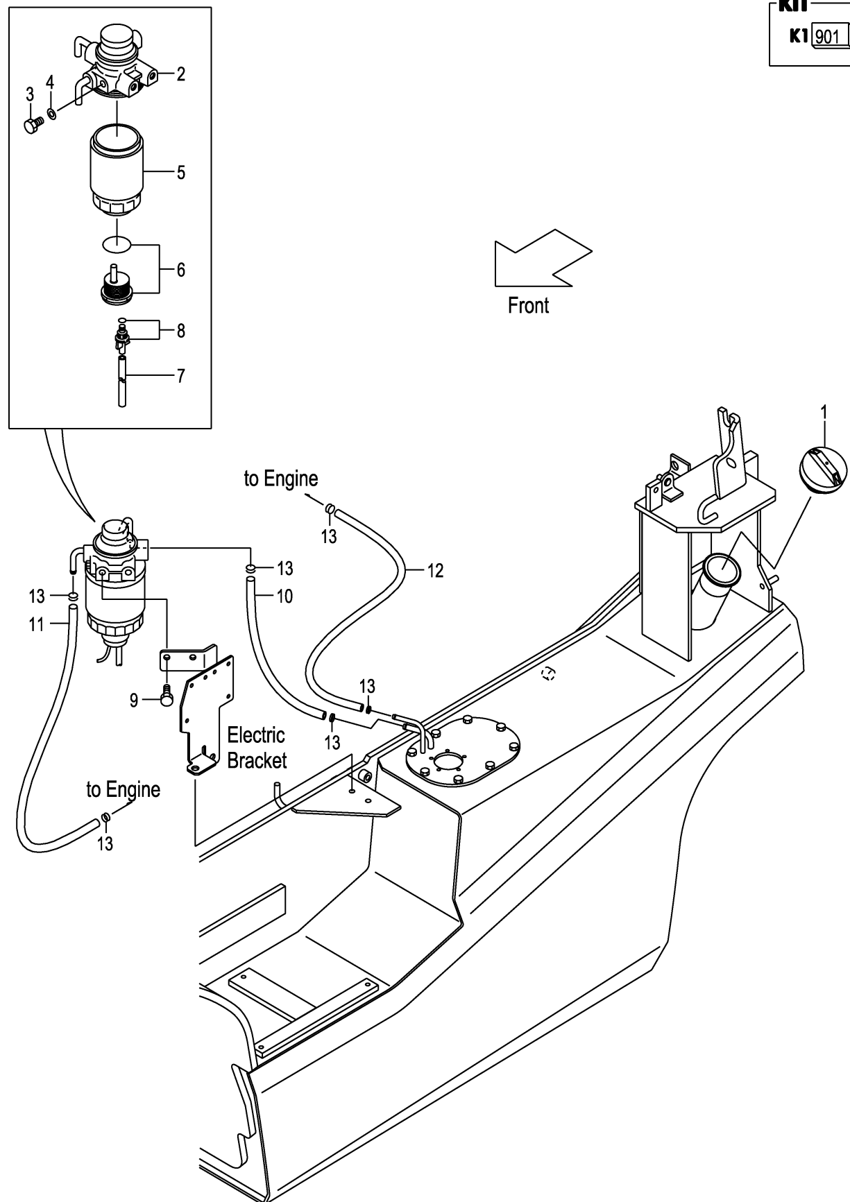
FIG.10 FUEL SYSTEM (F7Z32220) フューエルシステム
