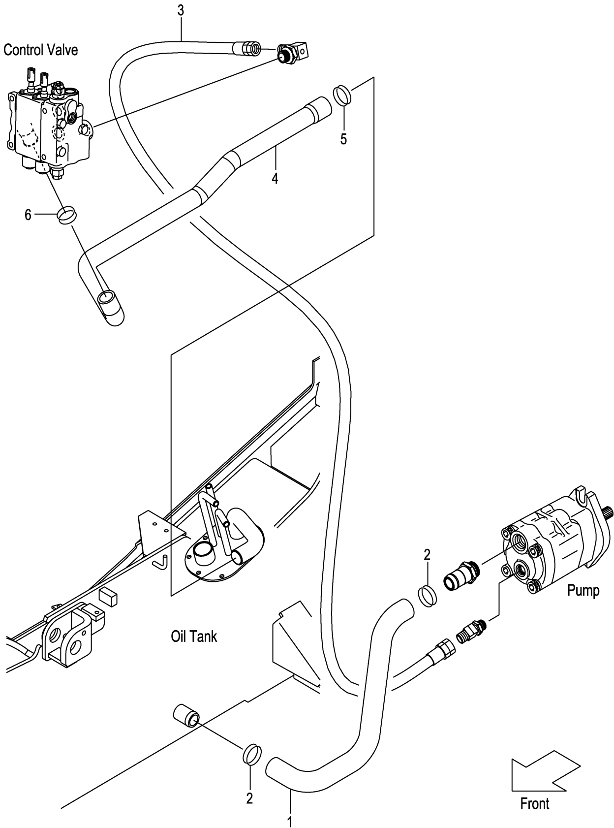
FIG.142 HYDRAULIC LINE (MAIN)(1/4) (F7Z37630) ハイドロリックライン(メイン)(1/4)
