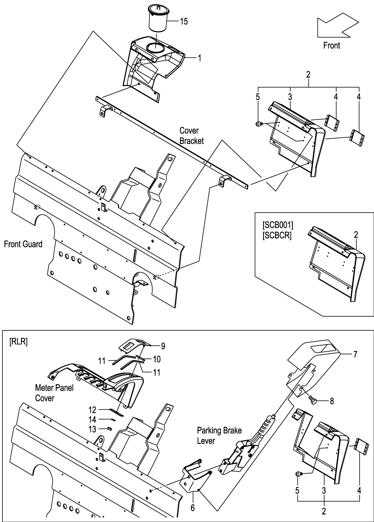
FIG.128 FRONT SIDE COVER (F7Z364C0) フロントサイドカバー
