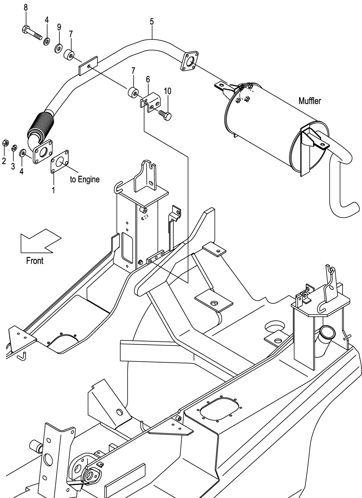
FIG.13 FRONT TUBE & JOINT (F7Z32380) フロントチューブ&ジョイント
