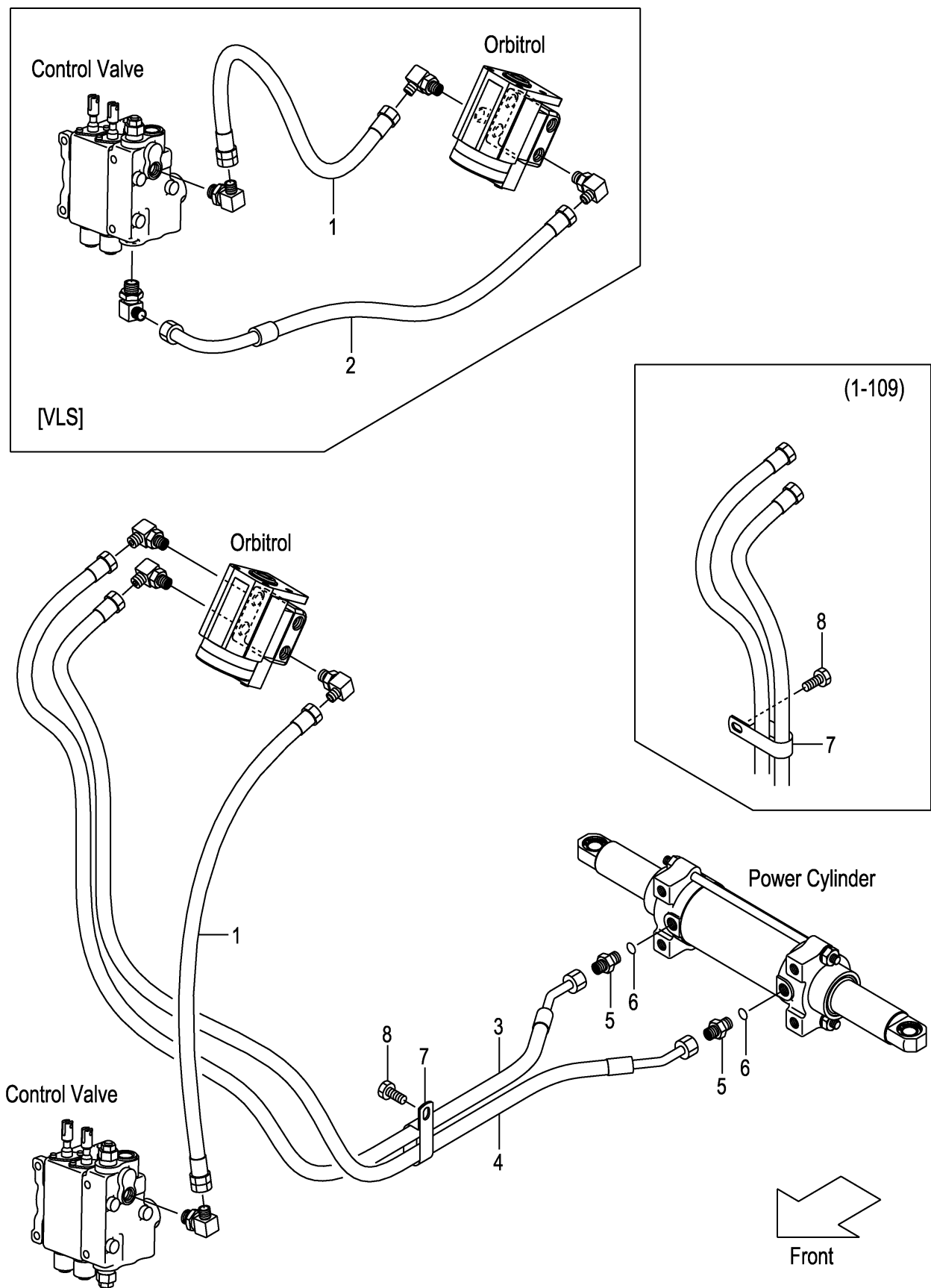
FIG.143 HYDRAULIC LINE (MAIN)(2/4) (F7Z37650) ハイドロリックライン(メイン)(2/4)
