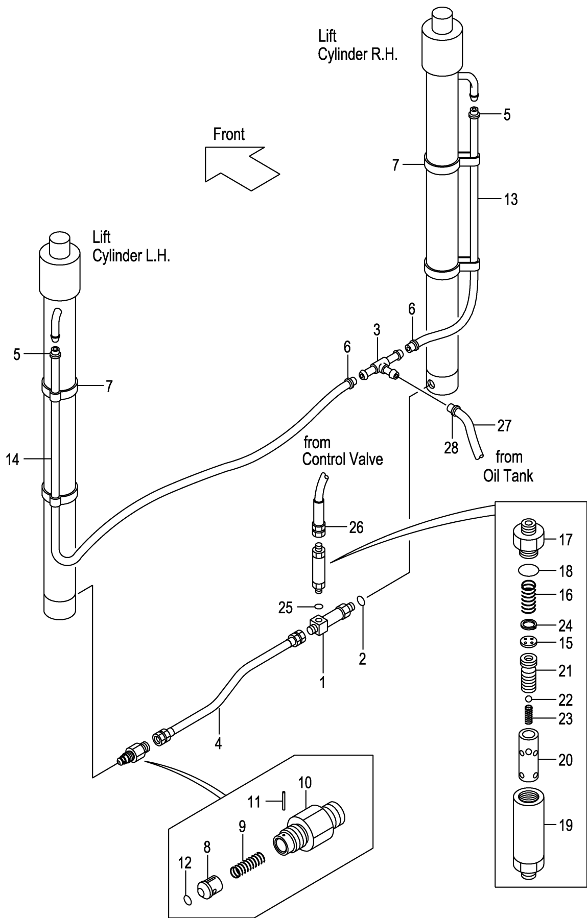
FIG.158 MAST PIPING [VM2N9] (M7028440) マストパイピング
