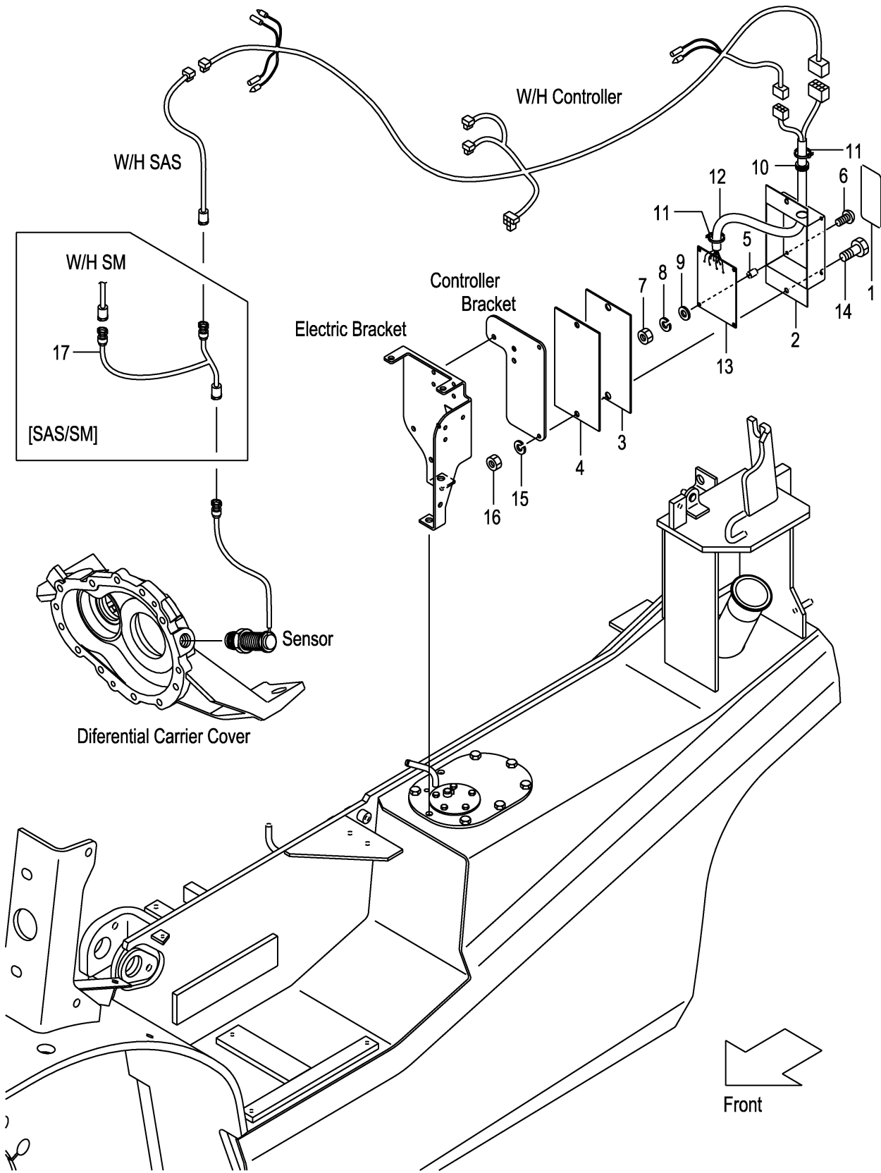
FIG.46 SPEED DETECTOR UNIT [SAS] (F7Z326E0) スピードデテクタユニット
