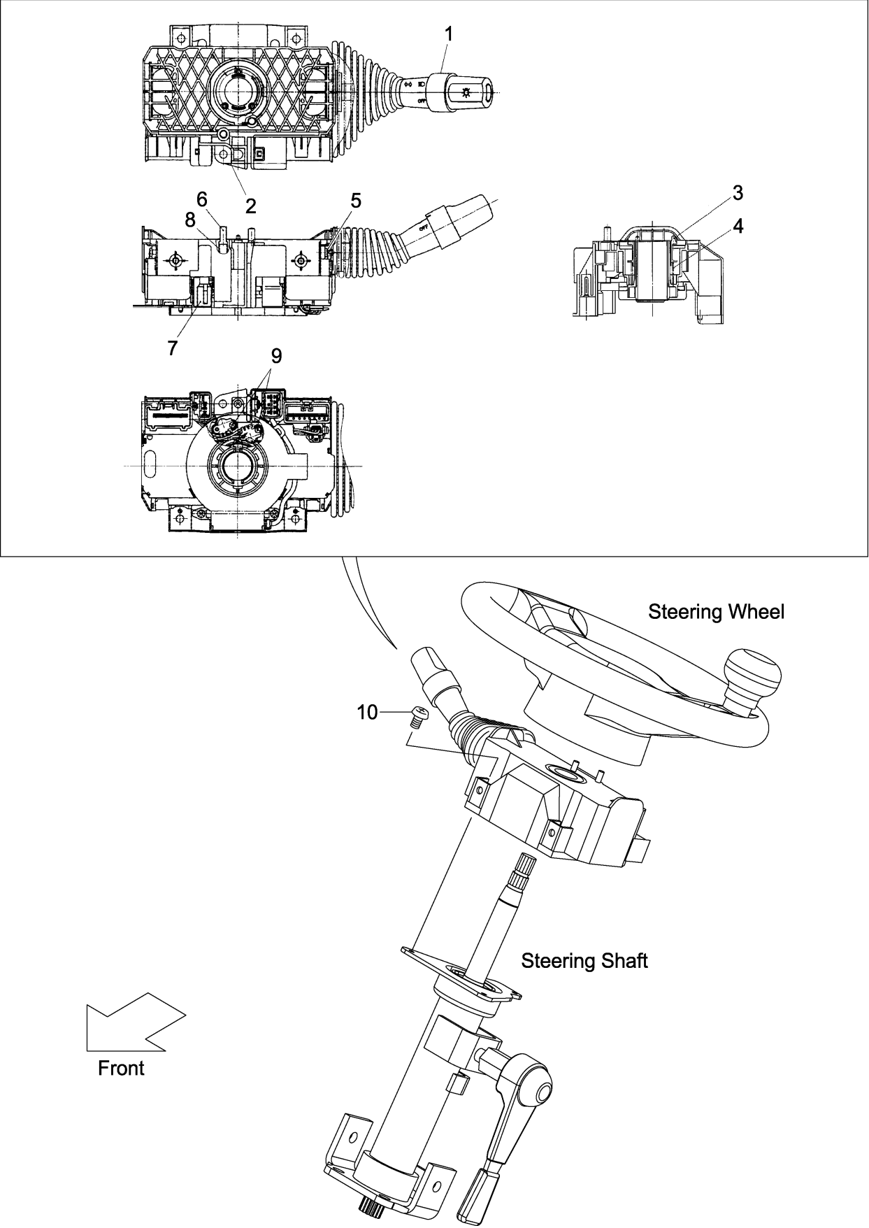
FIG.17 COMBINATION SWITCH (CLUTCH) (F7Z32440) コンビネーションスイッチ
