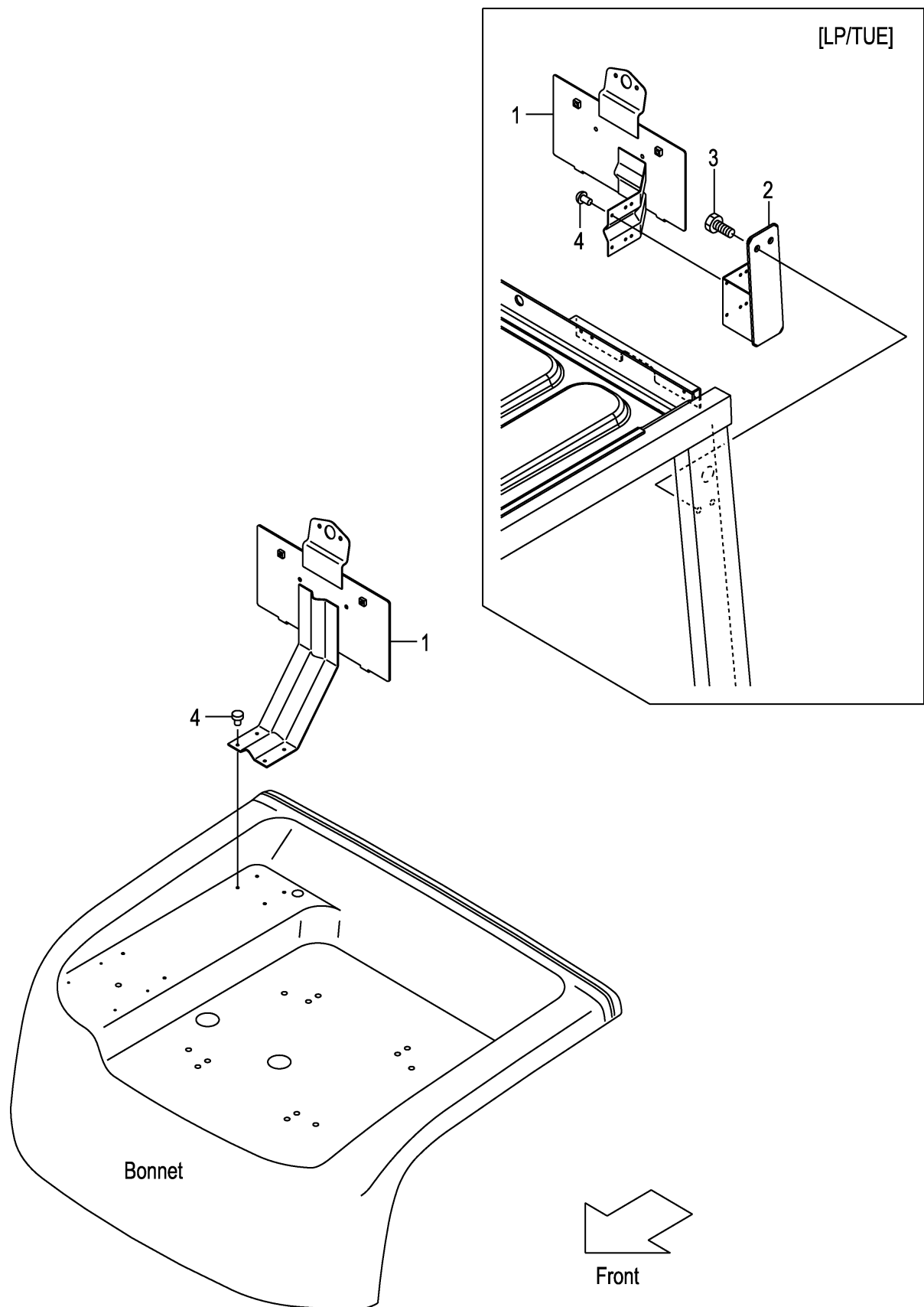
FIG.29 LICENSE LAMP [LP] (F7Z324N0) ライセンスランプ°
