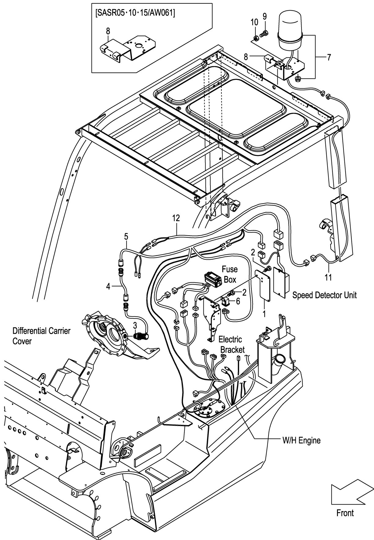
FIG.48 SPEED ALARM SYSTEM [SASR] (F7Z326G0) スピード・アラームシステム
