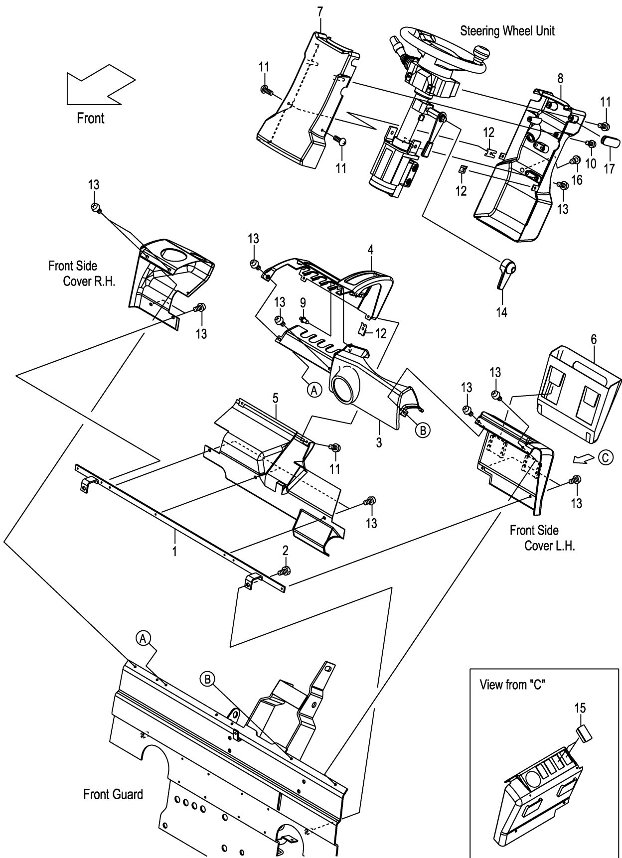
FIG.124 FRONT COVER (CLUTCH) (F7Z36470) フロントカバー
