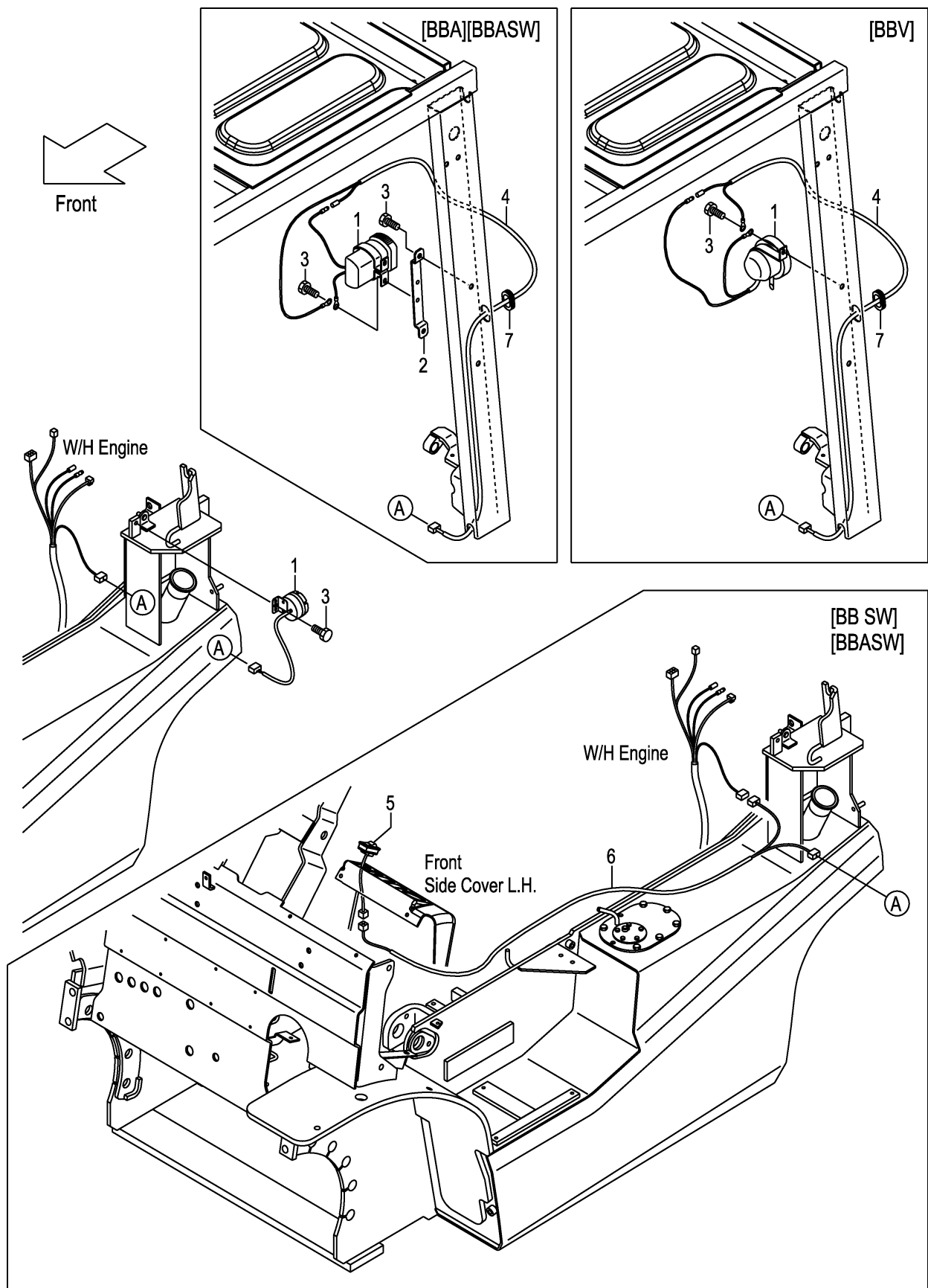
FIG.39 BACK BUZZER (F7Z324X0) バックブザー
