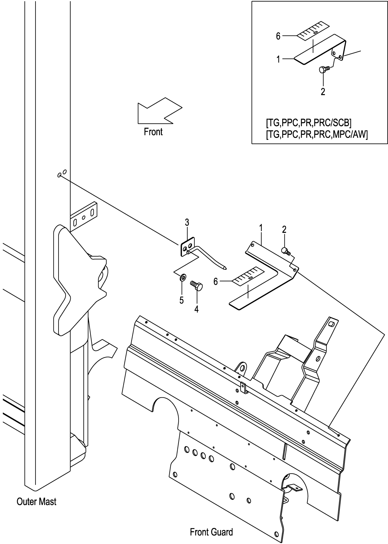
FIG.163 TILT GAUGE [VFM2N9/(TG,PPC,PR,PRC,MPC)] (M7020440) ティルトゲージ
