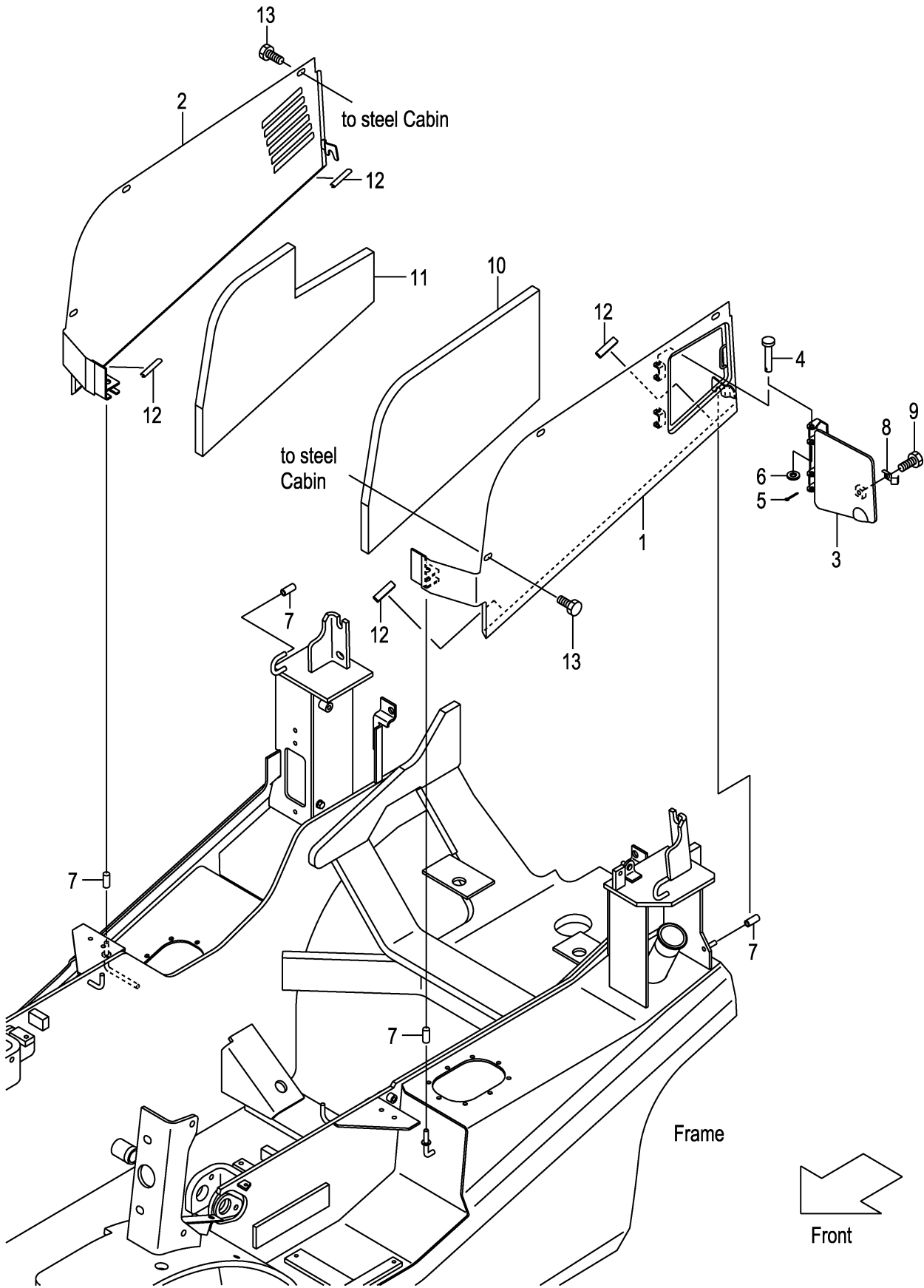
FIG.127 SIDE COVER [SCB001][SCBCR] (F7Z364B0) サイドカバー
