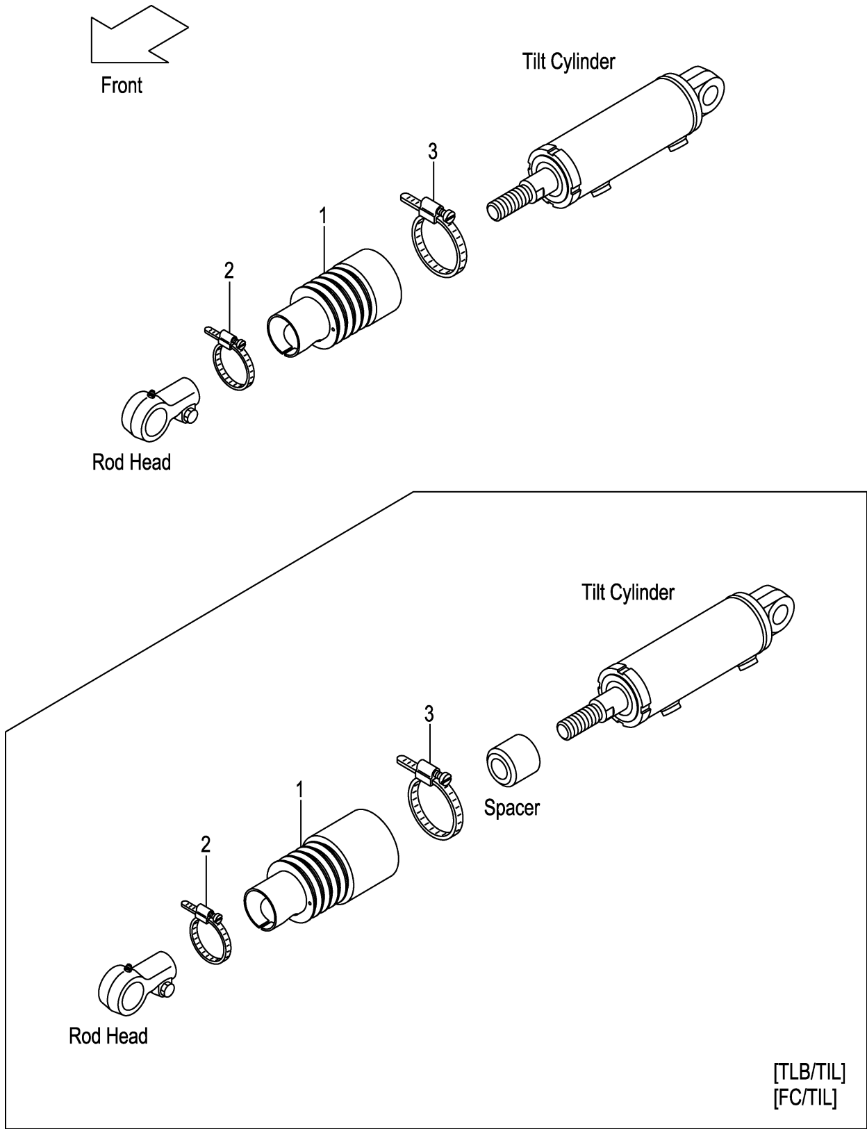
FIG.148 TILT BOOT [TLB][FC] (F7Z38520) ティルトブーツ
