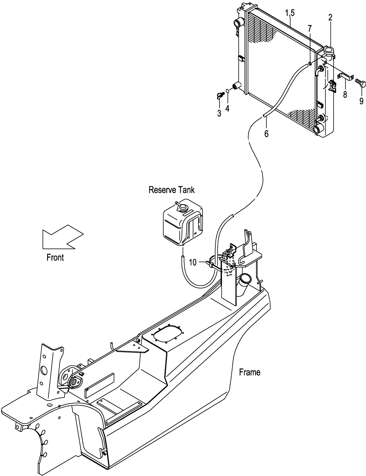
FIG.5 COOLING UNIT (TOR-CON) (F7Z32120) クーリングユニット
