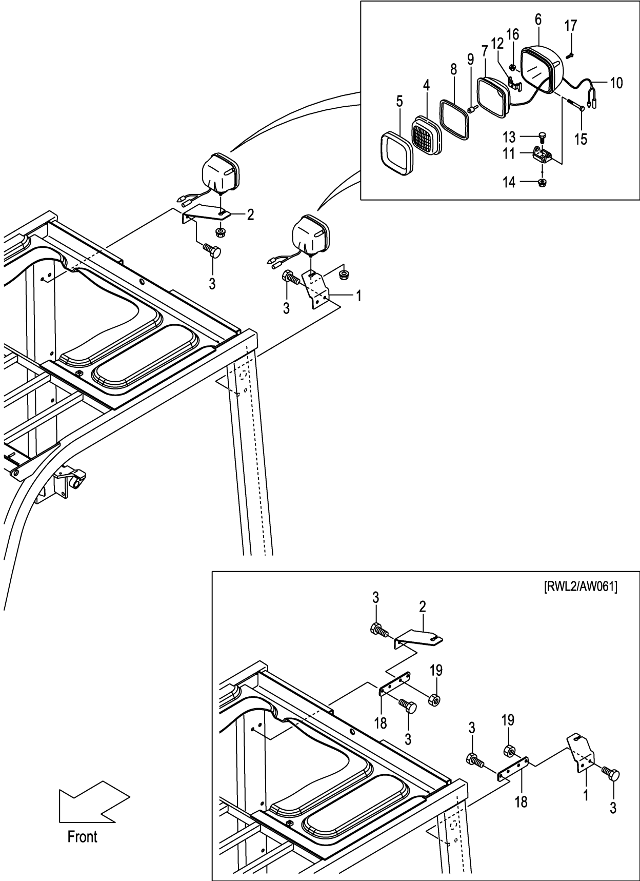
FIG.32 REAR WORKING LIGHT [RWL2] (F7Z324R0) リヤワーキングライト
