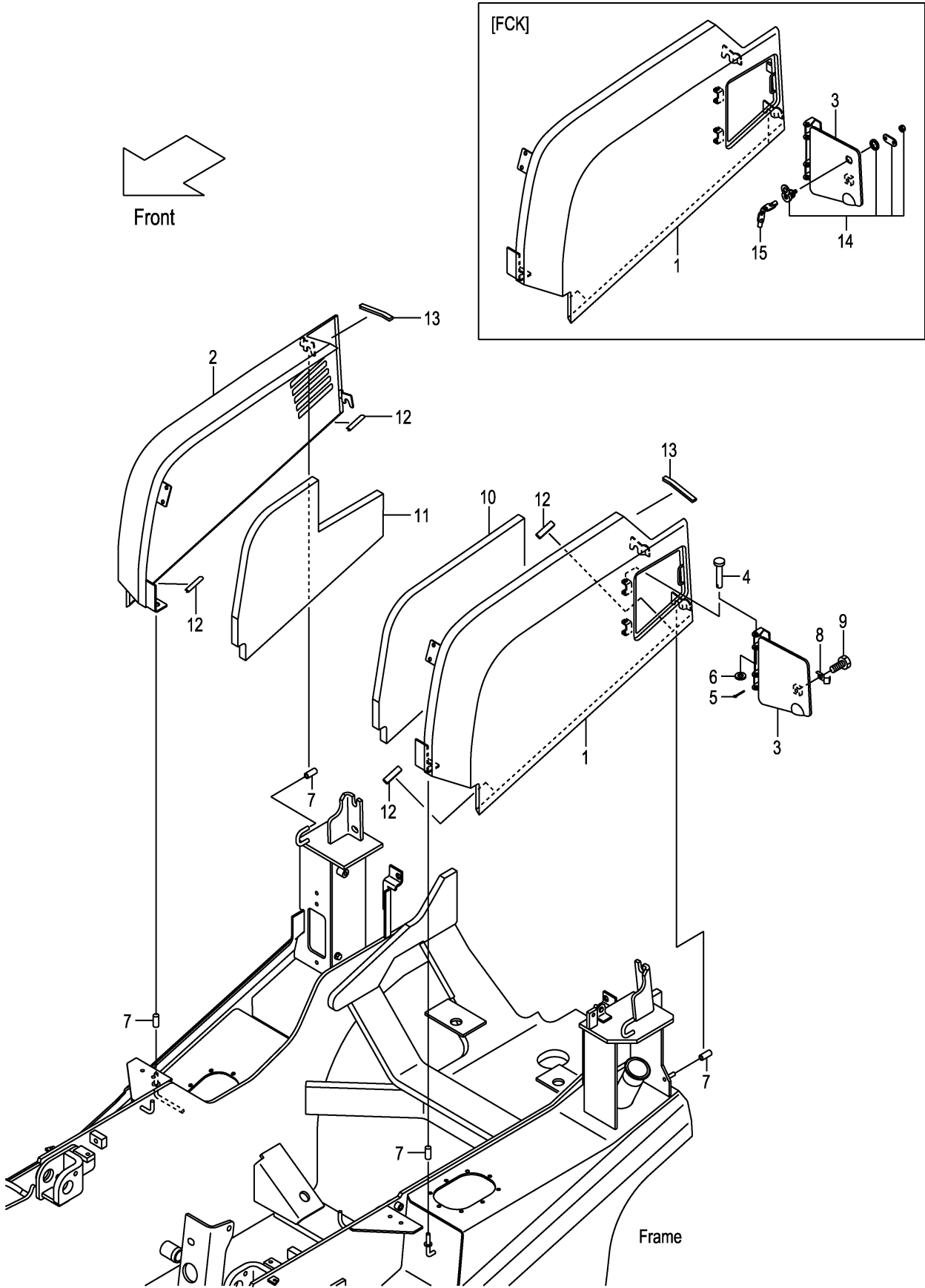
FIG.126 SIDE COVER (F7Z364A0) サイドカバー
