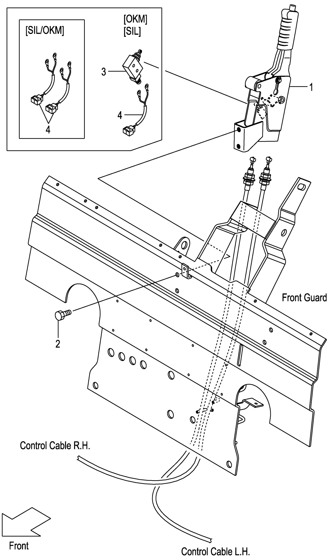
FIG.111 BRAKE LEVER (F7Z35510) ブレーキレバー
