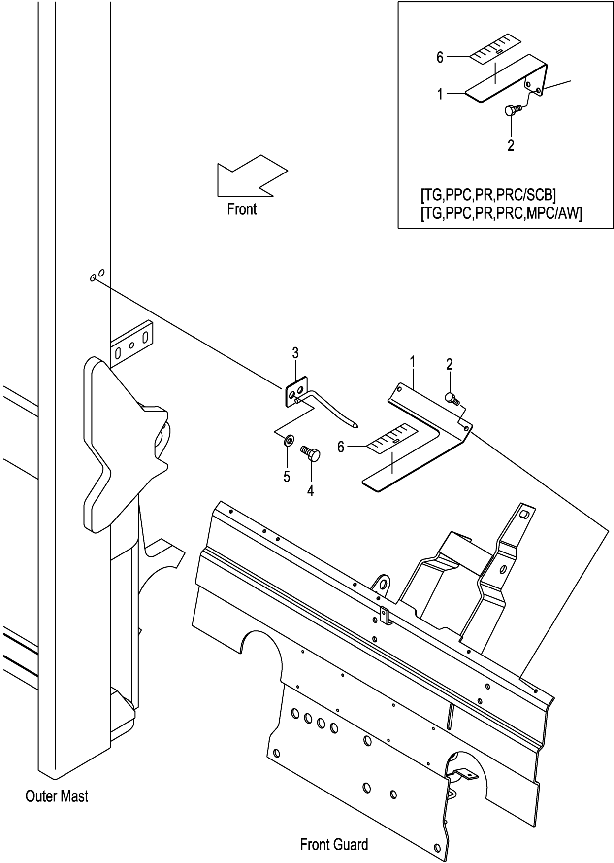
FIG.171 TILT GAUGE [VFHM2N9/(TG,PPC,PR,PRC,MPC)] (M7020750) ティルトゲージ
