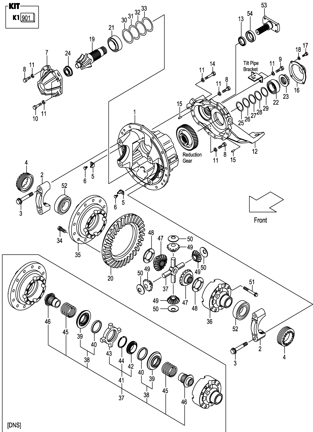
FIG.69 DIFFERENTIAL (F7Z33530) デイファレンシャル
