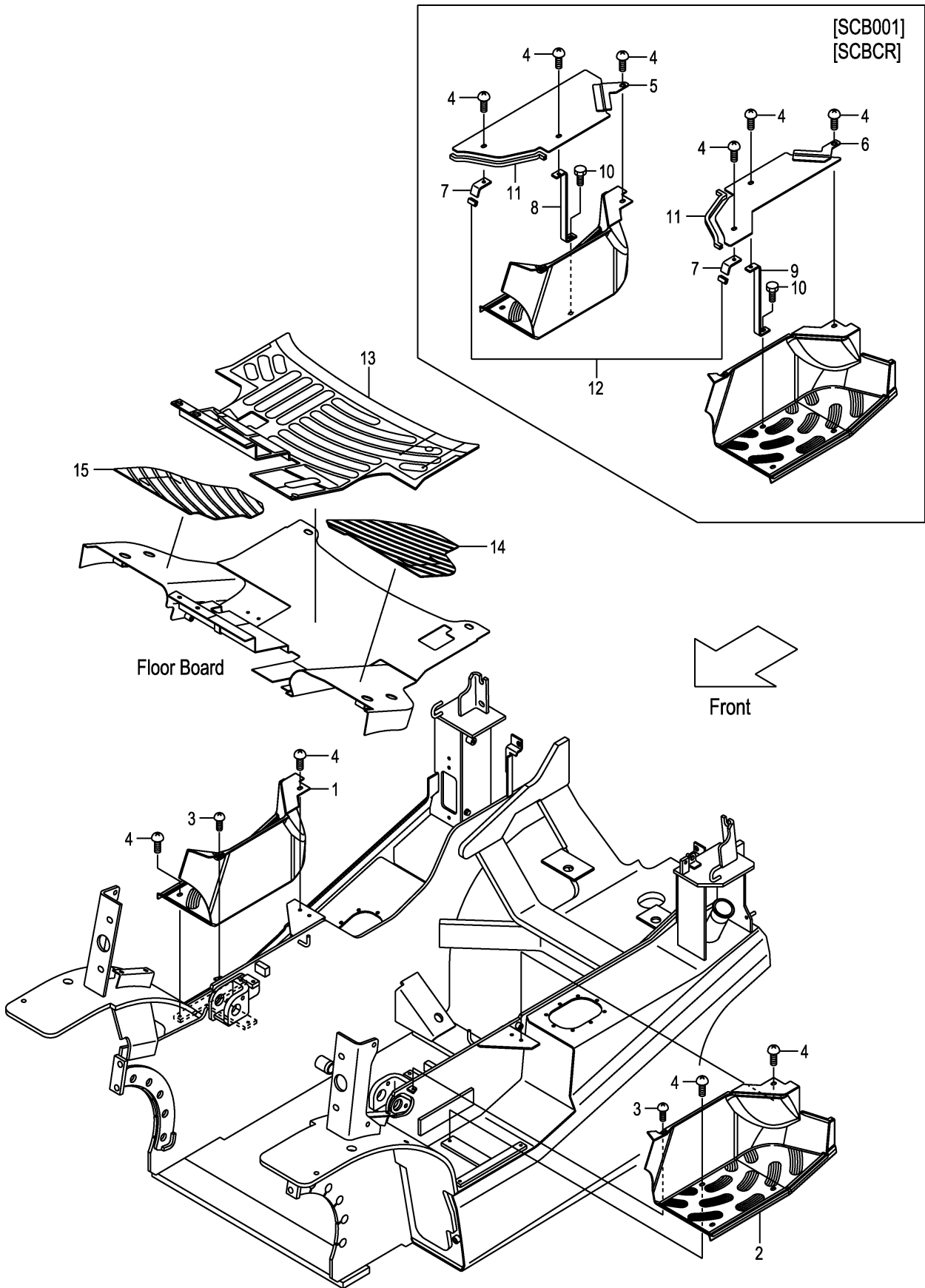
FIG.123 STEP & FLOOR MAT (F7Z36460) ステップ&フロアマット
