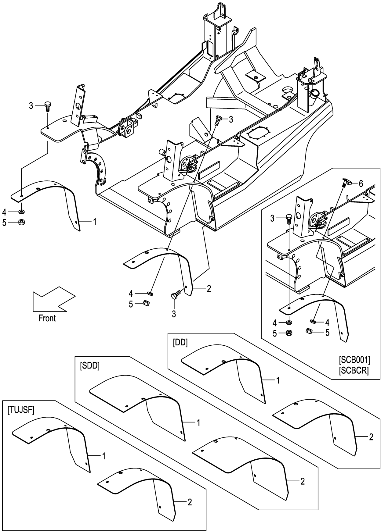
FIG.77 FENDER (F7Z34420) フェンダ
