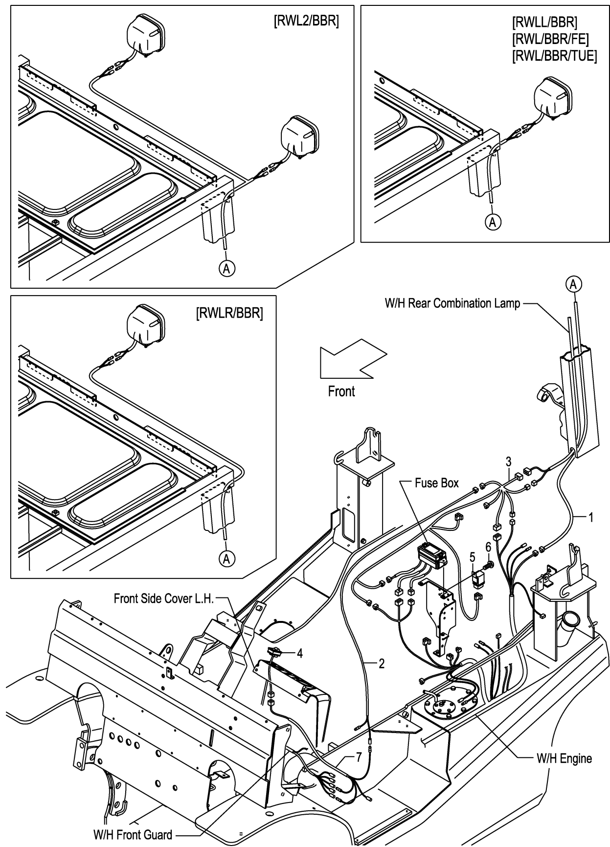
FIG.35 REAR WORKING LIGHT WIRE HARNESS [RWL/BBR] (F7Z324U0) リヤワーキングライトワイヤハーネス
