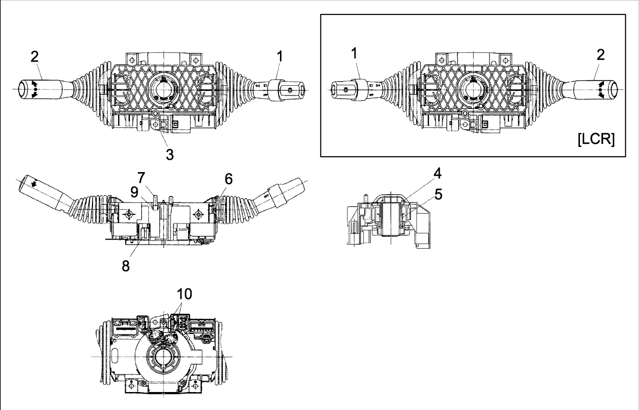
FIG.18 COMBINATION SWITCH (TOR-CON) (F7Z32450) コンビネーションスイッチ
