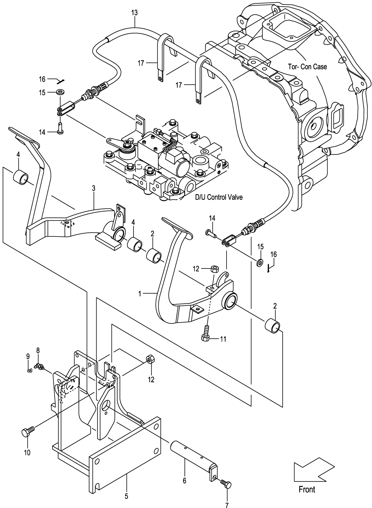
FIG.102 FOOT PEDAL (TOR-CON) (F7Z35420) フットペダル
