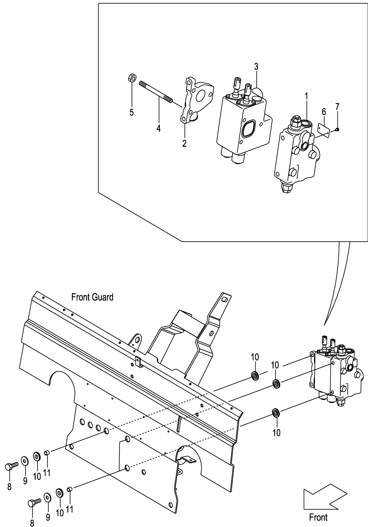
FIG.132 CONTROL VALVE [2SV] (F7Z37310) コントロールバルブ
