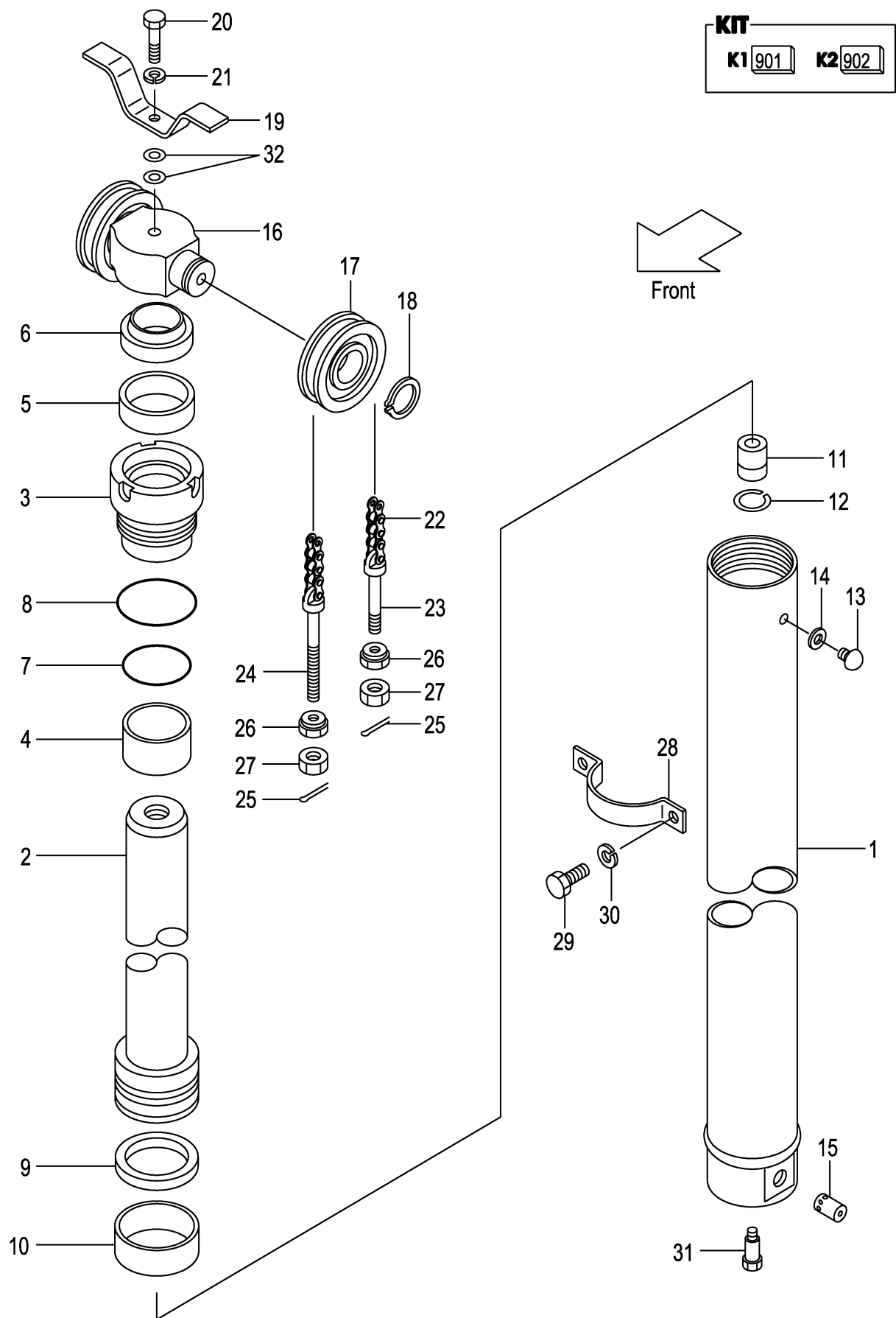
FIG.164 LIFT CYLINDER (FRONT) [VFM2N9] (M7020540) リフトシリンダ(フロント)
