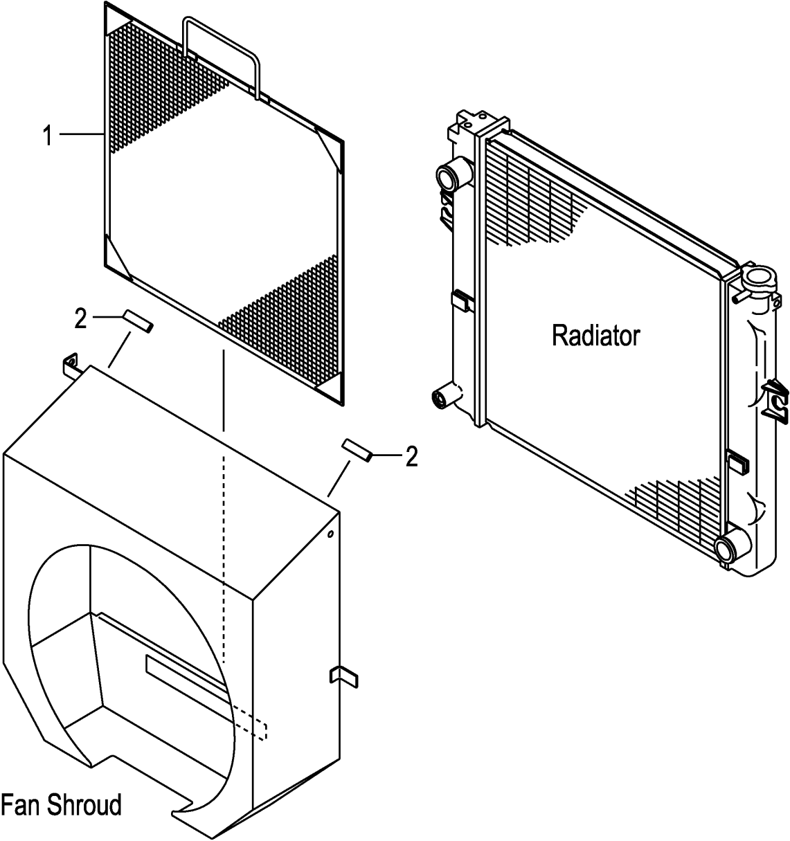
FIG.9 DUST SCREEN [DSR006][DSR008] (F7Z32180) ダストスクリーン
