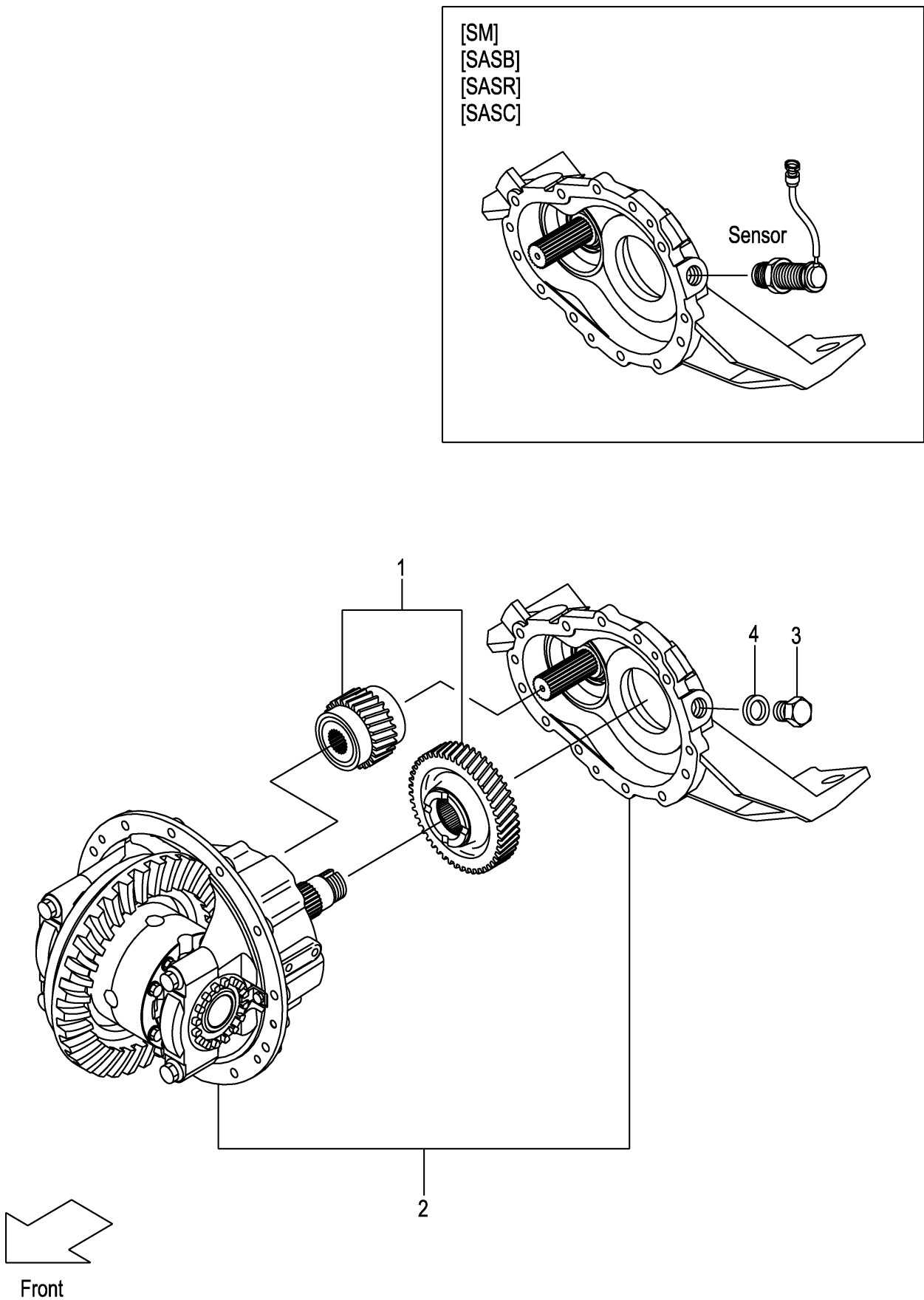
FIG.67 REDUCTION & DIFFERENTIAL (F7Z33510) リダクション&ディファレンシャル
