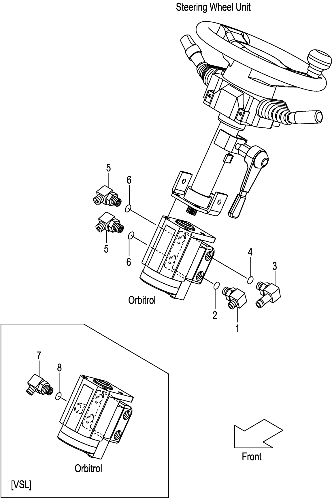
FIG.73 ORBITROL FITTING (F7Z34140) オービットロールフィッティング
