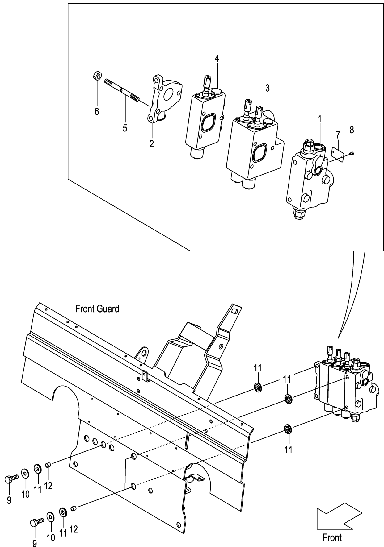
FIG.133 CONTROL VALVE [3SV] (F7Z37320) コントロールバルブ
