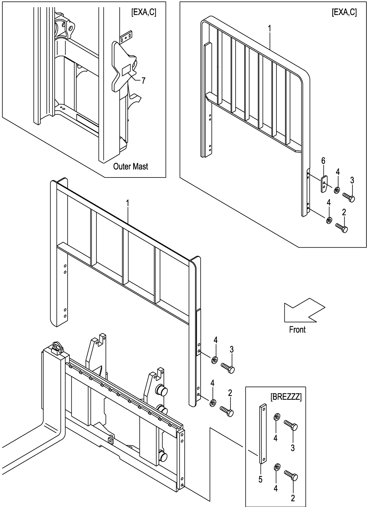
FIG.161 BACKREST [VFM2N9] (M7028260) バックレスト
