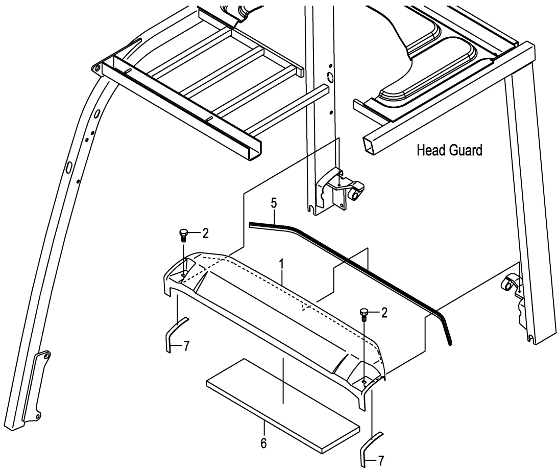
FIG.120 RADIATOR COVER (F7Z36430) ラジエータカバー
