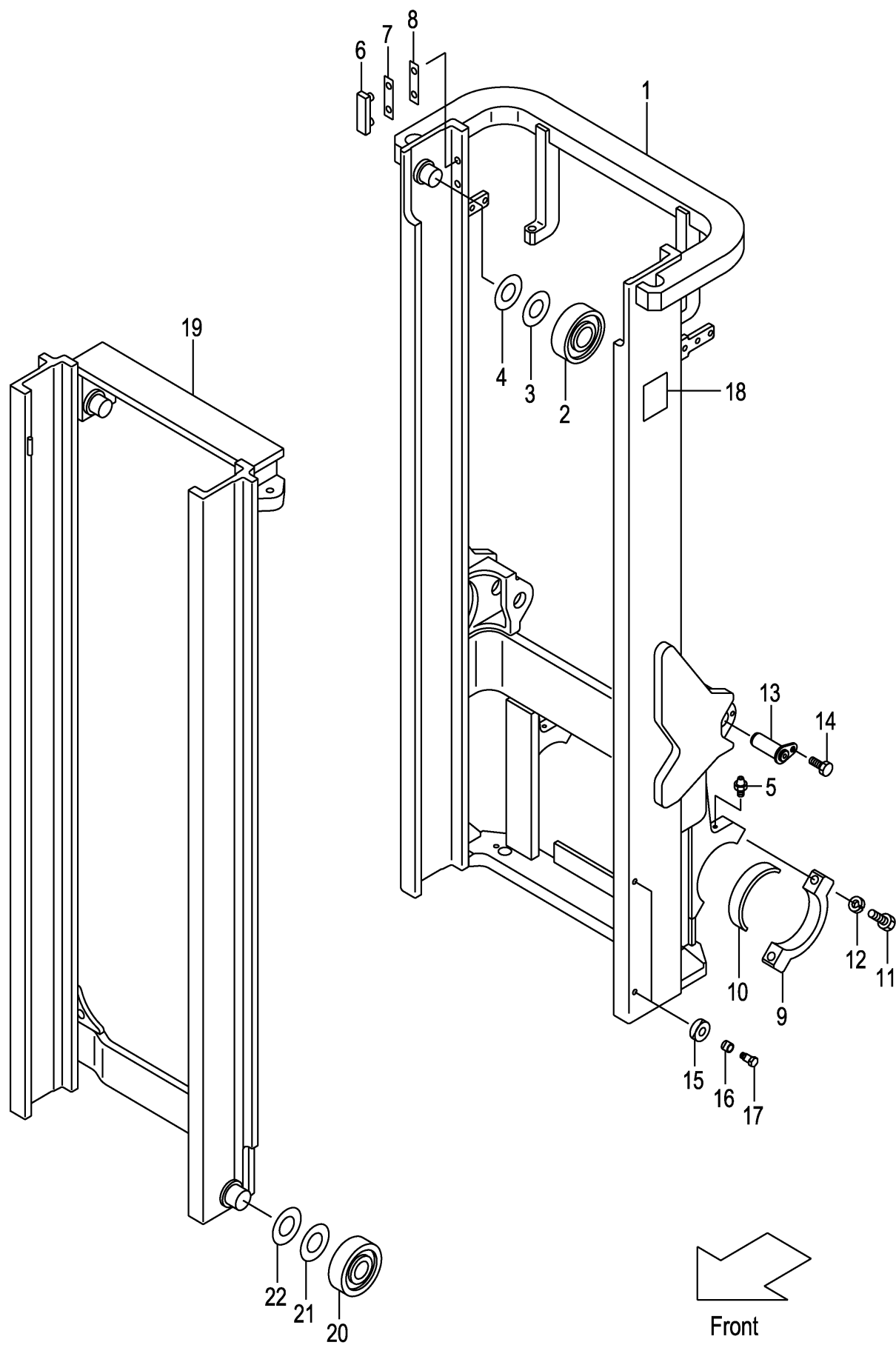
FIG.156 MAST [VM2N9] (M7028320) マスト
