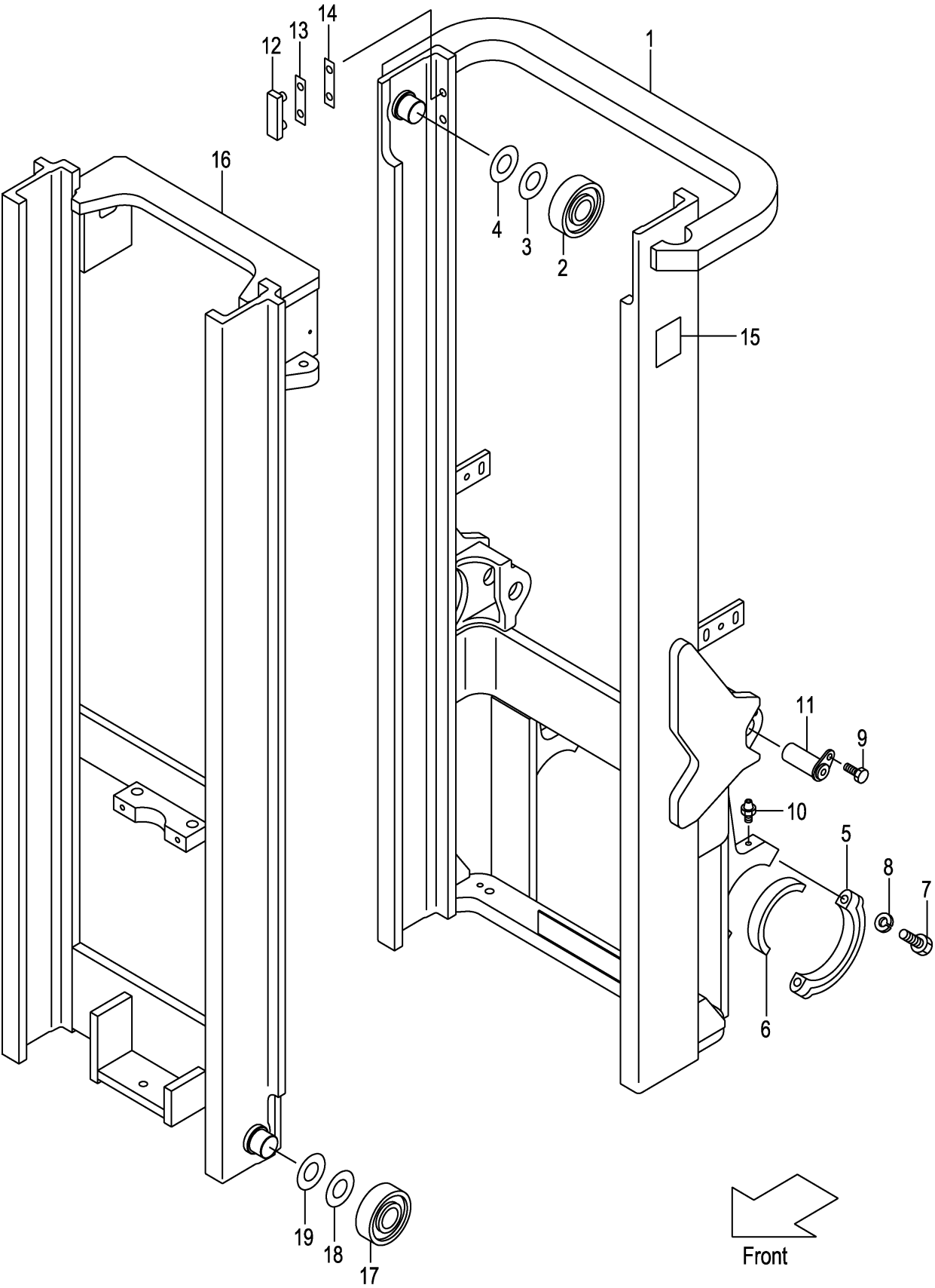
FIG.162 MAST [VFM2N9] (M7020430) マスト
