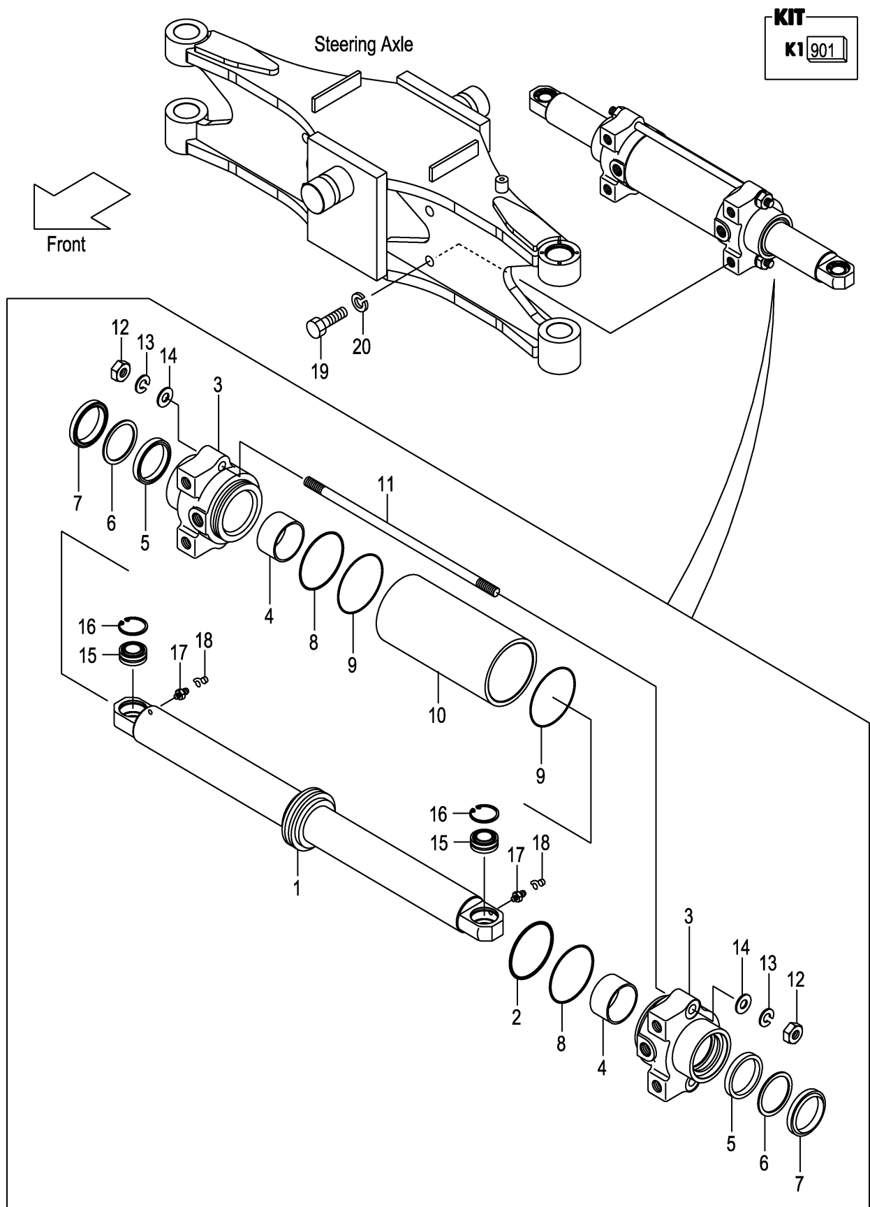
FIG.93 POWER CYLINDER (F7Z34510) パワーシリンダ
