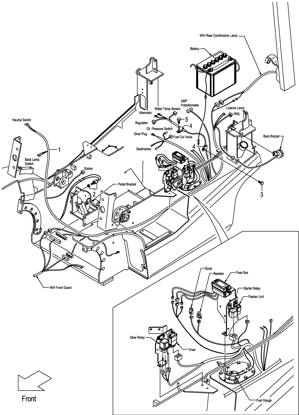
FIG.21 ENGINE WIRE HARNESS (CLUTCH) (F7Z324C0) エンジンワイヤハーネス
