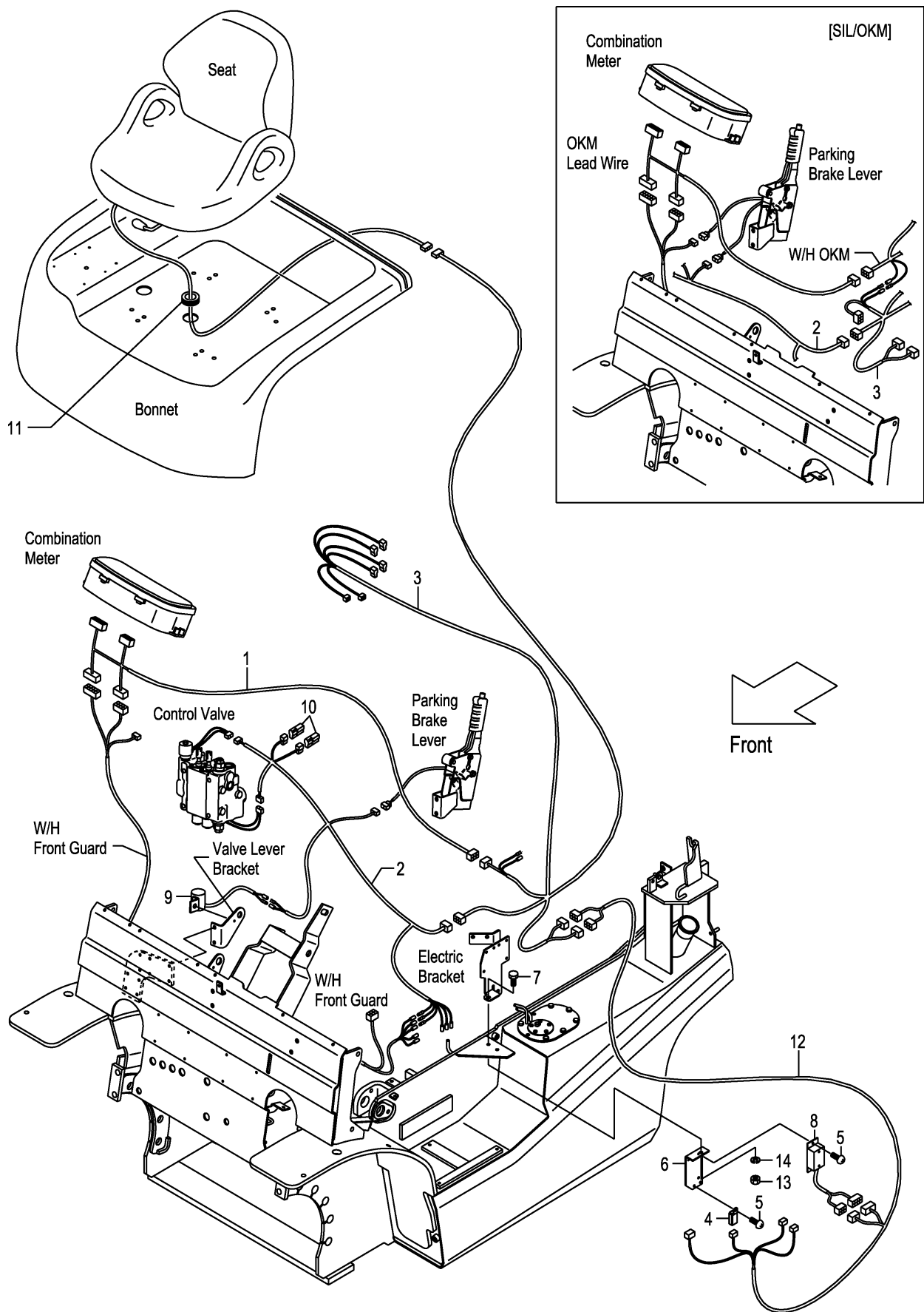
FIG.51 INTERLOCK (CLUTCH):[SIL] (F7Z326M0) インターロック
