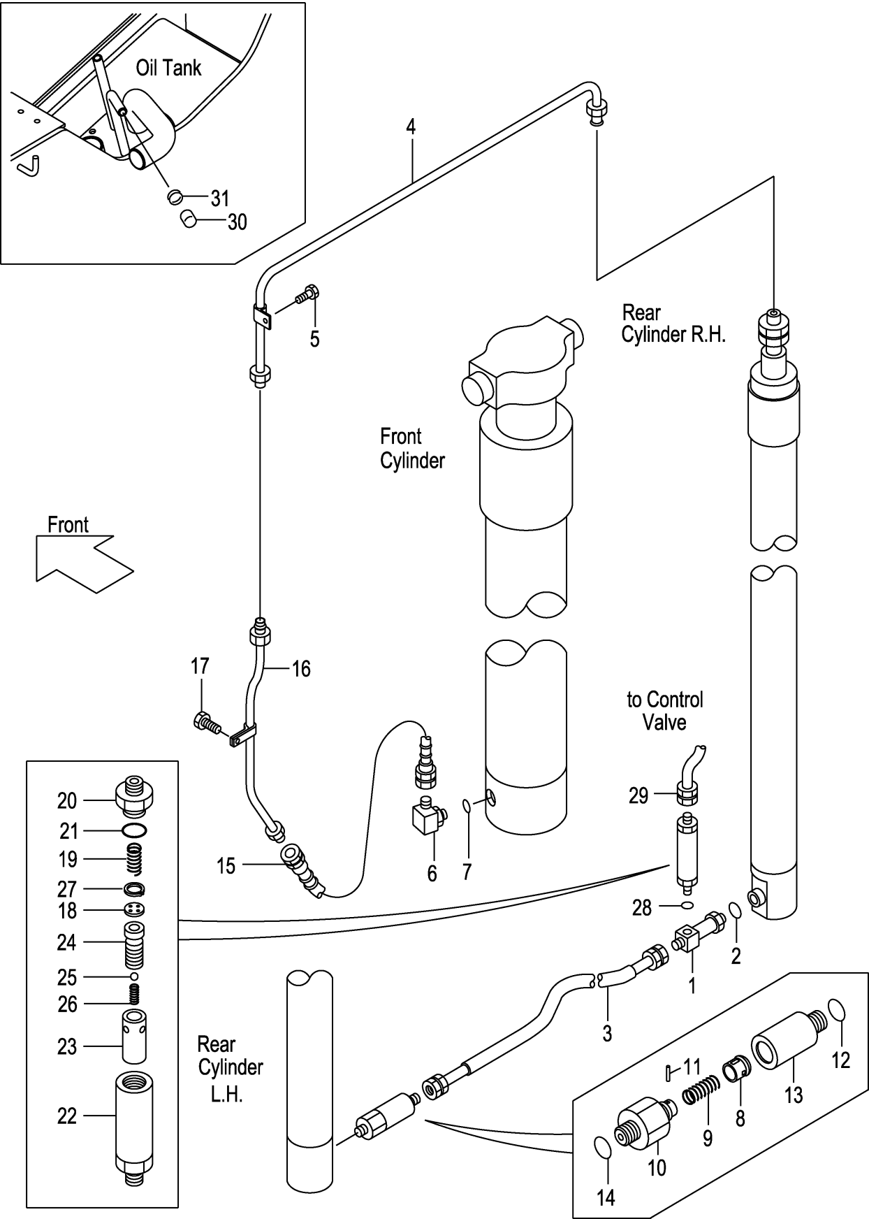
FIG.166 MAST PIPING [VFM2N9] (M7020560) マストパイピング
