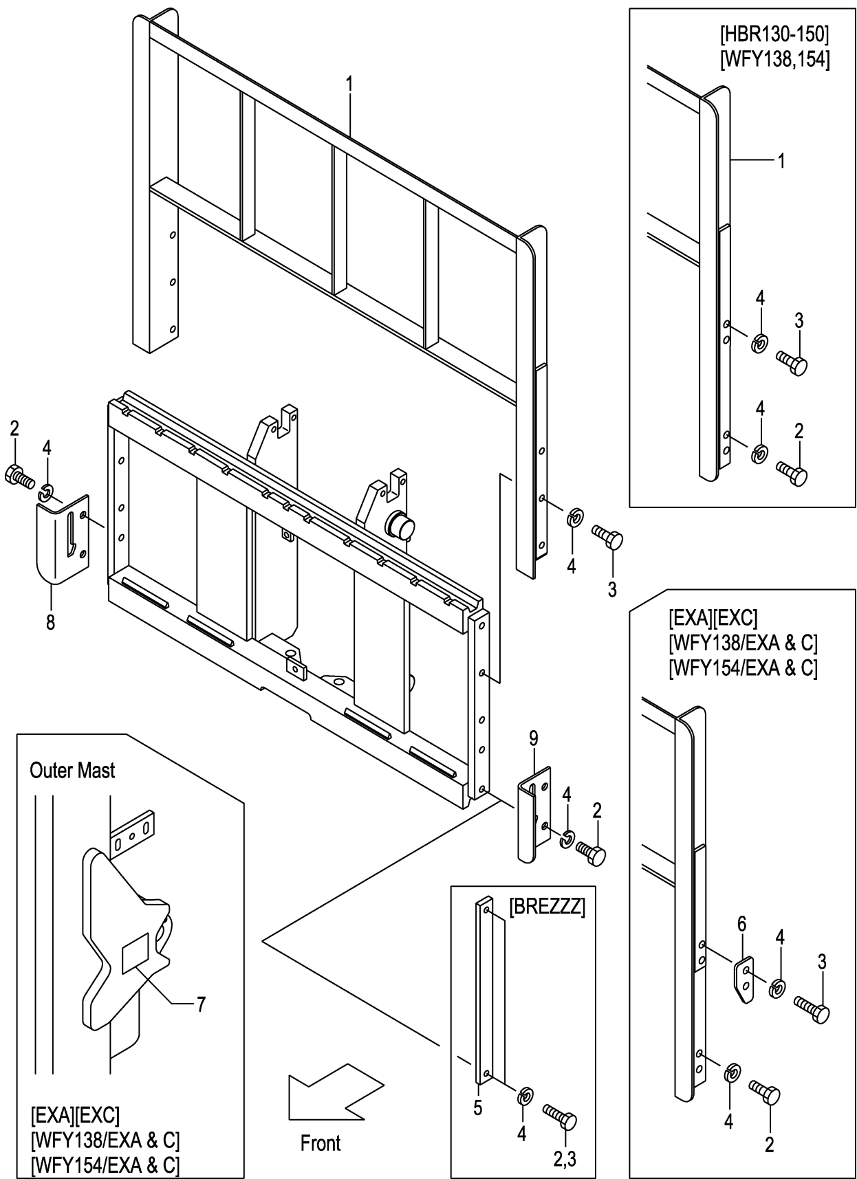
FIG.169 BACKREST [VFHM2N9] (M7028290) バックレスト
