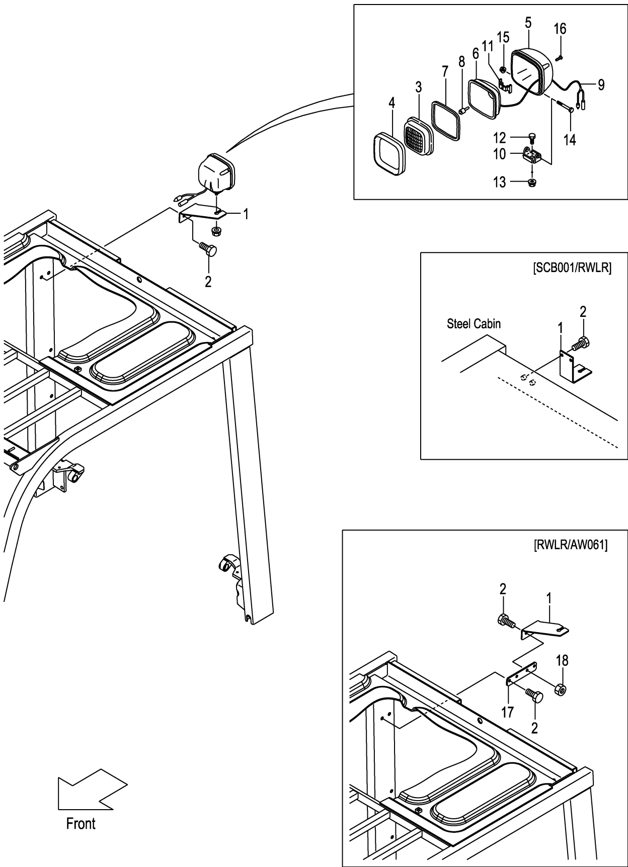
FIG.30 REAR WORKING LIGHT [RWLR] (F7Z324P0) リヤワーキングライト
