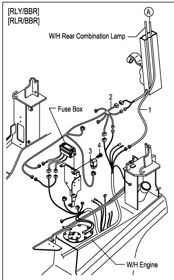
FIG.37 REVOLVING LIGHT WIRE HARNESS [RLY][RLR] (F7Z324W0) リボルビングライトワイヤハーネス
