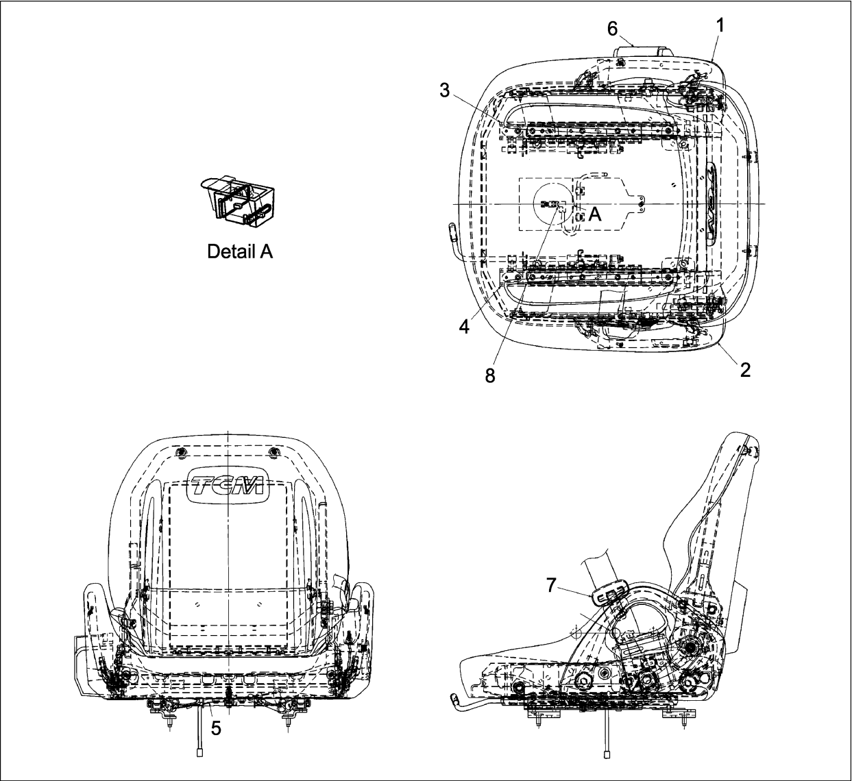
FIG.130 SEAT [HGL] (F7Z36820) シート
