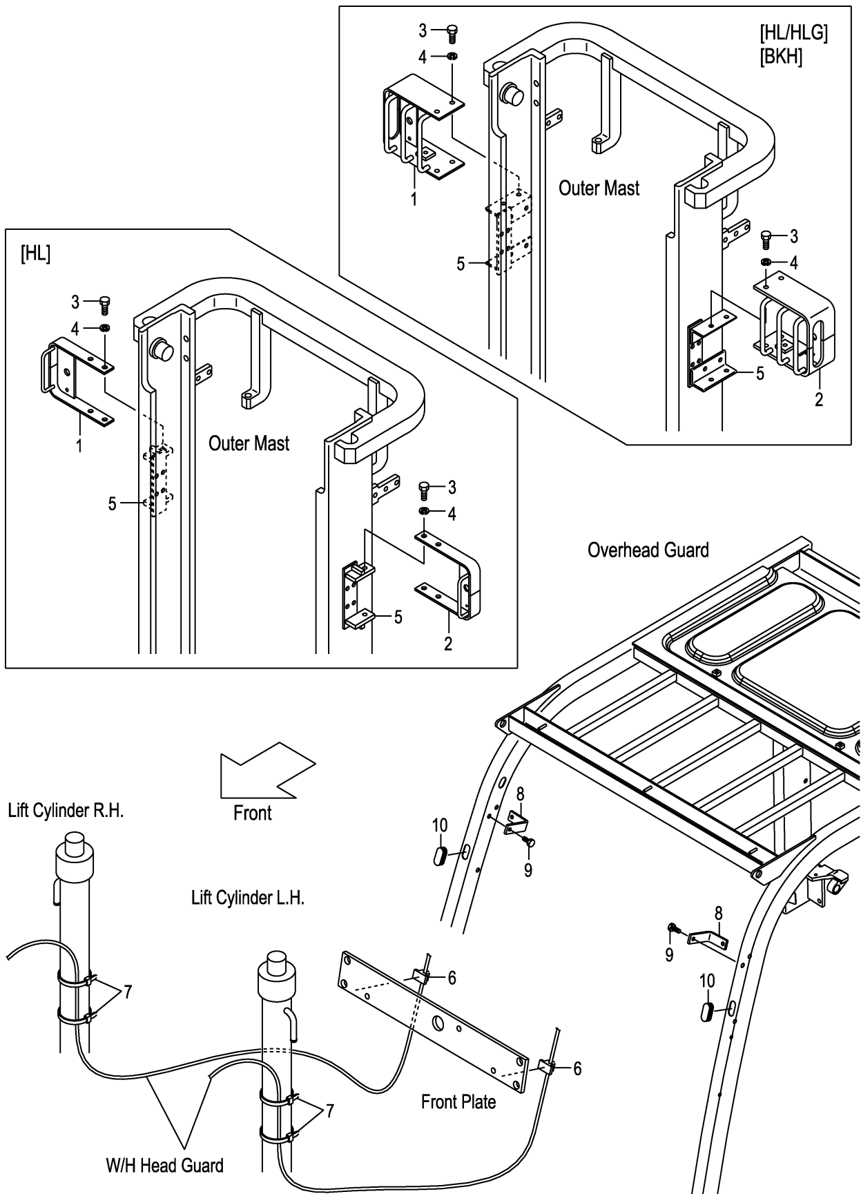
FIG.96 FRONT LAMP BRACKET [HL][BKH] (F7Z35130) フロントランプブラケット
