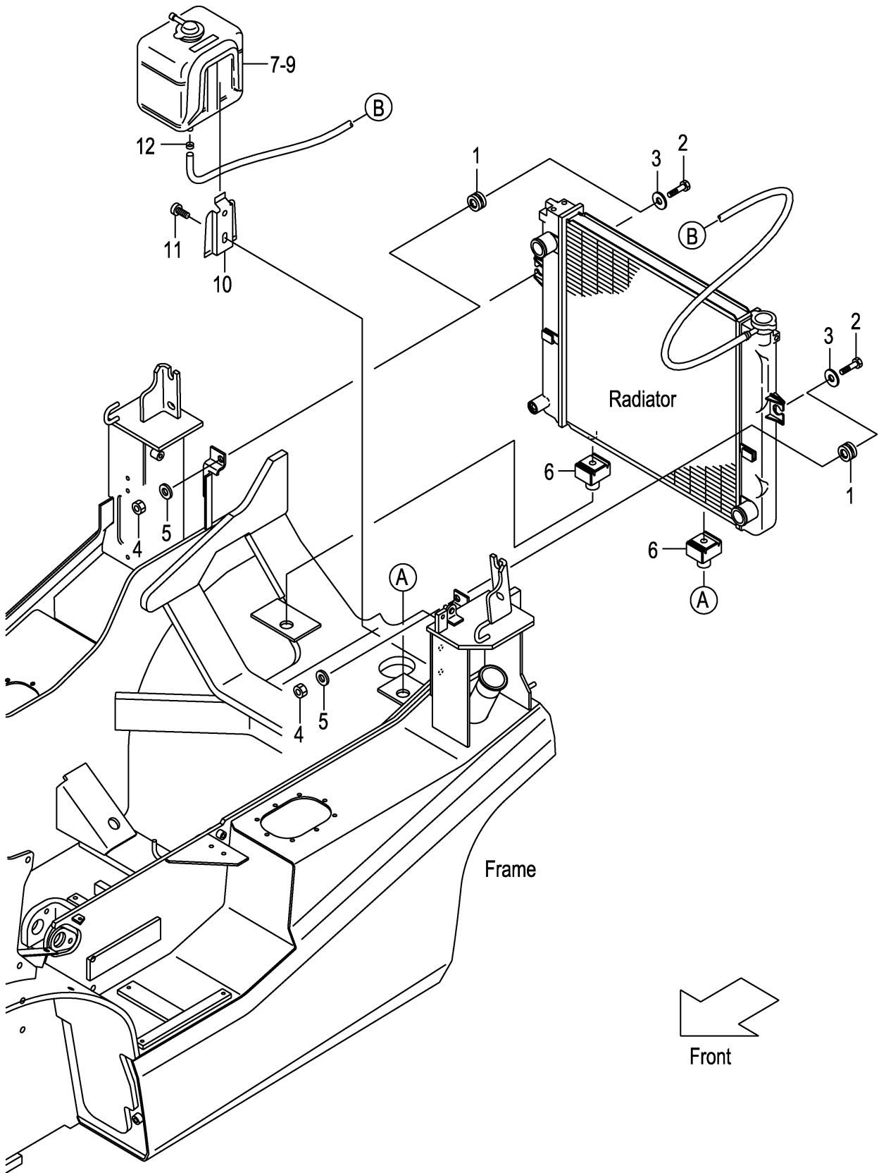
FIG.7 RADIATOR PARTS & RESERVE TANK (F7Z32150) ラジエータパーツ&リザーブタンク
