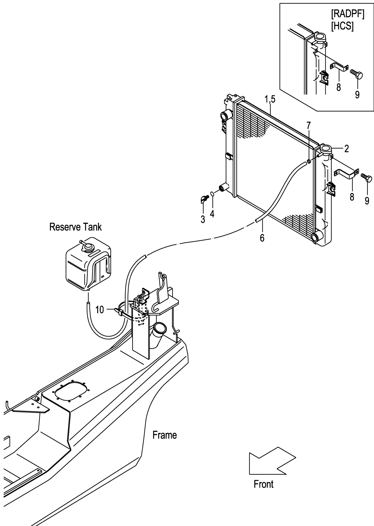
FIG.4 COOLING UNIT (CLUTCH) (F7Z32110) クーリングユニット
