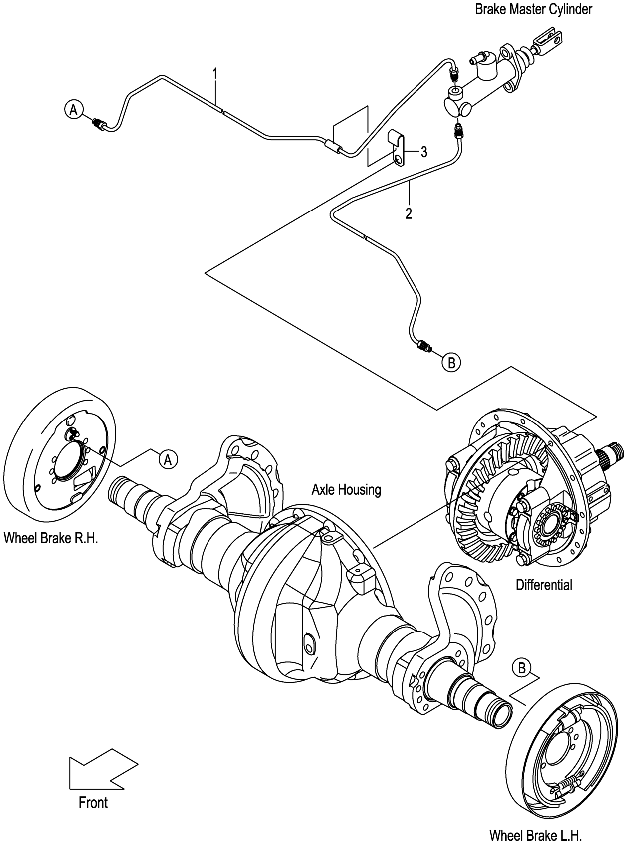
FIG.106 BRAKE PIPE (TOR-CON) (F7Z354A0) ブレーキパイプ
