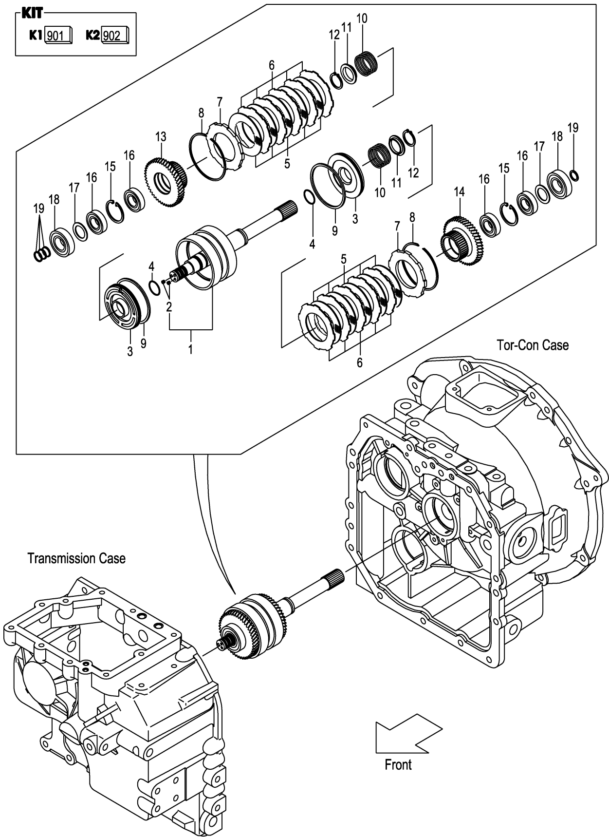
FIG.62 CLUTCH PACK (TOR-CON) (F7Z325B0) クラッチパック
