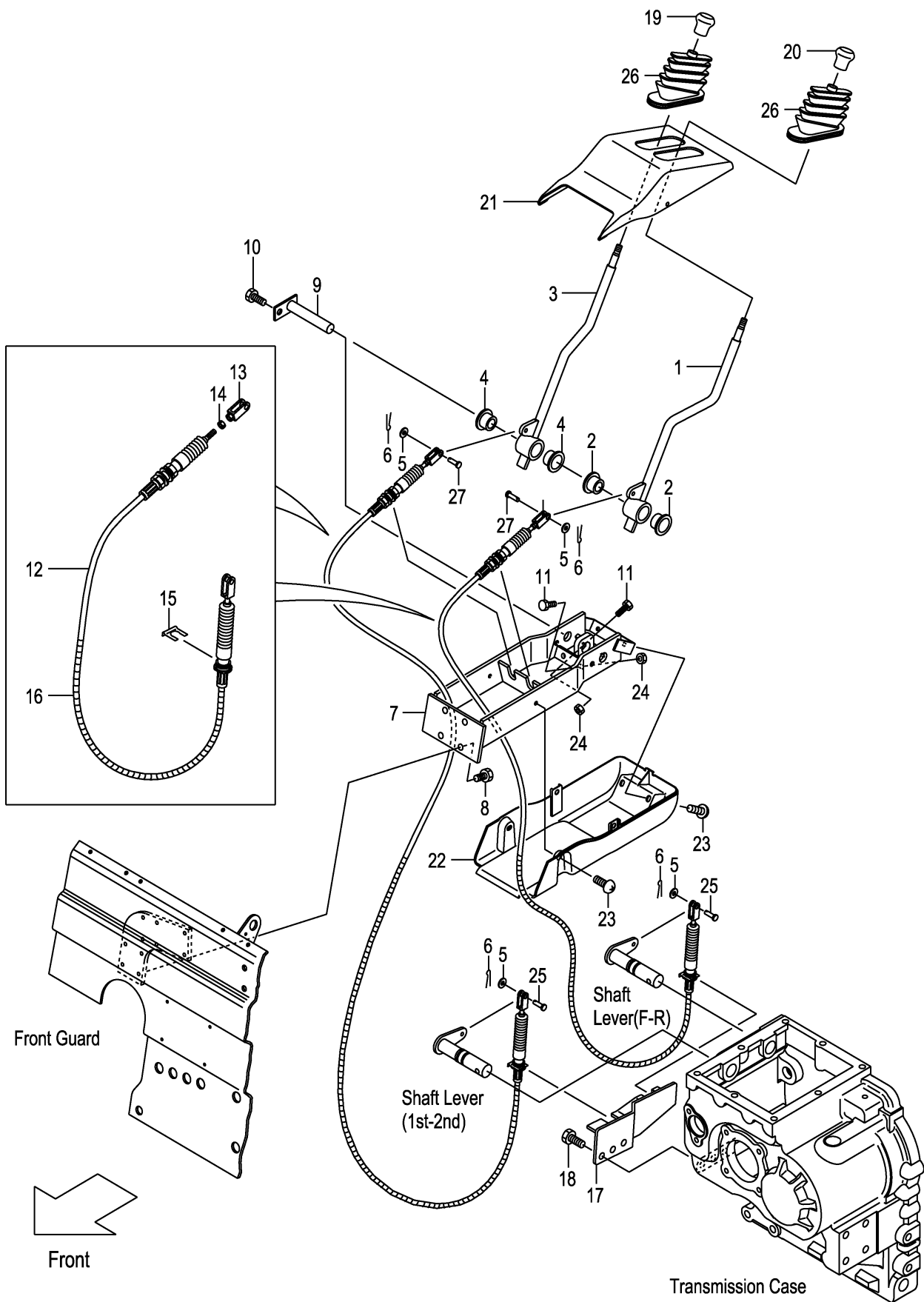
FIG.55 CHANGE LEVER (CLUTCH) (F7Z32540) チェンジレバー
