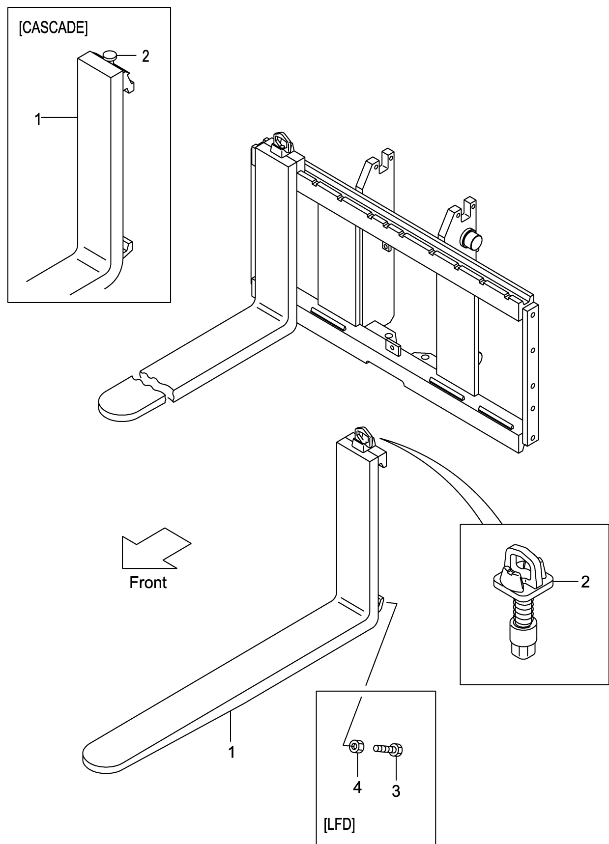
FIG.167 FORK [VFHM2N9] (M7028180) フォーク
