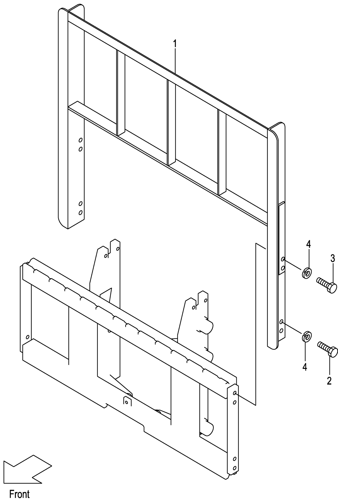
FIG.155 BACKREST [VM2N9] (M7028240) バックレスト
