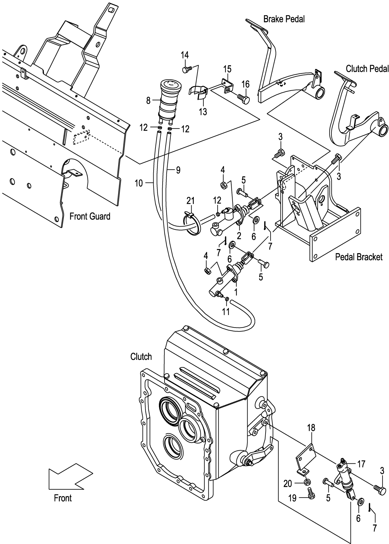
FIG.103 FOOT PEDAL CYLINDER (CLUTCH) (F7Z35440) フットペダルシリンダ
