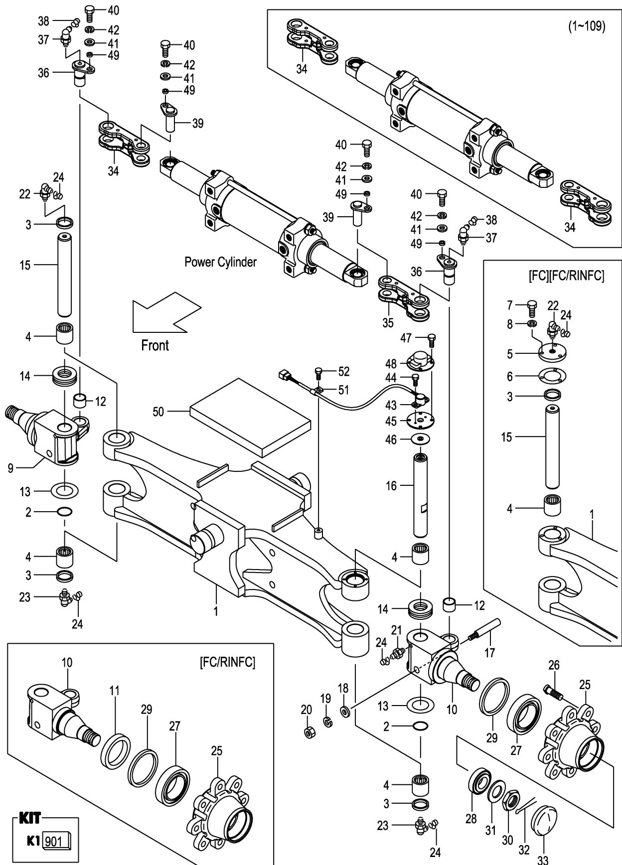
FIG.74 STEERING AXLE (F7Z34310) ステアリングアクスル
