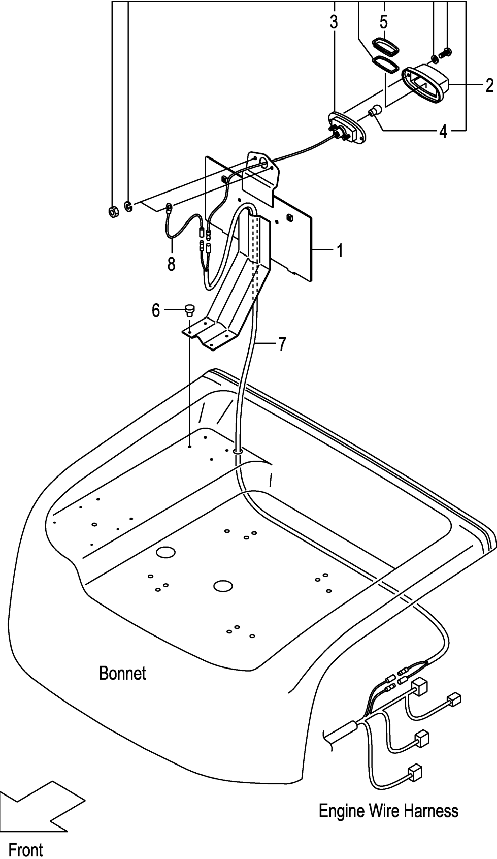
FIG.27 LICENSE LAMP [RRE] (F7Z324K0) ライセンスランプ°
