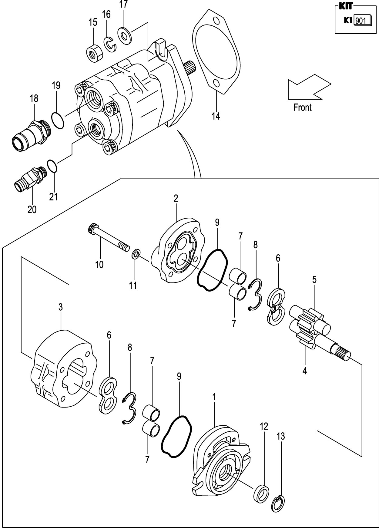
FIG.131 PUMP UNIT (F7Z37110) ポンプユニット
