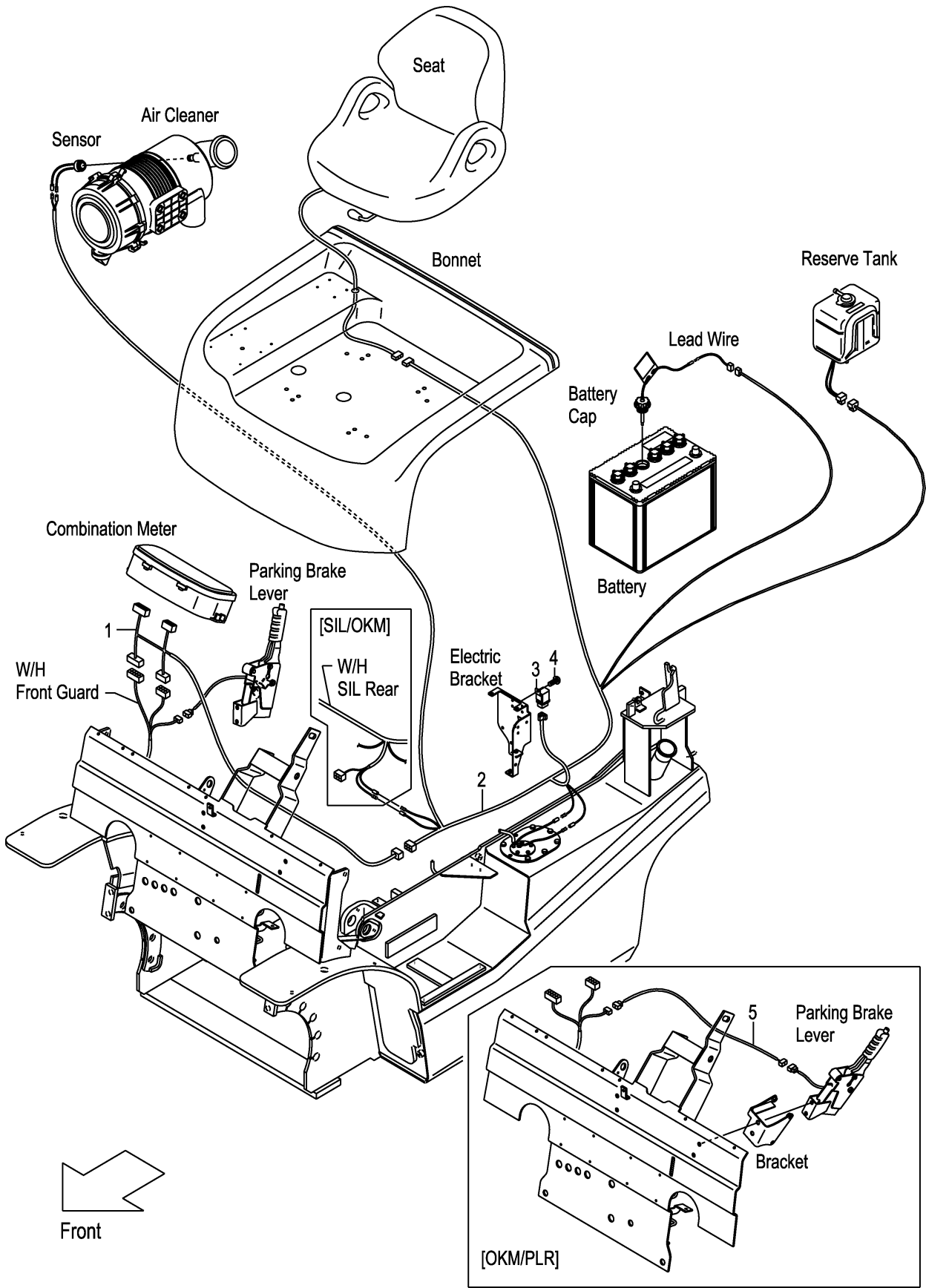
FIG.50 OK MONITOR [OKM] (F7Z326J0) OKモニター
