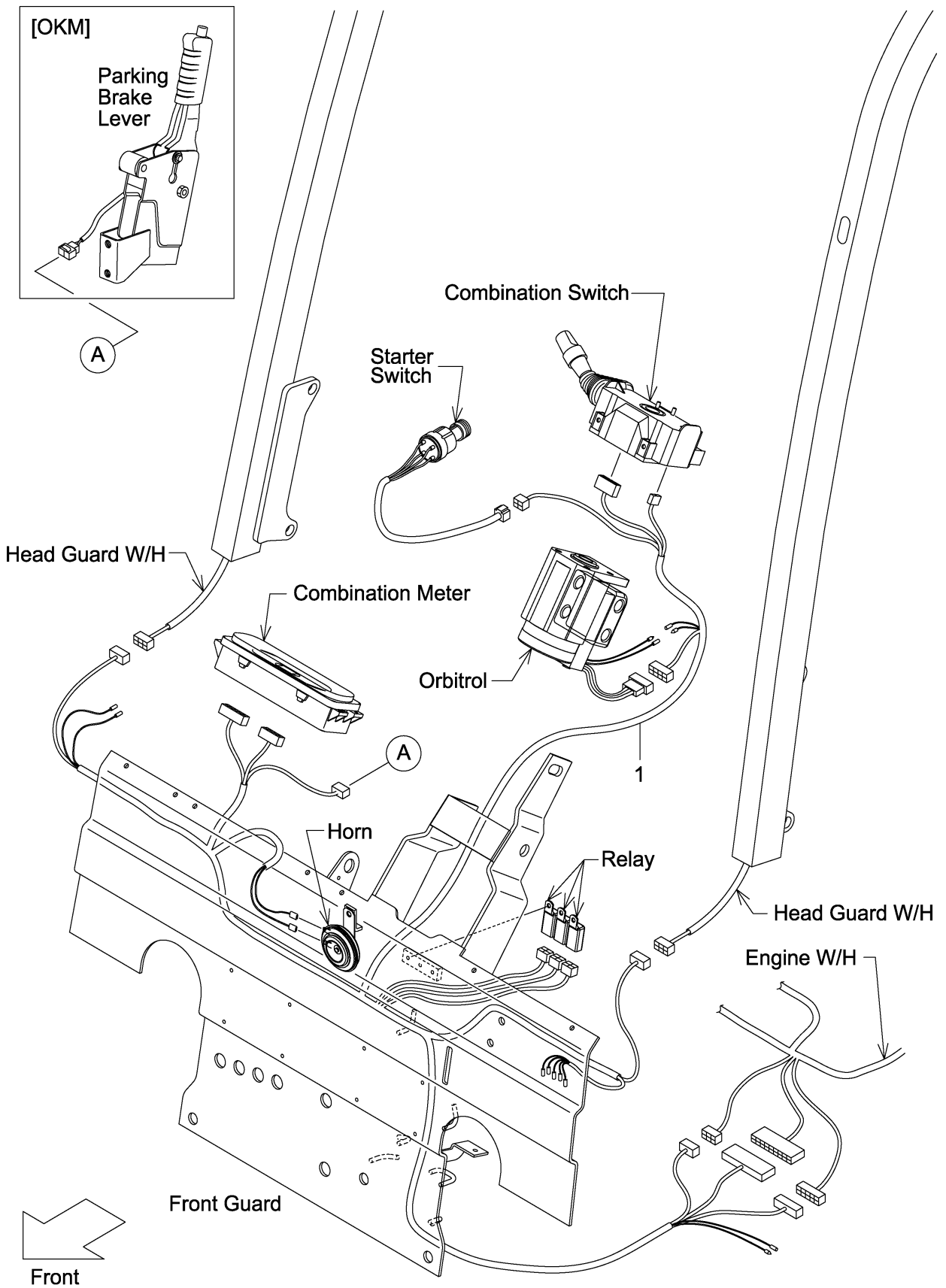
FIG.15 FRONT GUARD WIRE HARNESS (CLUTCH) (F7Z32420) フロントガードワイヤハーネス
