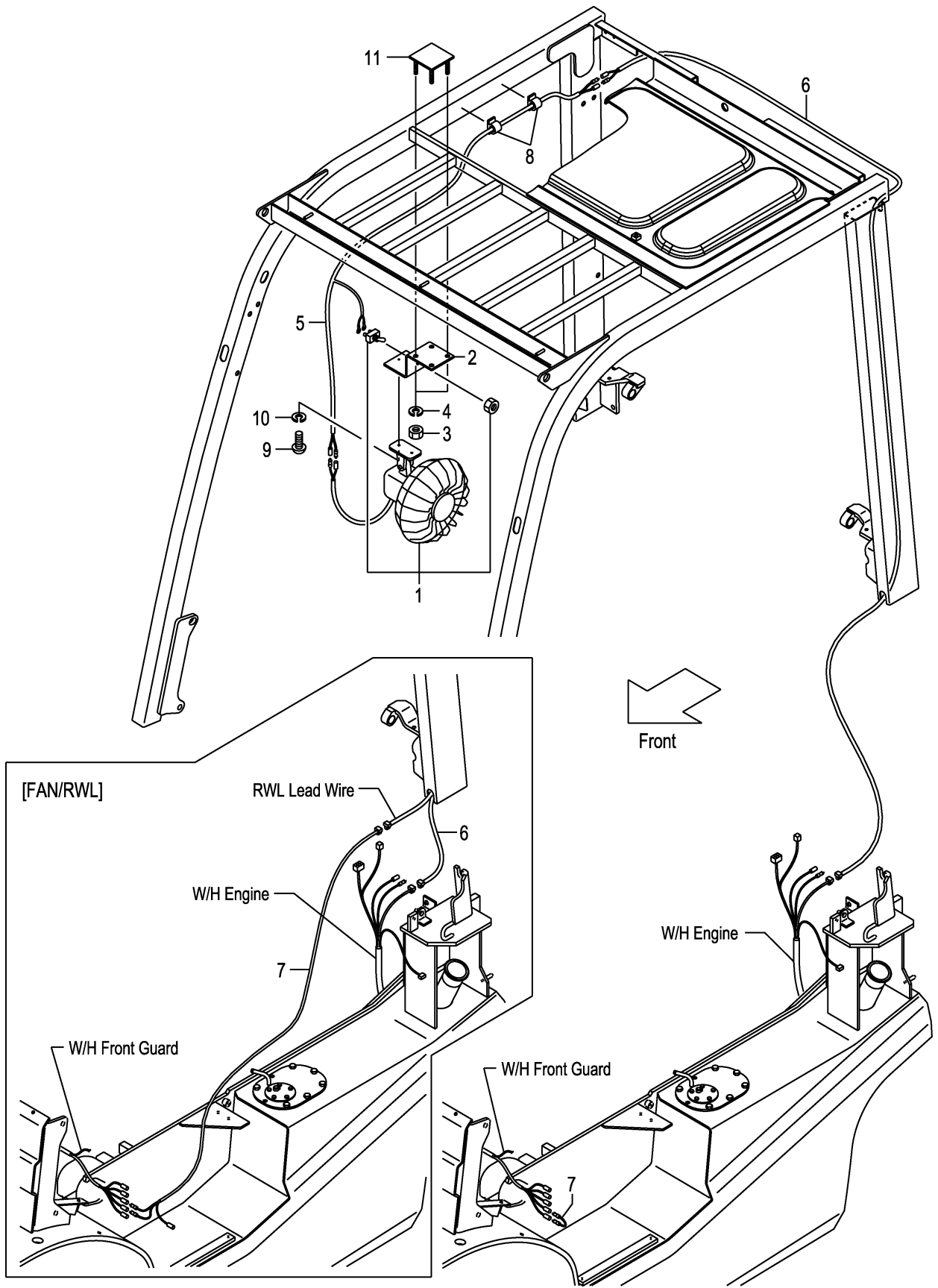
FIG.40 FAN [FAN] (F7Z32650) ファン
