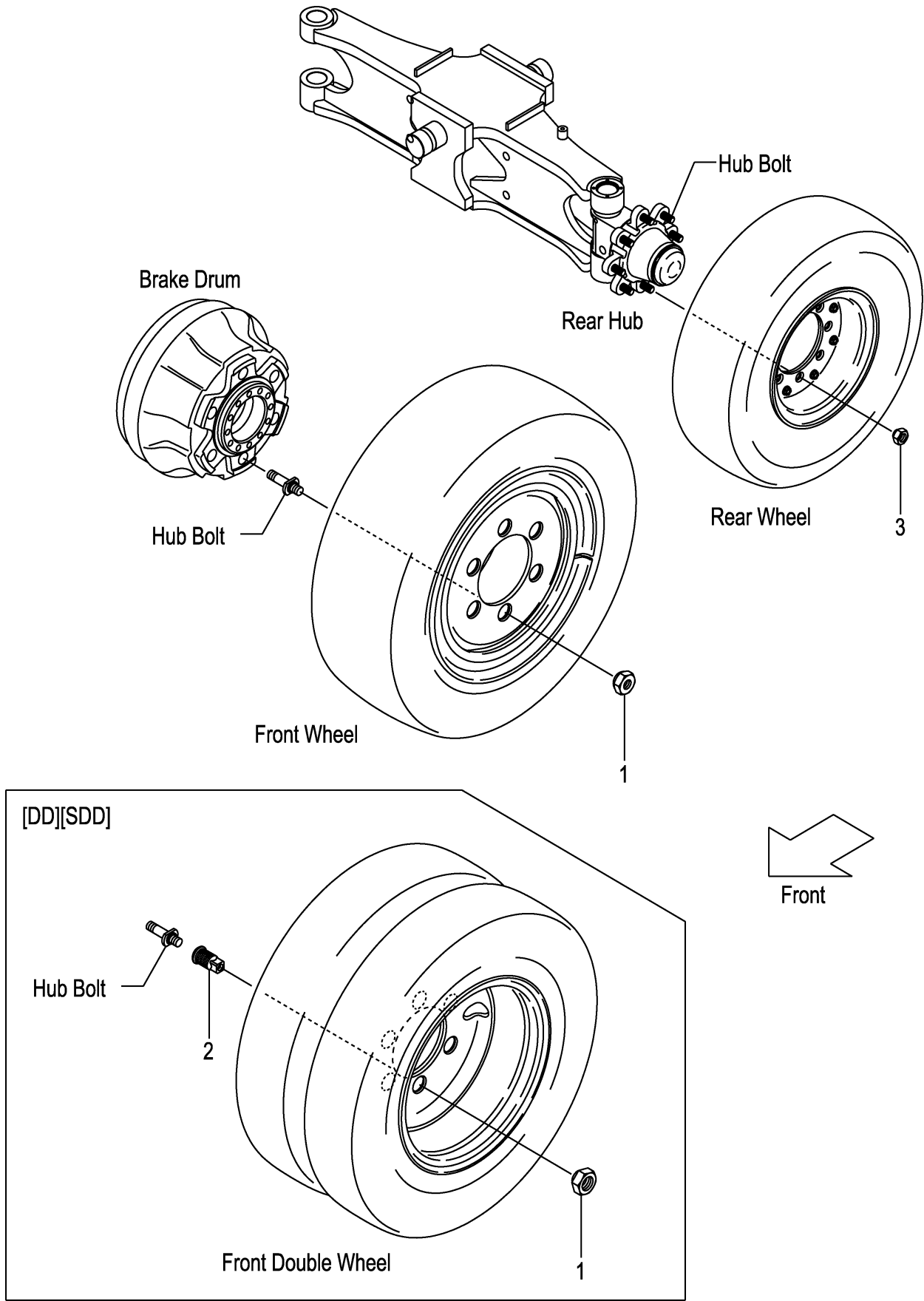
FIG.76 HUB NUT (F7Z34410) ハブナット
