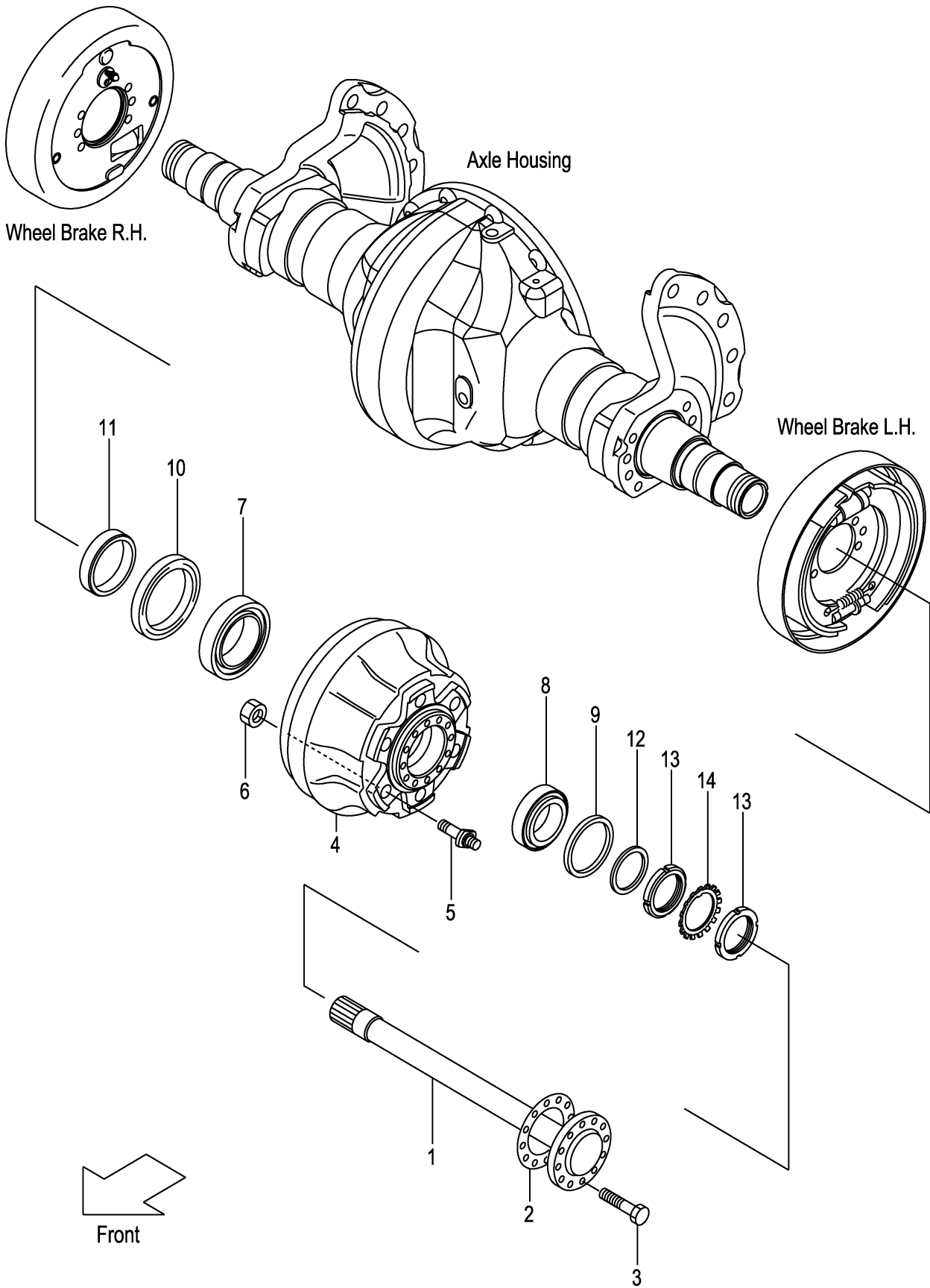
FIG.65 DRUM HUB (F7Z33020) ドラムハブ
