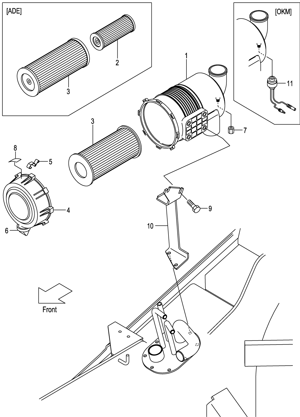
FIG.2 AIR CLEANER (F7Z31040) エアークリーナ
