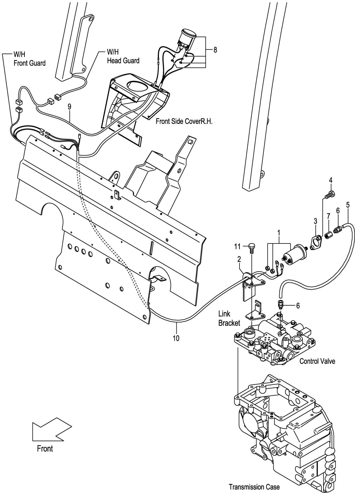
FIG.45 TORQUE CONVERTER PRESSURE METER [TPM] (F7Z326D0) トルクコンバータプレッシャメータ
