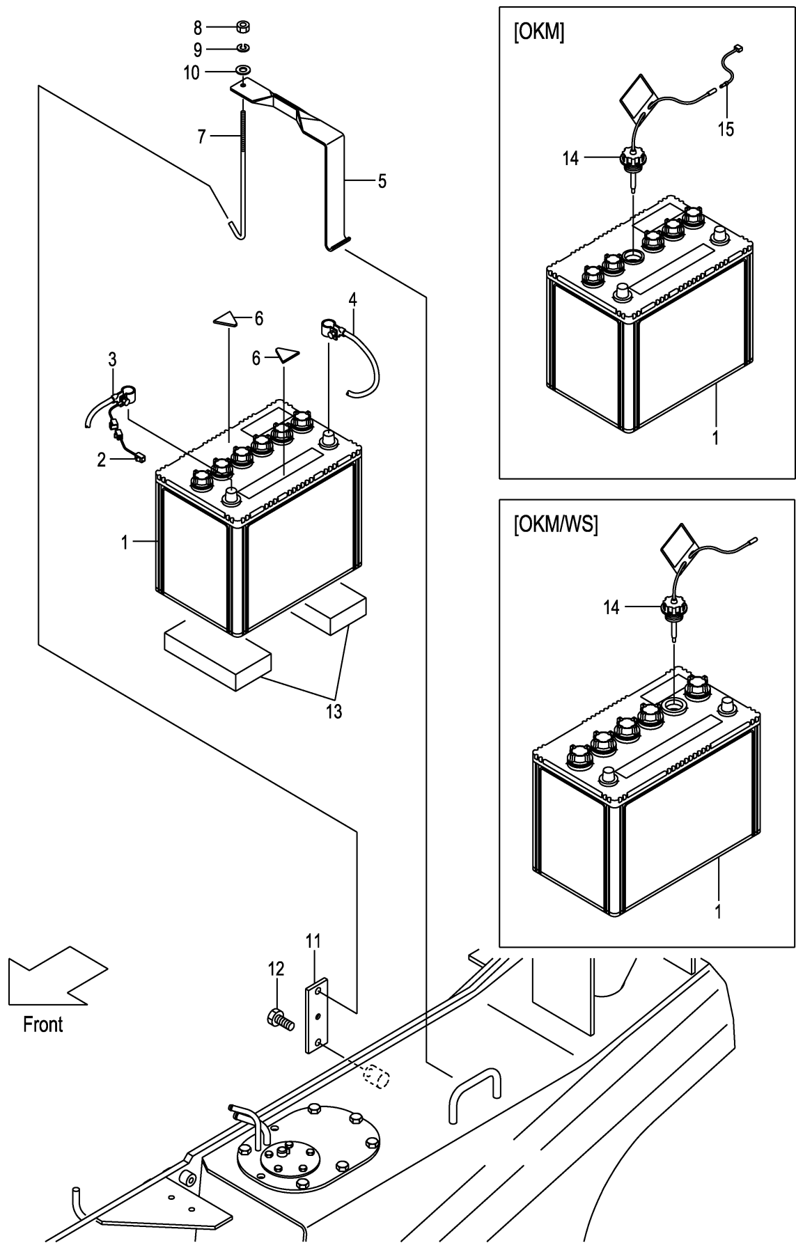
FIG.23 BATTERY (F7Z324F0) バッテリー
