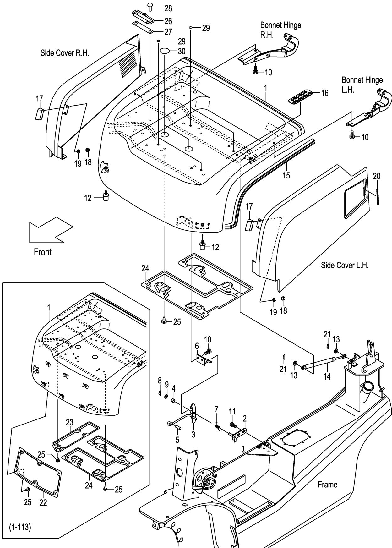
FIG.119 BONNET (F7Z36420) ホンネット
