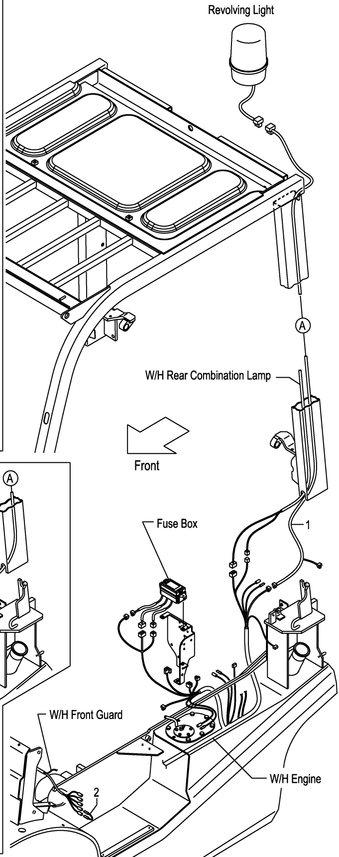
FIG.37 REVOLVING LIGHT WIRE HARNESS [RLY][RLR] (F7Z324W0) リボルビングライトワイヤハーネス
