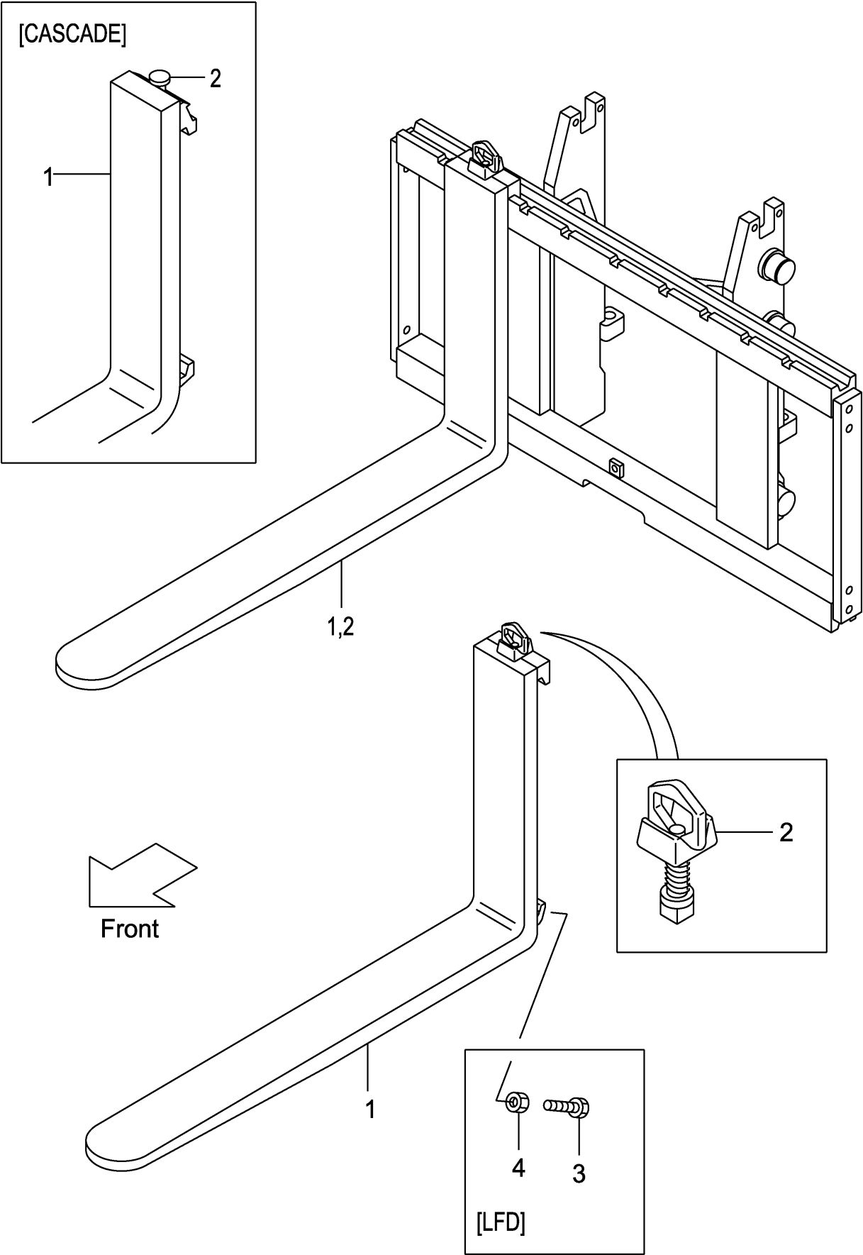
FIG.153 FORK [VM2N9] (M7028120) フォーク
