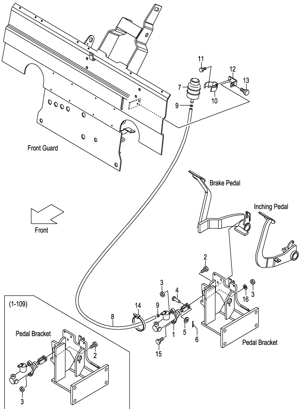
FIG.104 FOOT PEDAL CYLINDER (TOR-CON) (F7Z35450) フットペダルシリンダ
