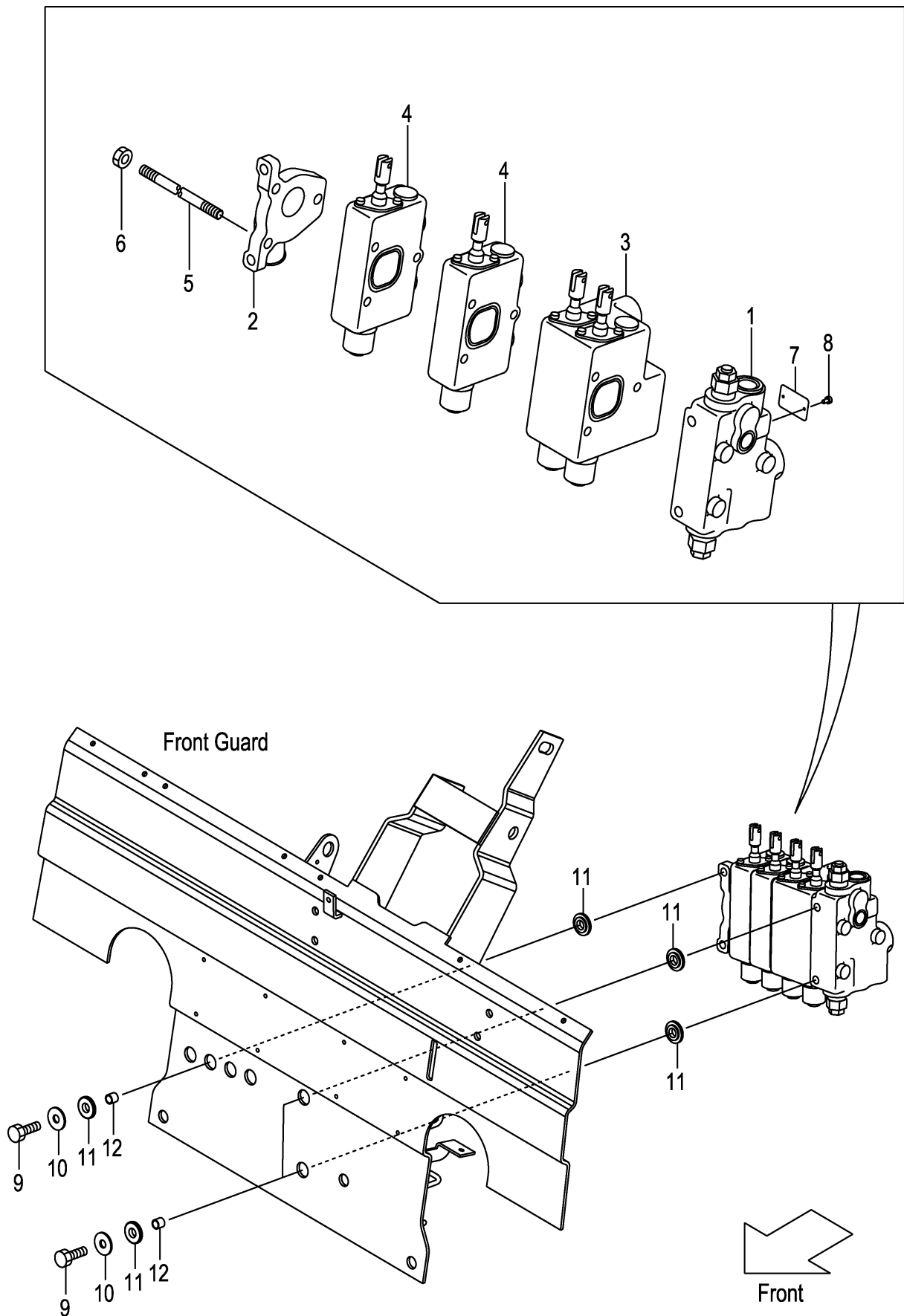
FIG.134 CONTROL VALVE [4SV] (F7Z37330) コントロールバルブ
