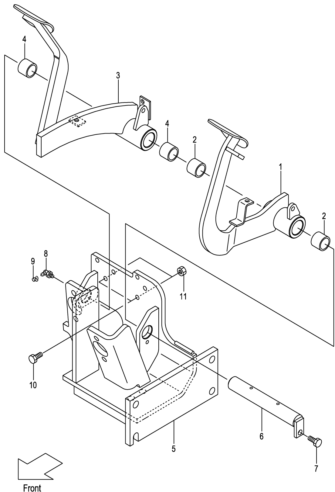
FIG.101 FOOT PEDAL (CLUTCH) (F7Z35410) フットペダル
