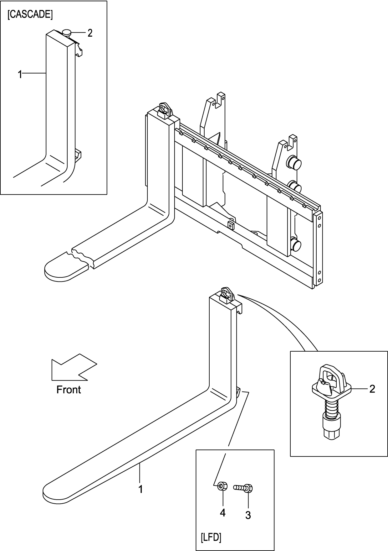
FIG.159 FORK [VFM2N9] (M7028150) フォーク
